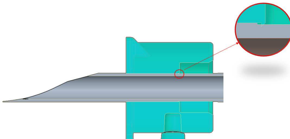
Figura 20: Trava que só permite o movimento para um dos lados da agulha Fonte: dados da pesquisa
