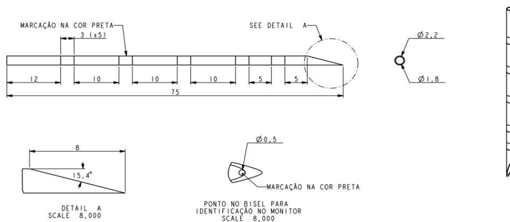
Figura 7: Desenho gráfico da agulha baseline número I.
