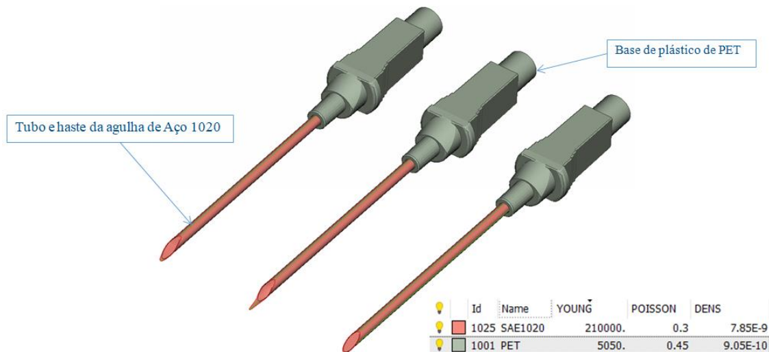
Figura 14: Material adotado para a agulha foi SAE 1020 e para a parte plástica foi o PET (polietileno tereftalato)
