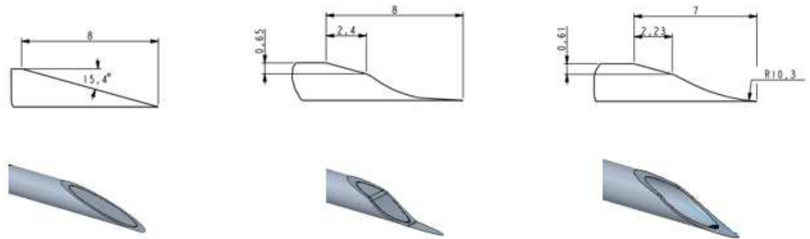
Figura 6: Desenho dos chanfros do bisel do guia metálico do cateter para terapia endovenosa periférica.
