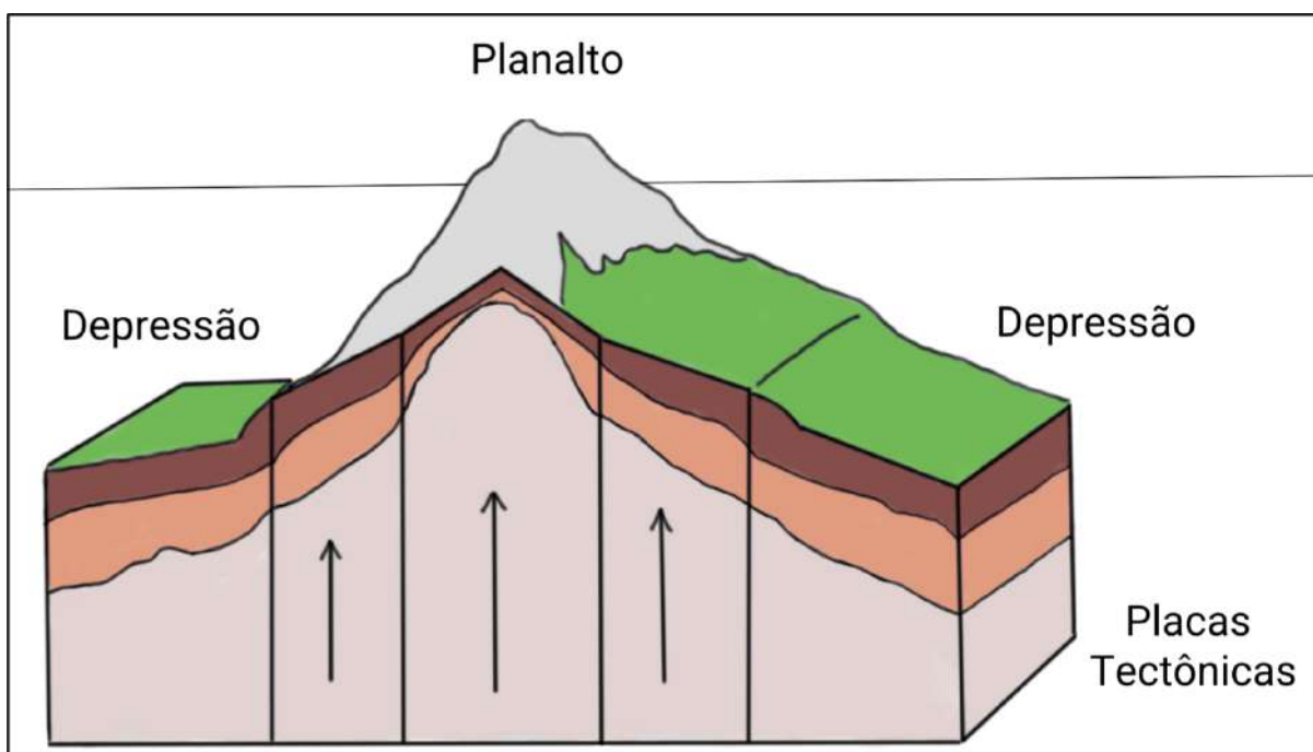
Figura 2: Soerguimento epirogênético
