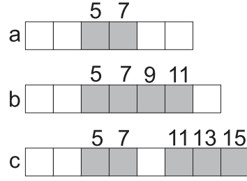
Figura 20 – Exemplos de Ladrilhamentos Inválidos
