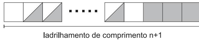
Figura 36 – Possível ladrilhamento de o(n + 1)_{p(n)+2}
