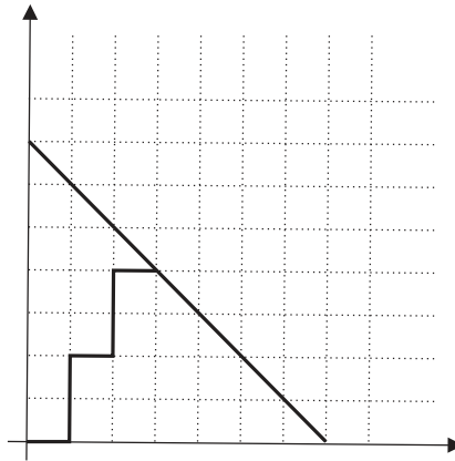
Figura 1 – Procedimento dos Caminhos 01
