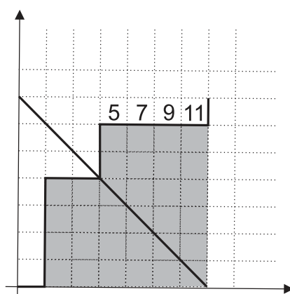
Figura 7 – Procedimento dos Caminhos refletido 02
