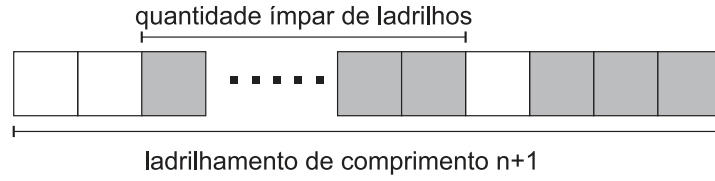
Figura 41 – Ladrilhamento inviável \equiv 3 \pmod{4} - caso ímpar
