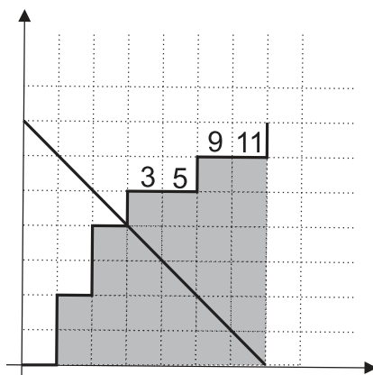
Figura 6 – Procedimento dos Caminhos refletido 01
