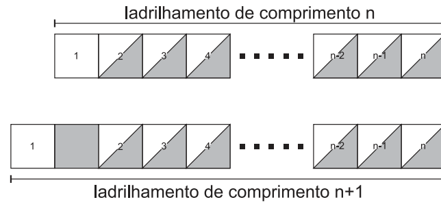
Figura 30 – Aplicação do Teorema 7 em ladrilhamentos
