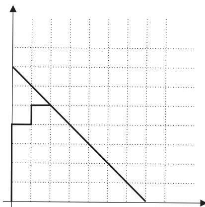
Figura 3 – Procedimento dos Caminhos 03
