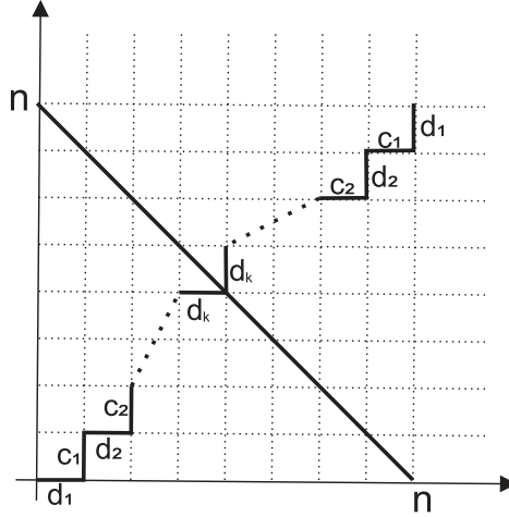
Figura 12 – Conversão direta matriz x ímpares 02
