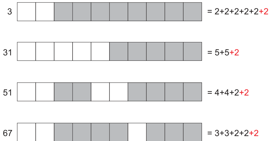
Figura 44 – Termos de referência para n=10
