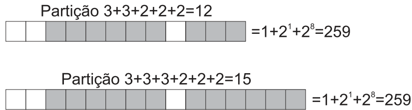
Figura 52 – Ladrilhamentos de mesma interpretação em o(n) (4)
