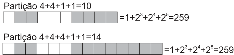
Figura 48 – Ladrilhamentos de mesma interpretação em o(n) (2)
