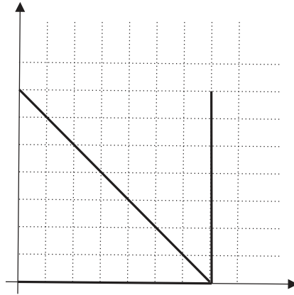
Figura 10 – Procedimento dos Caminhos refletido 05
