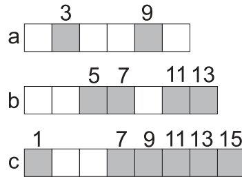
Figura 19 – Exemplos de Ladrilhamentos Inválidos
