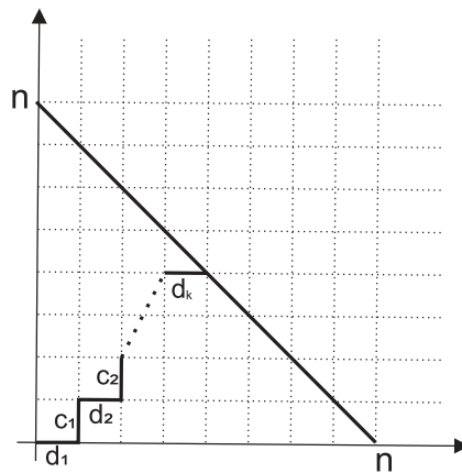
Figura 11 – Conversão direta matriz x ímpares 01
