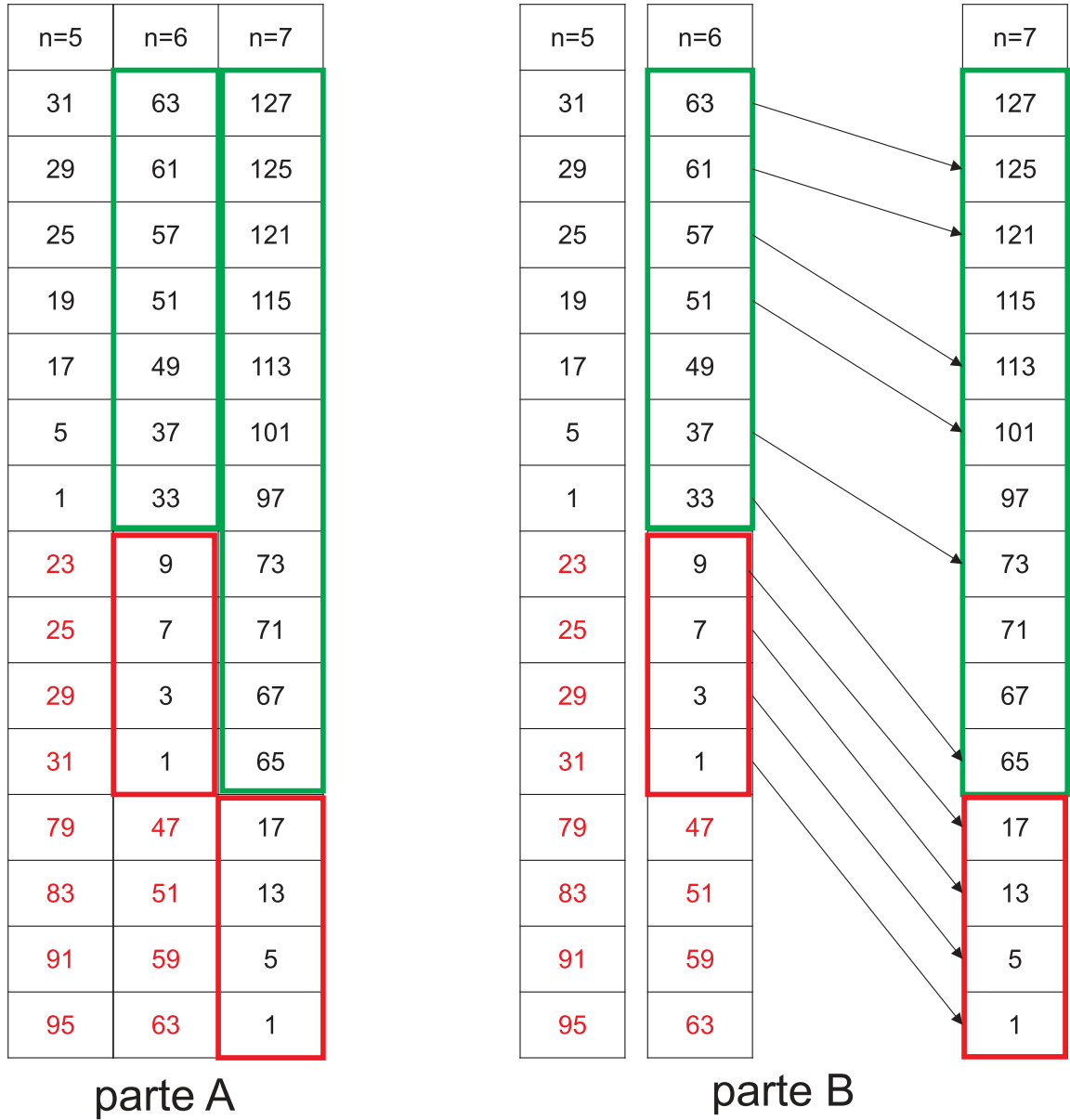
Figura 29 – Relação entre elementos o(5) o(6) o(7) através do Teorema 7
