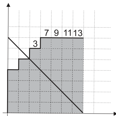
Figura 8 – Procedimento dos Caminhos refletido 03
