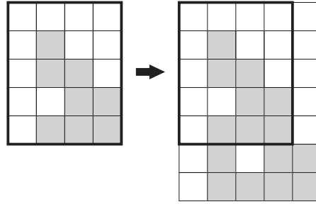
Figura 21 – Comparativo de ladrilhamentos válidos de n=4 e n+1=5 (1)
