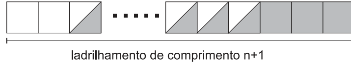
Figura 39 – Formato do maior Ladrilhamento \equiv 3 \pmod{4}
