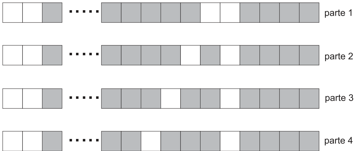
Figura 43 – Ladrilhamento \equiv 3 \pmod{4} - caso ímpar
