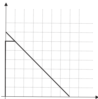
Figura 4 – Procedimento dos Caminhos 04
