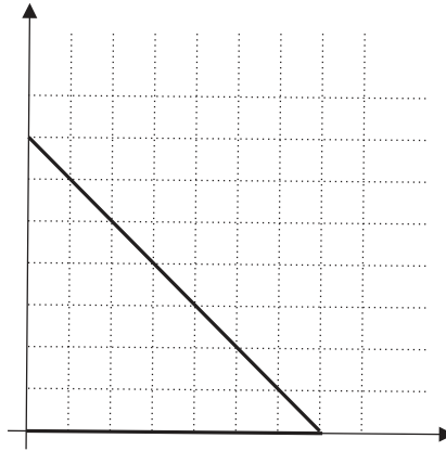
Figura 5 – Procedimento dos Caminhos 05
