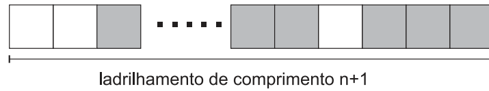
Figura 40 – Maior Ladrilhamento \equiv 3 \pmod{4} - caso par
