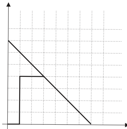
Figura 2 – Procedimento dos Caminhos 02
