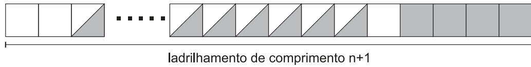
Figura 42 – Candidato - Ladrilhamento \equiv 3 \pmod{4} - caso ímpar
