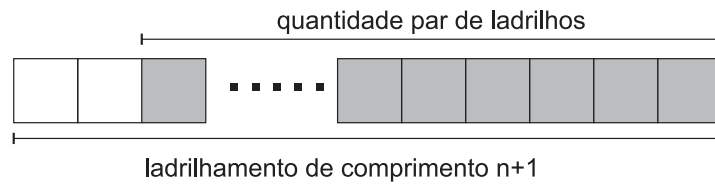
Figura 38 – Menor Ladrilhamento \equiv 3 \pmod{4} - caso par
