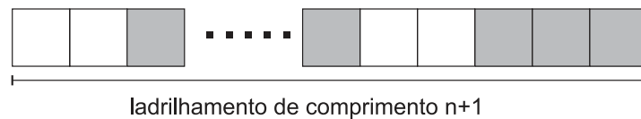
Figura 37 – Ladrilhamento de o(n + 1)_{p(n)+2}
