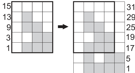
Figura 22 – Comparativo de ladrilhamentos válidos de n=4 e n+1=5 (2)
