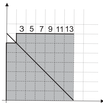
Figura 9 – Procedimento dos Caminhos refletido 04
