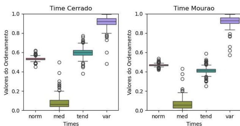
Figura 10- Gráficos Boxplot das dos valores globais das equipes 13ª e 14ª colocadas na classificação, atribuindo peso iguais para os critérios temporais (norm), atribuindo peso 1 para média (med), atribuindo peso 1 para tendência (tend) e atribuindo peso 1 para coeficiente de variação (var).
