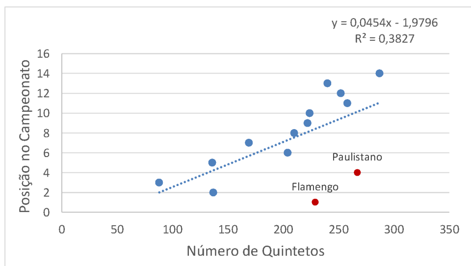
Figura 5 - Dispersão do número de quintetos pela classificação dos times no NBB.
