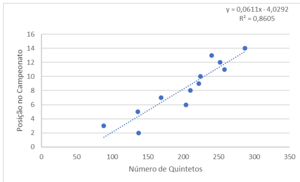
Figura 6 - Dispersão do número de quintetos pela classificação dos times no NBB, excluindo Flamengo e Paulistano.
