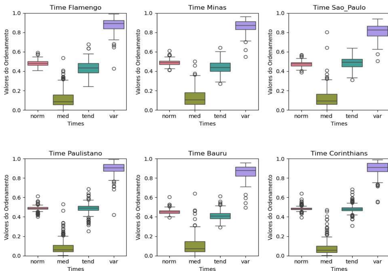
Figura 8 - Gráficos Boxplot das dos valores globais das equipes da 1º à 6º colocação na classificação, atribuindo peso iguais para os critérios temporais (norm), atribuindo peso 1 para média (med), atribuindo peso 1 para tendência (tend) e atribuindo peso 1 para coeficiente de variação (var).
