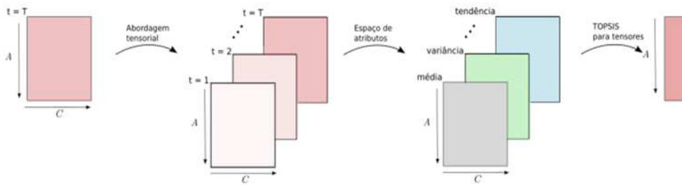
Figura 4- Figura representativa da metodologia proposta por (CAMPELO et al. 2023).
