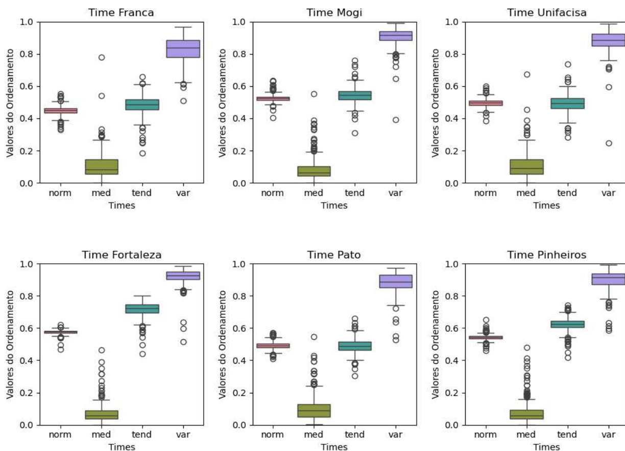
Figura 9- Gráficos Boxplot das dos valores globais das equipes da 7ª à 12ª colocação na classificação, atribuindo peso iguais para os critérios temporais (norm), atribuindo peso 1 para média (med), atribuindo peso 1 para tendência (tend) e atribuindo peso 1 para coeficiente de variação (var).
