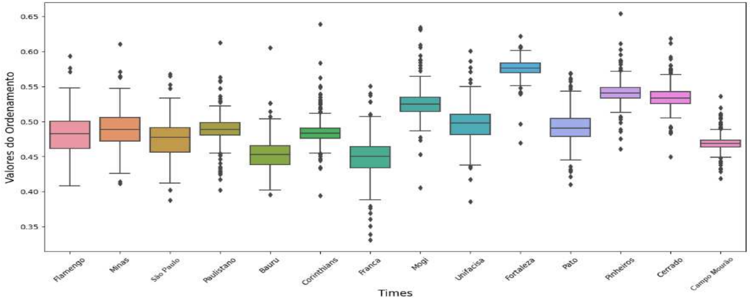
Figura 7 - Gráficos Boxplot da dos valores globais dos quintetos (obtidos por MCDA) de cada equipe.
