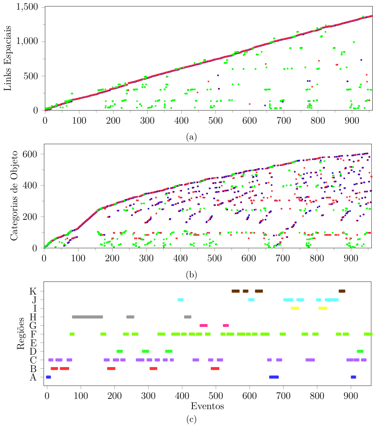
Figura 7.18 – Relação entre nós de eventos e as informações dos links espaciais conectados a eles.(a) Links espaciais conectados aos eventos na memória episódica; (b) Categorias de objetos referidos pelos links espaciais do evento; (c) Região ocupada pelo agente durante o evento. (a,b) Verdes indicam uma conexão do tipo contexto espacial. Azuis indicam uma conexão do tipo início de evento. Vermelhos indicam uma conexão do tipo final de evento. (c) Cada cor e letra de região refere-se as segmentações adotadas na Figura 6.3.
