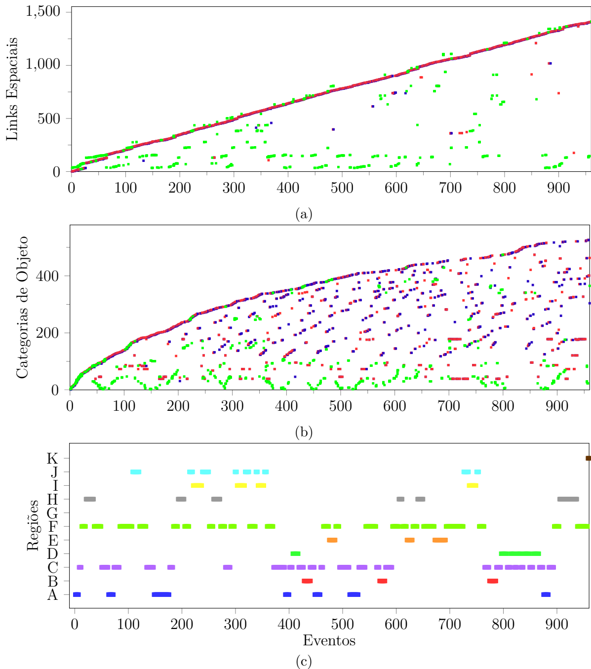
Figura 7.19 – Relação entre nós de eventos e as informações dos links espaciais conectados a eles. (a) Links espaciais conectados aos eventos na memória episódica; (b) Categorias de objetos referidos pelos links espaciais do evento; (c) Região ocupada pelo agente durante o evento. (a,b) Verdes indicam uma conexão do tipo contexto espacial. Azuis indicam uma conexão do tipo início de evento. Vermelhos indicam uma conexão do tipo final de evento. (c) Cada cor e letra de região refere-se as segmentações adotadas na Figura 6.3.
