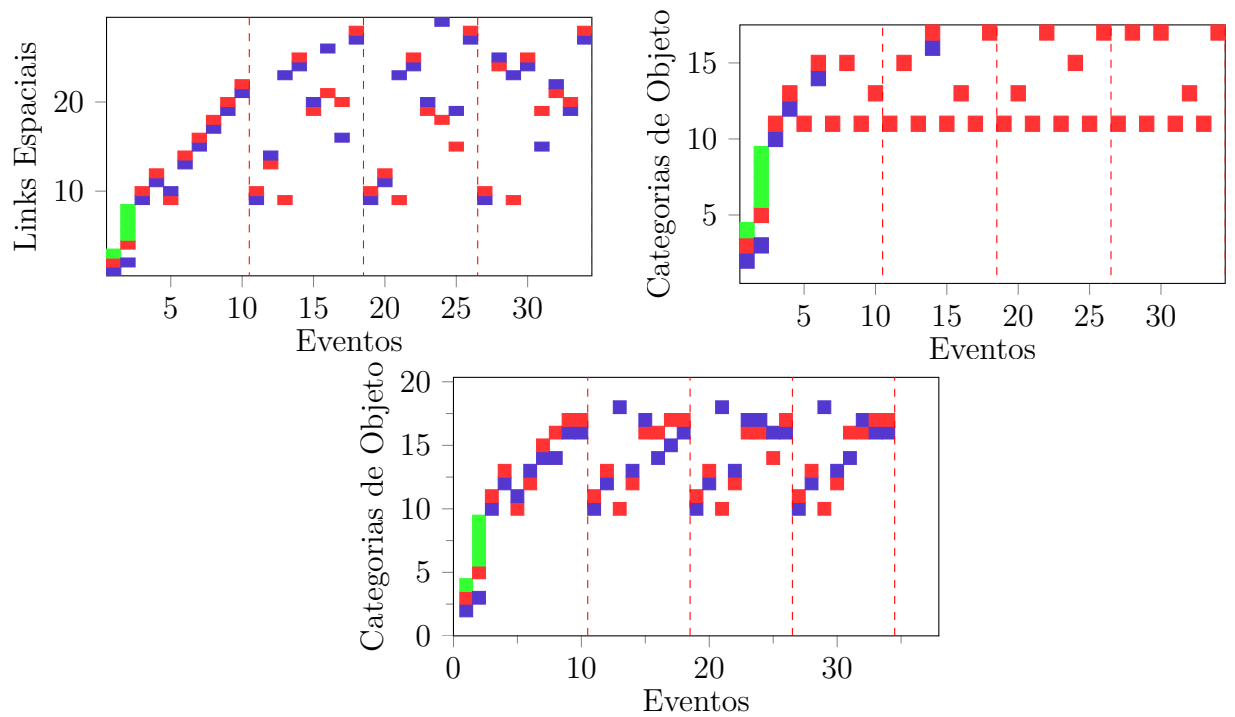
Figura 7.12 – Relações entre eventos e as informações dos links espaciais conectados para execução com limiar de evento 0.01 e objeto 0.2.
