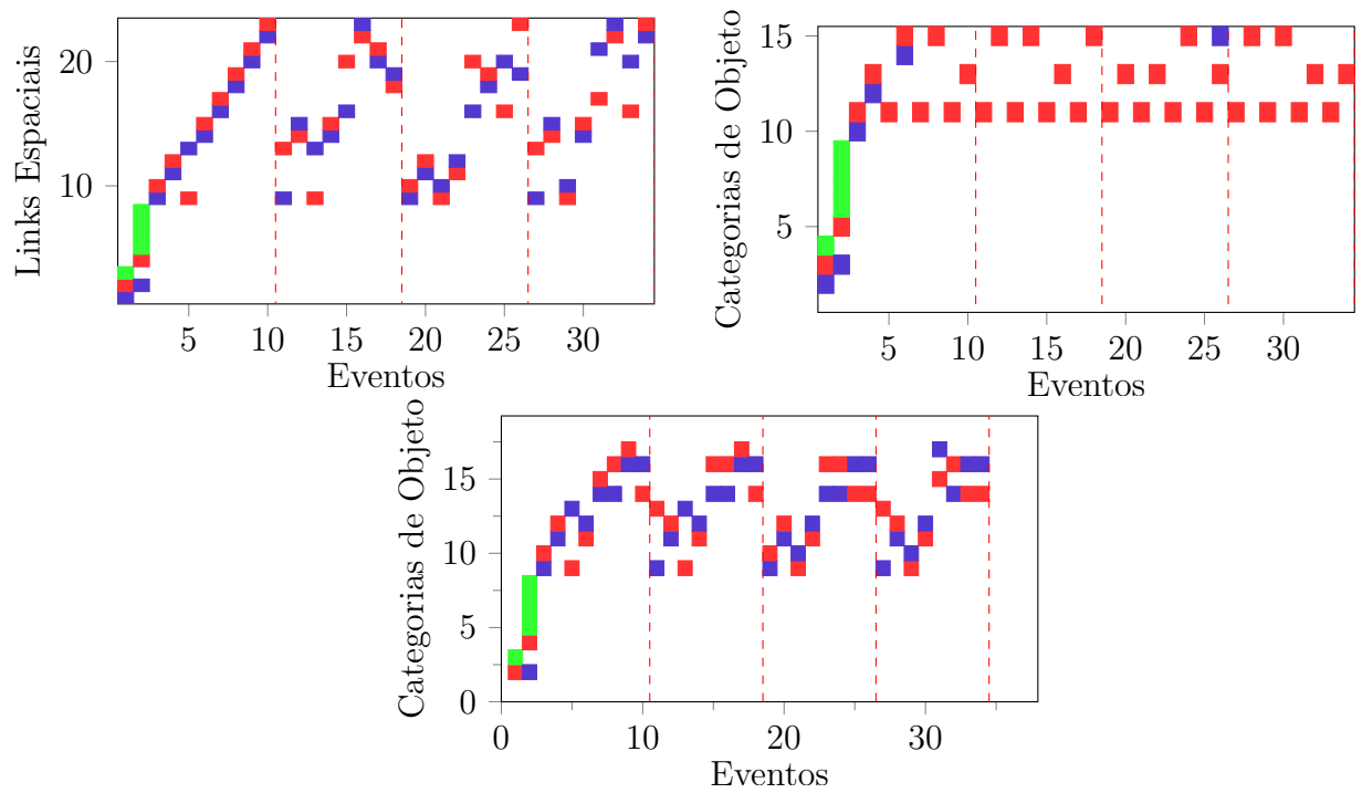
Figura 7.13 – Relações entre eventos e as informações dos links espaciais conectados para execução com limiar de evento 0.01 e objeto 0.1.
