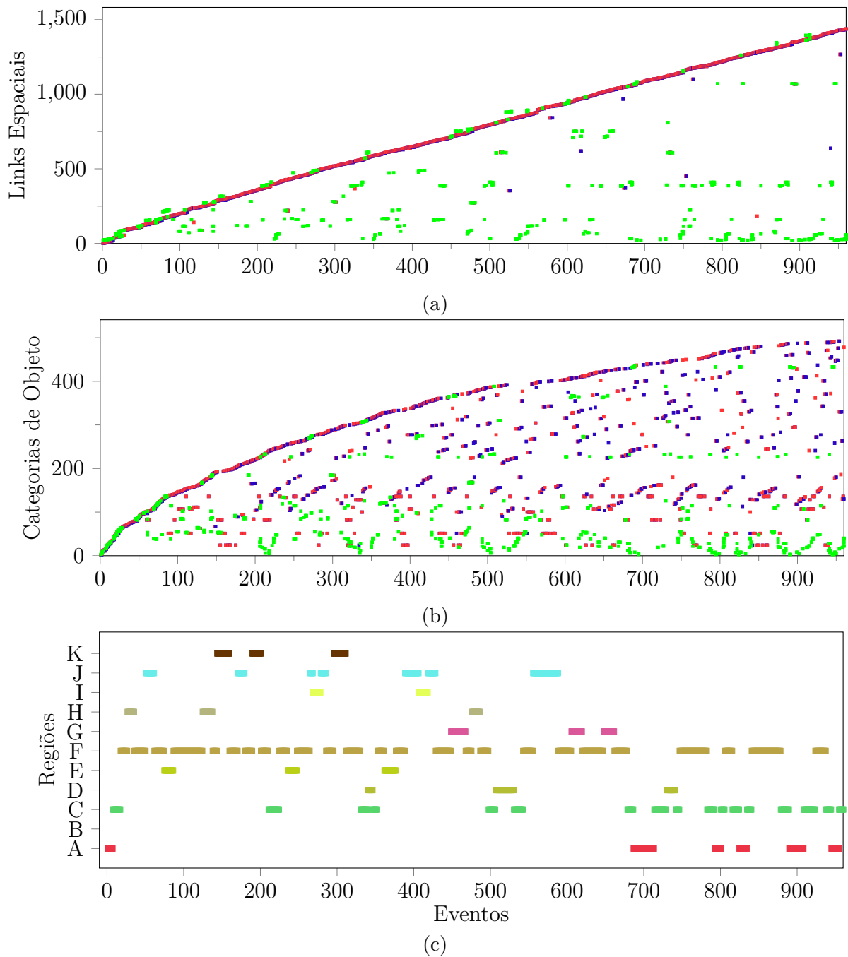
Figura 7.17 – Relação entre nós de eventos e as informações dos links espaciais conectados a eles. (a) Links espaciais conectados aos eventos na memória episódica; (b) Categorias de objetos referidos pelos links espaciais do evento; (c) Região ocupada pelo agente durante o evento. (a,b) Verdes indicam uma conexão do tipo contexto espacial. Azuis indicam uma conexão do tipo início de evento. Vermelhos indicam uma conexão do tipo final de evento. (c) Cada cor e letra de região refere-se as segmentações adotadas na Figura 6.3.
