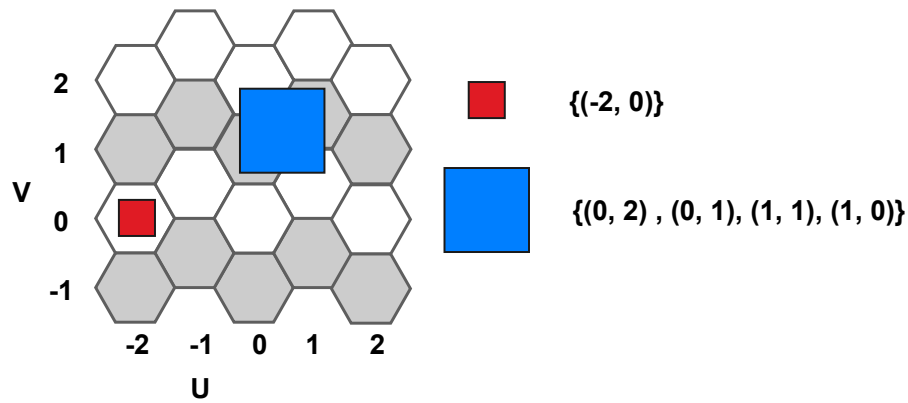
Figura 5.4 – Representação matricial da grade hexagonal. De forma alternada, é destacado em cinza as células pertencentes a uma mesma linha. Adicionalmente é exibido como pode-se obter o conjunto de células ocupadas por objetos do ambiente. O objeto vermelho ocupa somente a célula (-2, 0) , enquanto do objeto azul ocupa as células (0, 2) , (0, 1) , (1, 1) e (1, 0)
