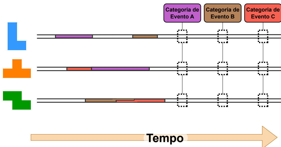
Figura 5.10 – Ilustração do funcionamento dos codelets de detecção de evento.
