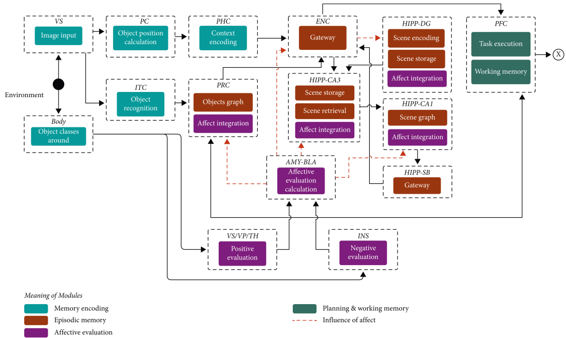
Figura 2.5 – Sistema episódico da arquitetura Cuâyôllôtl - extraído de Martin et al. (2021)
