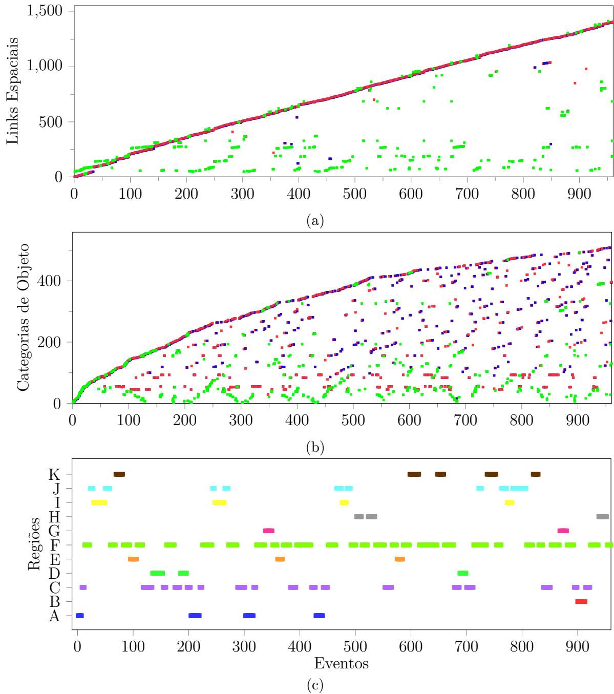
Figura 7.16 – Relação entre nós de eventos e as informações dos links espaciais conectados a eles. (a) Links espaciais conectados aos eventos na memória episódica; (b) Categorias de objetos referidos pelos links espaciais do evento; (c) Região ocupada pelo agente durante o evento. (a,b) Verdes indicam uma conexão do tipo contexto espacial. Azuis indicam uma conexão do tipo início de evento. Vermelhos indicam uma conexão do tipo final de evento. (c) Cada cor e letra de região refere-se as segmentações adotadas na Figura 6.3.
