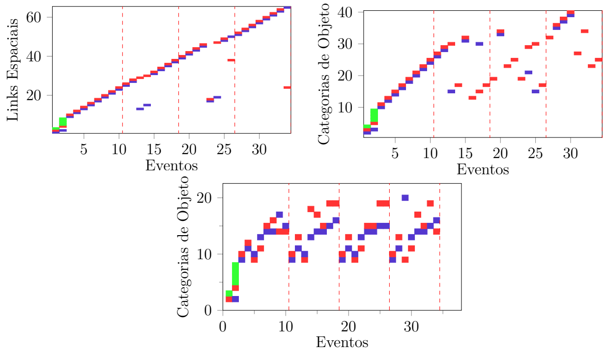
Figura 7.4 – Relações entre eventos e as informações dos links espaciais conectados para execução com limiar de evento 0.01 e objeto 0.95.
