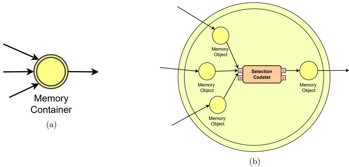
Figura 3.2 – Elemento Memory Container . (a) Representação de um memory container conforme padrão esquemático do CST; (b) Representação do funcionamento interno de um memory container - adaptado de Gudwin et al. (2017) .
