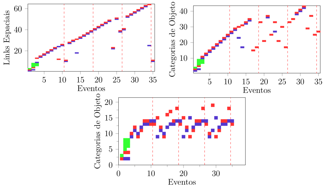
Figura 7.5 – Relações entre eventos e as informações dos links espaciais conectados para execução com limiar de evento 0.01 e objeto 0.9.
