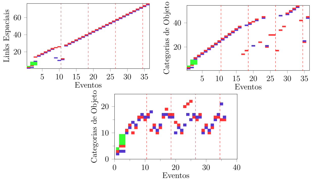
Figura 7.3 – Relações entre eventos e as informações dos links espaciais conectados para execução com limiar de evento 0.01 e objeto 0.99.
