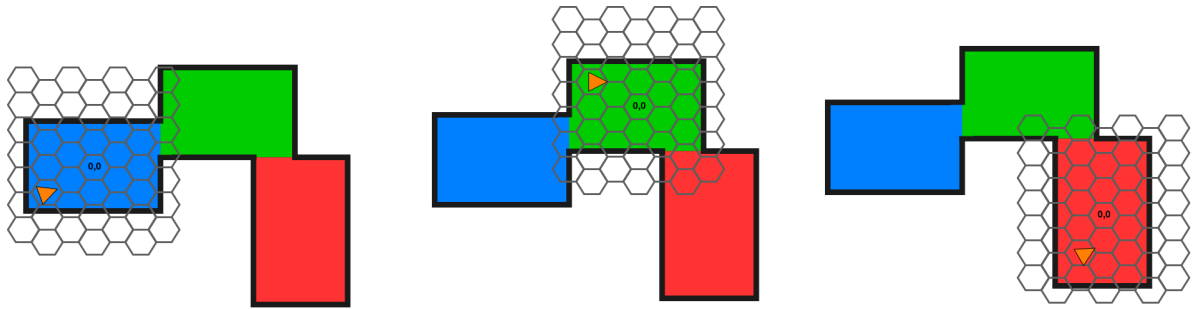
Figura 5.5 – Exemplo de offset da grade hexagonal por região. Cada retângulo representa uma região conhecida pelo agente (triângulo laranja). Quando posicionado no ambiente azul, a grade hexagonal é centrada no mesmo. Conforme o agente se locomove pelo ambiente a grade para representação da posição dos objetos percebidos é deslocada de forma a alinhar seu centro como o centro do ambiente.
