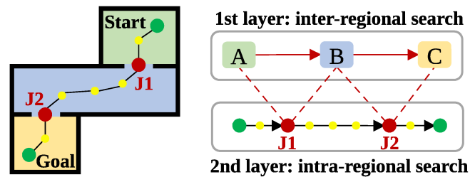
Figura 5.6 – Ilustração do método de planejamento de rotas hierárquico - extraído de Ryu (2020).
