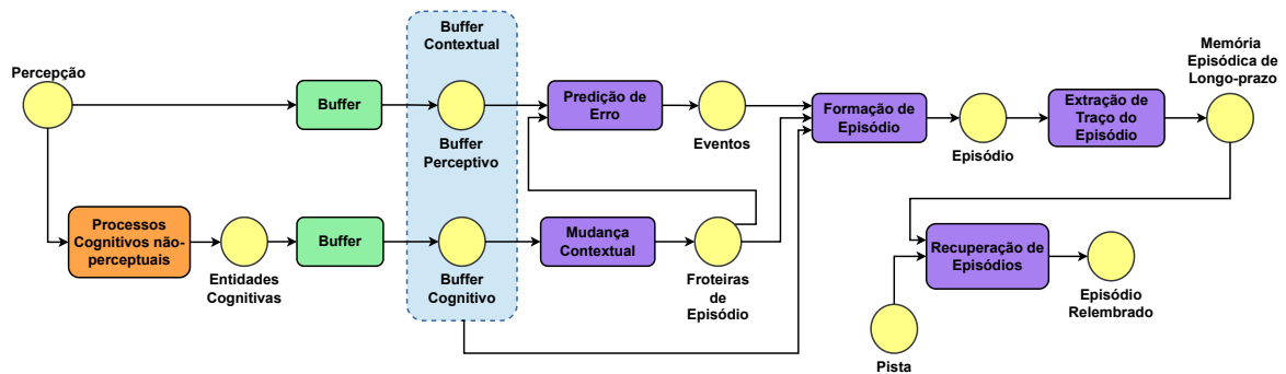
Figura 4.1 – Modelo conceitual para sistema de memória episódica proposto. Retângulos com cantos arredondados são codelets com setas indicando a direção do fluxo de informações; Círculos são memory objects ; Retângulo azul com bordas tracejadas são grupos de memórias utilizado como uma ferramenta de organização para agregar memory objects .
