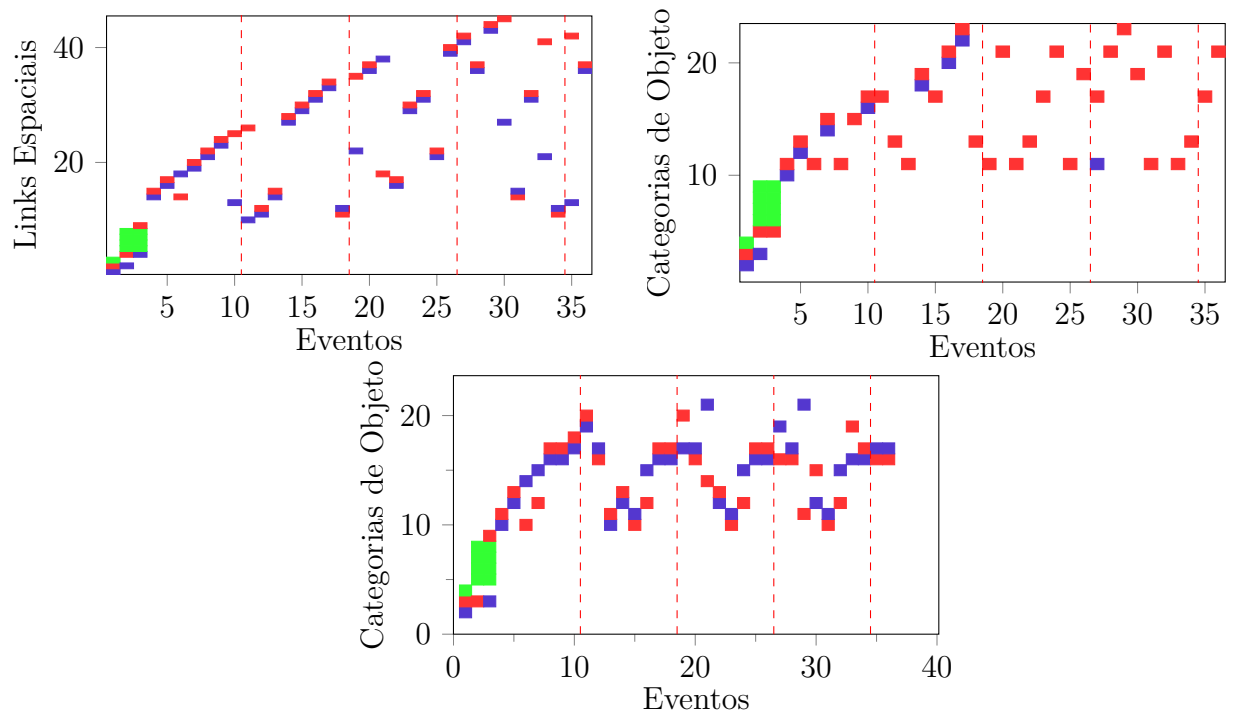
Figura 7.9 – Relações entre eventos e as informações dos links espaciais conectados para execução com limiar de evento 0.01 e objeto 0.5.
