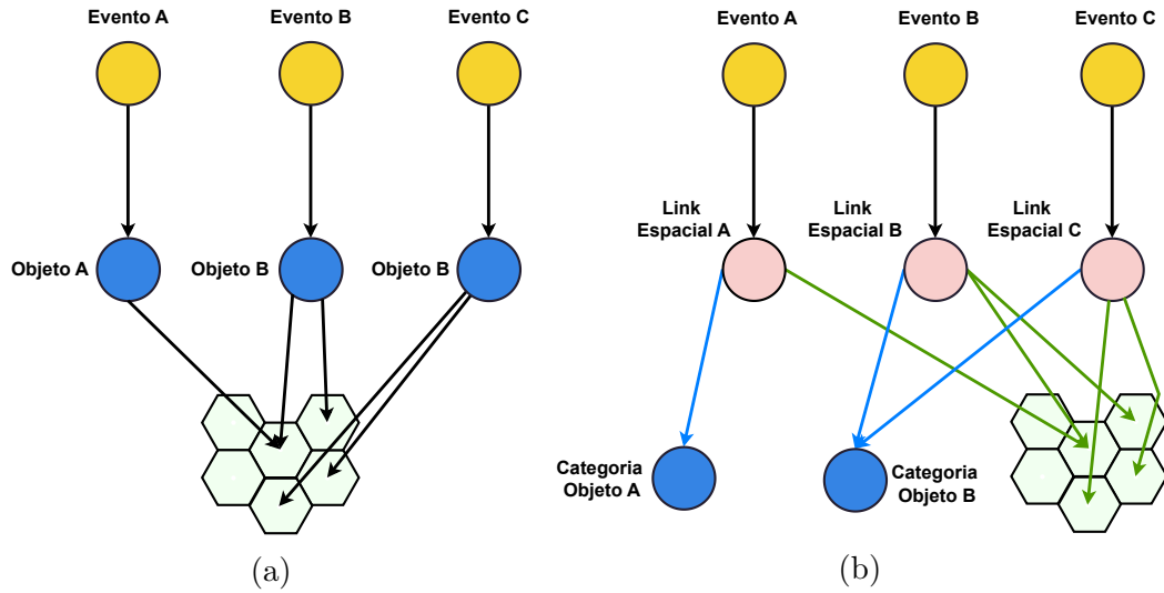
Figura 5.12 – Transformação de um episódio experienciado em um episódio armazenado. Círculos amarelos são Ideas de evento, azuis de objetos, rosas de link e hexagonos são Ideas de posição. (a) Representação em grafo de um episódio experienciado, i.e., a saída fornecida pelo codelet de formação de episódio; (b) Representação em grafo de um episódio armazenado com links espaciais.
