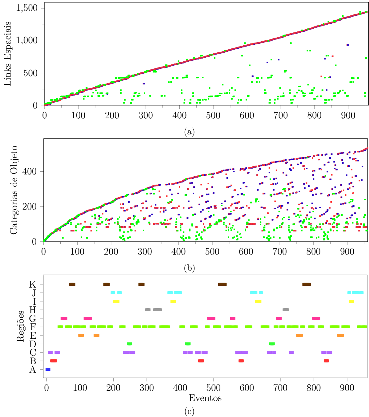
Figura 6.4 – Relação entre nós de eventos e as informações dos links espaciais conectados a eles. (a) Links espaciais conectados aos eventos na memória episódica; (b) Categorias de objetos referidos pelos links espaciais do evento; (c) Região ocupada pelo agente durante o evento. (a,b) Pontos verdes indicam uma conexão do tipo contexto espacial. Pontos azuis indicam uma conexão do tipo início ou fim de evento. Linhas tracejadas vermelhas indicam os instantes de segmentação de episódios. (c) Cada cor e letra de região refere-se as segmentações adotadas na Figura 6.3.
