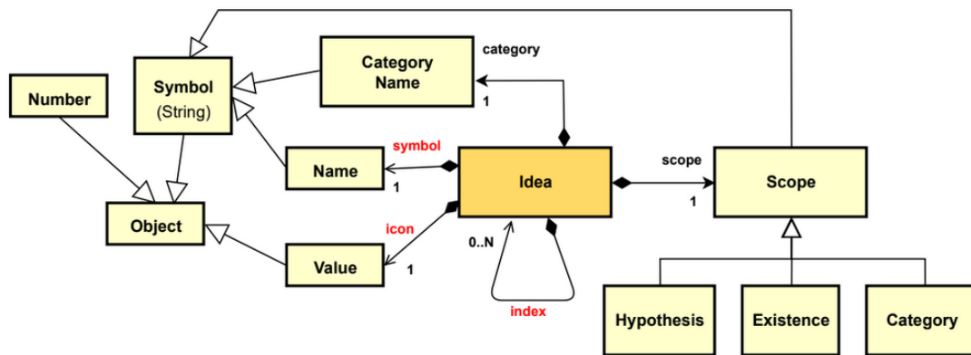
Figura 3.5 – Diagrama da estrutura computacional de uma Idea - extraído de Camargo et al. (2022) .
