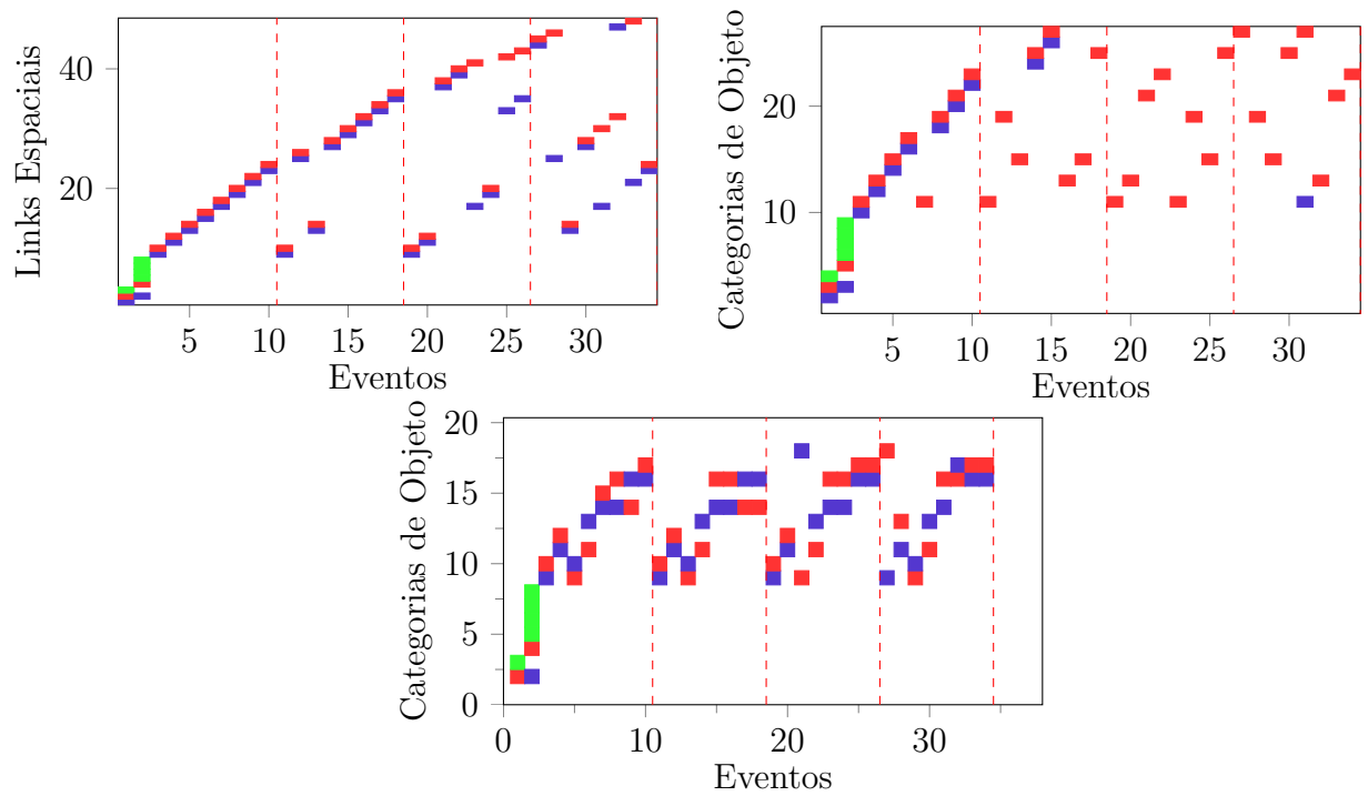
Figura 7.7 – Relações entre eventos e as informações dos links espaciais conectados para execução com limiar de evento 0.01 e objeto 0.7.
