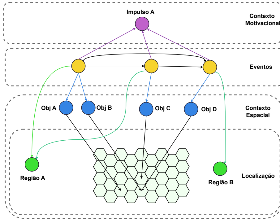
Figura 5.8 – Exemplo de representação de um episódio. Cada círculo e hexágono corresponde a uma Idea que contém informação sobre um objeto, evento, região, motivação, ou posição.
