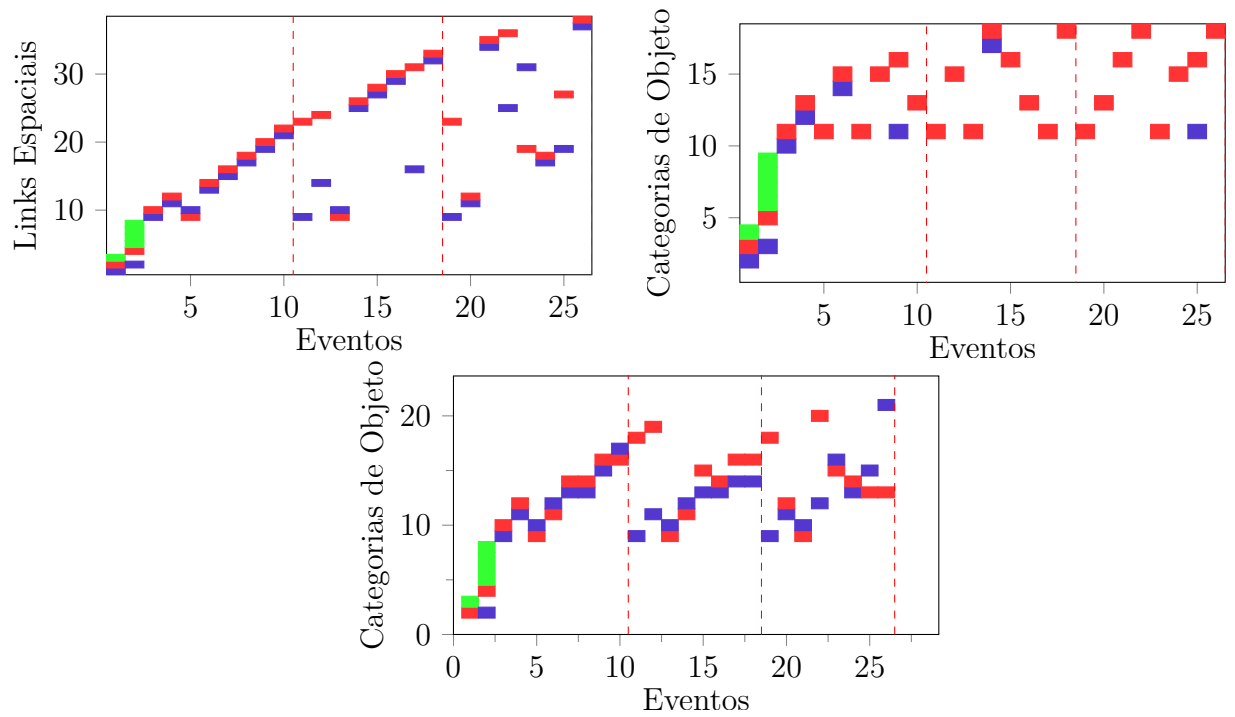
Figura 7.11 – Relações entre eventos e as informações dos links espaciais conectados para execução com limiar de evento 0.01 e objeto 0.3.
