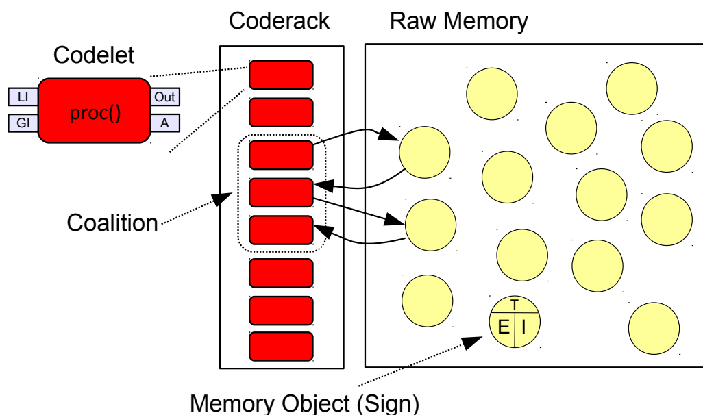
Figura 3.1 – Componentes bases do Cognitive Systems Toolkit - extraído de (PARAENSE et al. , 2016).
