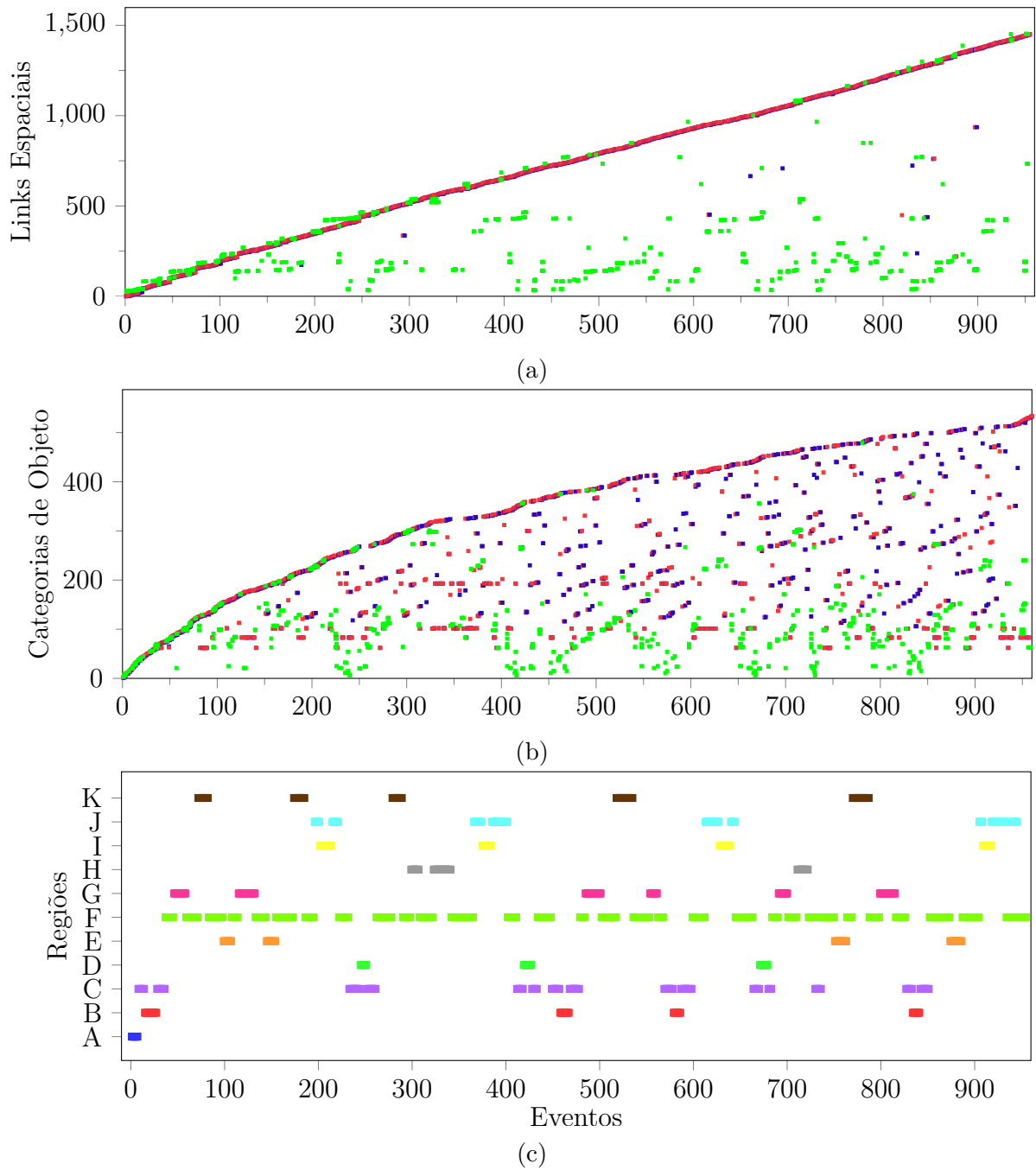
Figura 7.15 – Relação entre nós de eventos e as informações dos links espaciais conectados a eles. (a) Links espaciais conectados aos eventos na memória episódica; (b) Categorias de objetos referidos pelos links espaciais do evento; (c) Região ocupada pelo agente durante o evento. (a,b) Verdes indicam uma conexão do tipo contexto espacial. Azuis indicam uma conexão do tipo início de evento. Vermelhos indicam uma conexão do tipo final de evento. (c) Cada cor e letra de região refere-se as segmentações adotadas na Figura 6.3.
