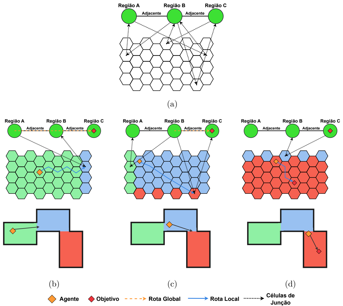
Figura 5.7 – Exemplo de planejamento de rotas realizado pela arquitetura. (a) Representação das regiões conhecidas pelo agente, suas conexões de adjacência e células de junção. As células de junção indicam, para uma dada região, quais células da grade levam a regiões adjacentes e qual é esta região; (b) Planejamento da rota local da região A para B; (c) Planejamento da rota local da região B para C; (d) Planejamento da rota local dentro da região C do agente até o objetivo; (b,c,d) Na parte inferior é mostrado um mapa global do ambiente e a locomoção a ser executada pelo agente correspondente à rota local.
