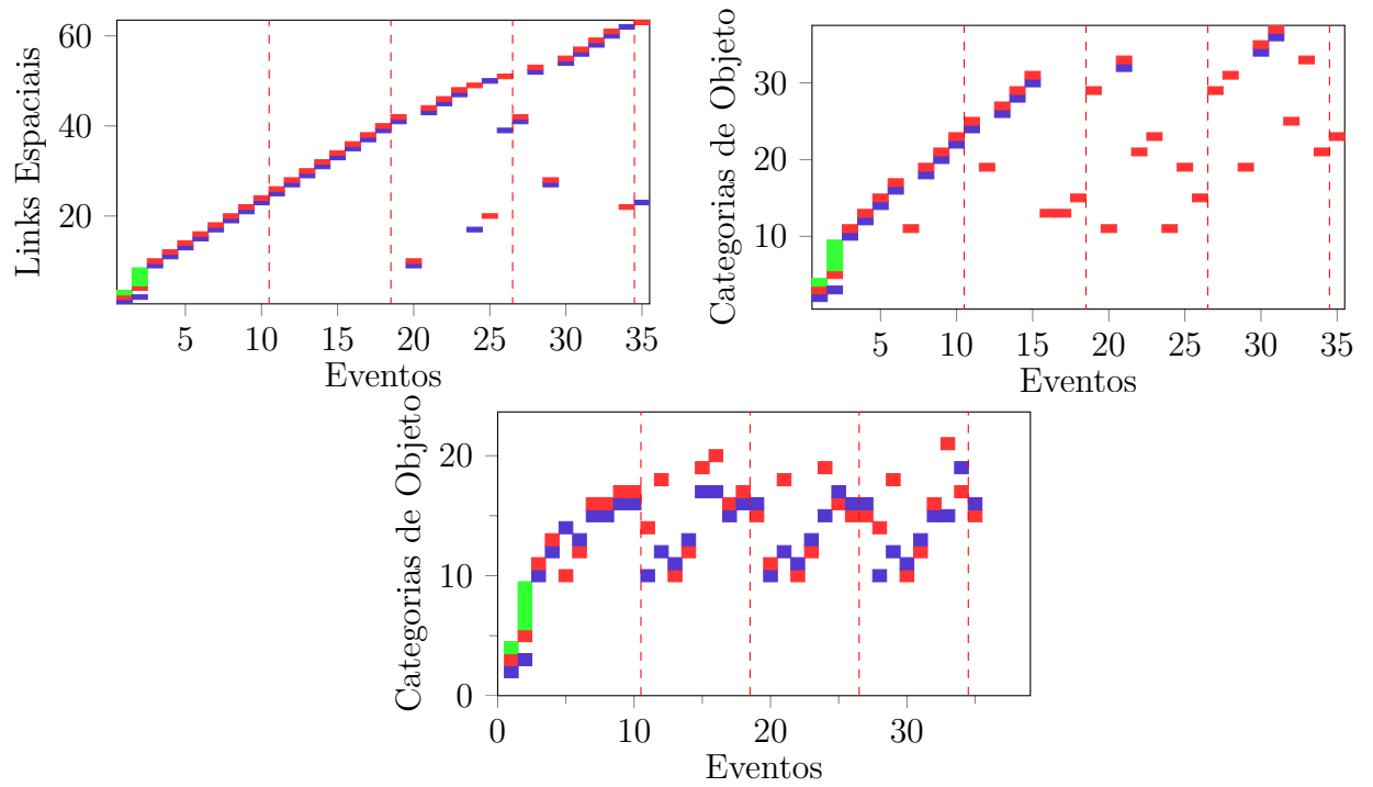
Figura 7.6 – Relações entre eventos e as informações dos links espaciais conectados para execução com limiar de evento 0.01 e objeto 0.8.
