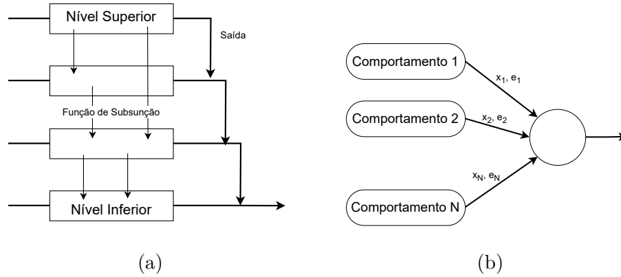
Figura 3.3 – Representação comparativa dos modelos de (a) subsunção clássica e (b) subsunção dinâmica - adaptado de (GUDWIN et al. , 2017)
