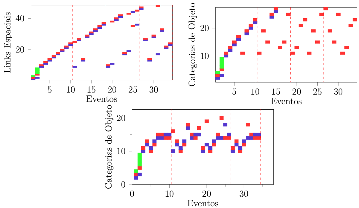
Figura 7.8 – Relações entre eventos e as informações dos links espaciais conectados para execução com limiar de evento 0.01 e objeto 0.6.
