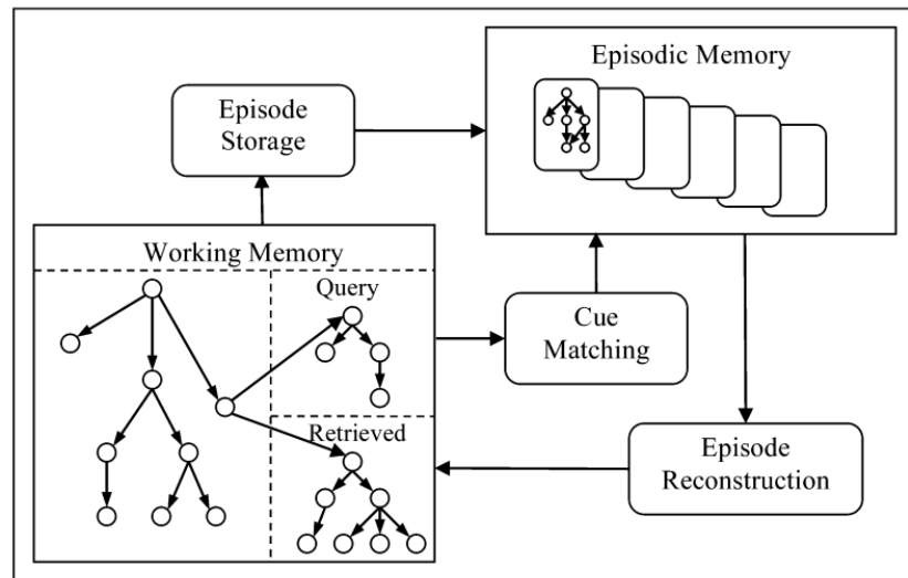
Figura 2.3 – Módulos utilizados para processamento de memórias episódicas na arquitetura SOAR - extraído de Laird (2012) .
