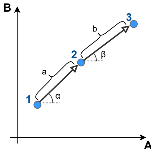
Figura 5.9 – Ilustração da operação de verificação de mudança linear. 1, 2 e 3 são três amostras sequências. Para ser um evento linear, temos que a + b \geq d e |\alpha - \beta| \leq \phi , onde d e \phi são os limiares de comparação.
