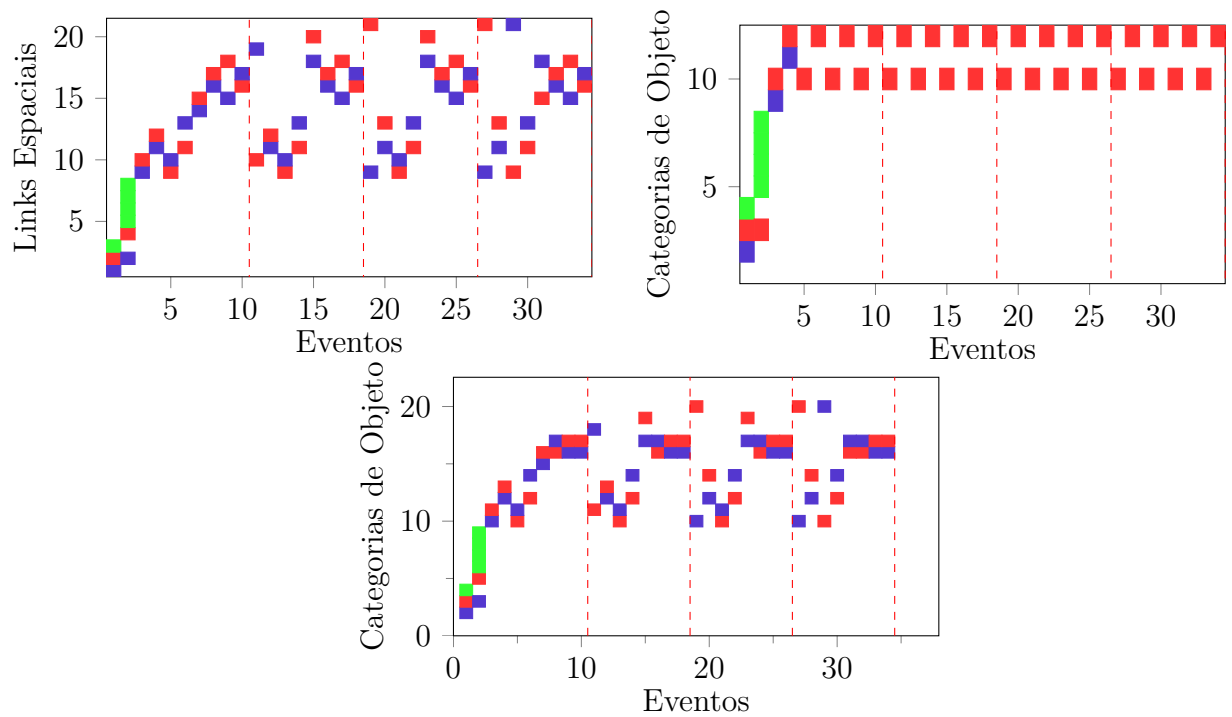
Figura 7.14 – Relações entre eventos e as informações dos links espaciais conectados para execução com limiar de evento 0.01 e objeto 0.0.
