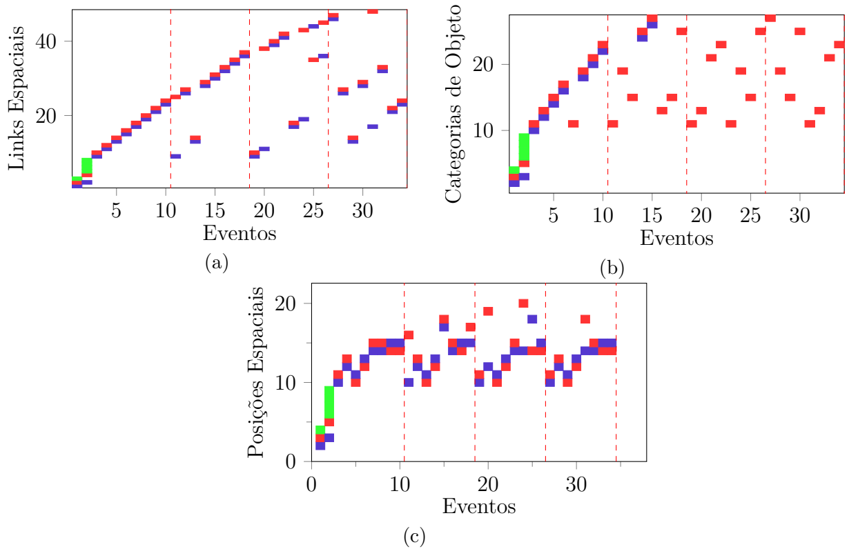
Figura 6.2 – Relação entre nós de eventos e as informações dos links espaciais conectados a eles. (a) Links espaciais conectados aos eventos na memória episódica; (b) Categorias de objetos referidos pelos links espaciais do evento; (c) Células de grade referidas pelos links espaciais do evento. Verdes indicam uma conexão do tipo contexto espacial. Azuis indicam uma conexão do tipo início de evento. Vermelhos indicam uma conexão do tipo final de evento. Linhas tracejadas vermelhas indicam os instantes de segmentação de episódios.
