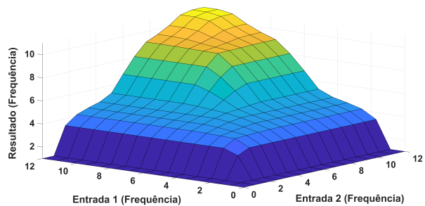
Figura 5.7: Gráfico de Superfície para operador lógico “OU” representando a combinação de diferentes valores de frequência pelo método de Takagi-Sugeno
