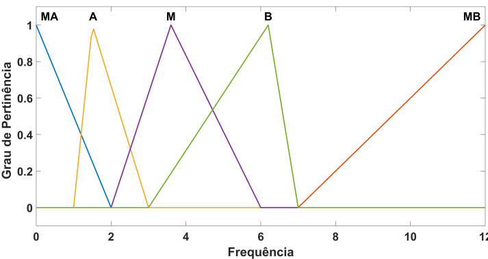
Figura 5.2: Gráfico das Funções de Pertinência que definem cada uma das Variáveis Linguísticas da Frequência para o operador lógico “OU” (Valores de Saída)
