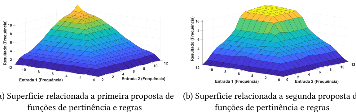
Figura 5.4: Superfície para operador lógico 'OU' representando a combinação de diferentes valores de frequência - Método de inferência Mamdani
