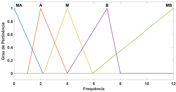
Figura 5.1: Gráfico das Funções de Pertinência que definem cada uma das Variáveis Linguísticas da Frequência para operador lógico “E” (Valores de Saída)
