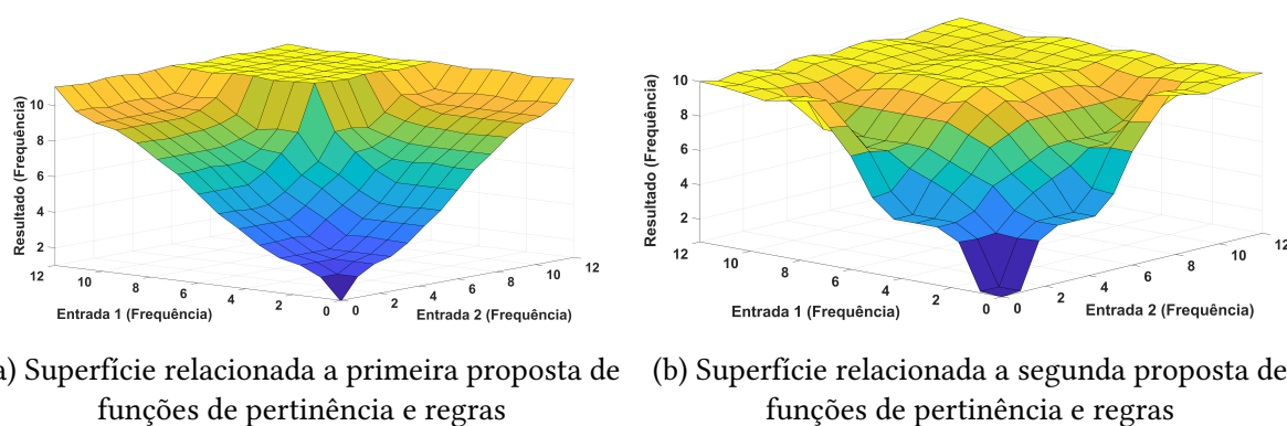
Figura 5.3: Superfície para operador lógico 'E' representando a combinação de diferentes valores de frequência - Método de inferência Mamdani
