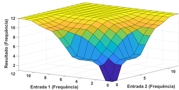
Figura 5.6: Gráfico de Superfície para operador lógico “E” representando a combinação de diferentes valores de frequência pelo método de Takagi-Sugeno
