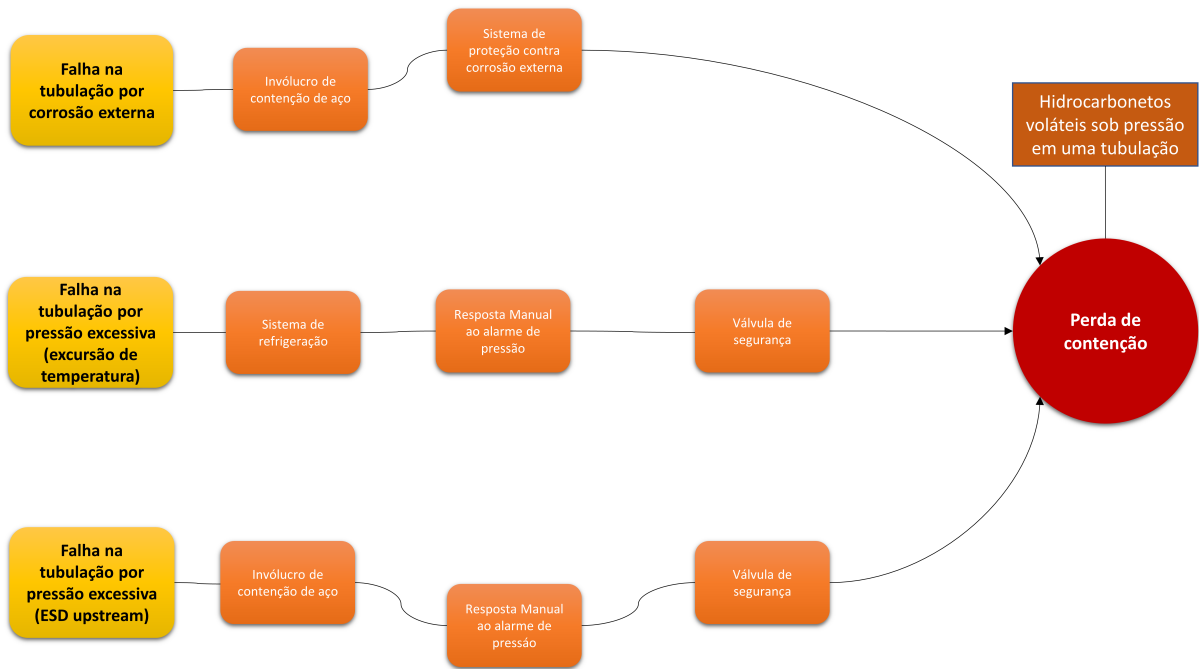
Figura 4.1: Lado esquerdo do Bowtie : Investigação da perda de contenção relacionado
