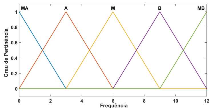
Figura 4.4: Gráfico das Funções de Pertinência que definem cada uma das Variáveis Linguísticas da Frequência (Valores de Entrada)
