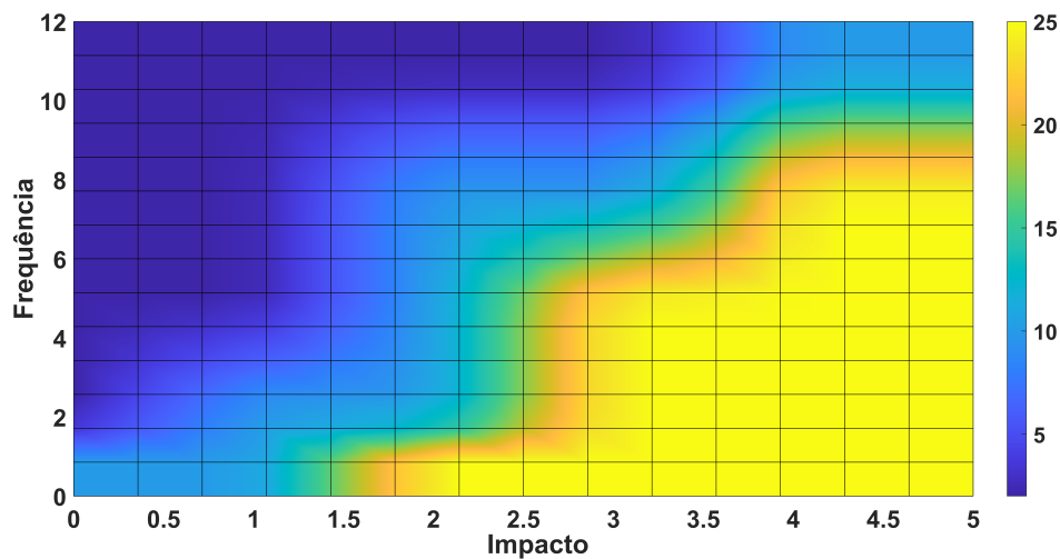
Figura 5.8: Matriz de Risco Fuzzificada pelo Método de Takagi-Sugeno
