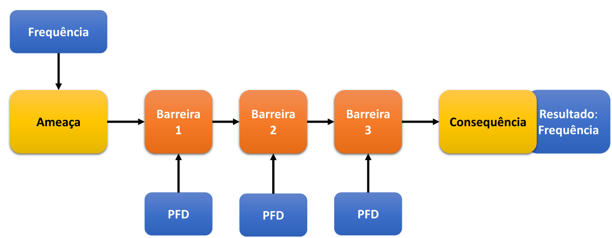
Figura 2.6: Exemplo do diagrama do LOPA
