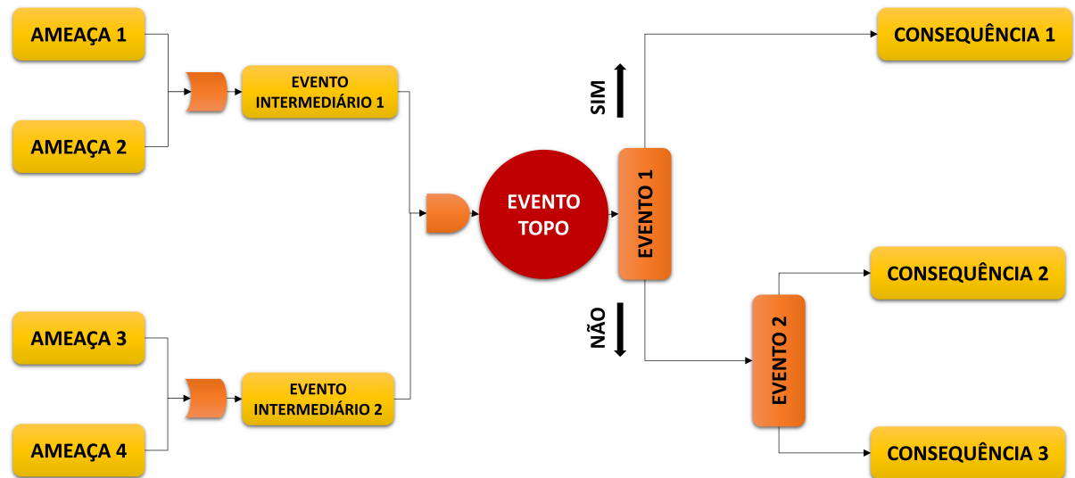
Figura 2.5: Diagrama simples de um bowtie quantitativo
