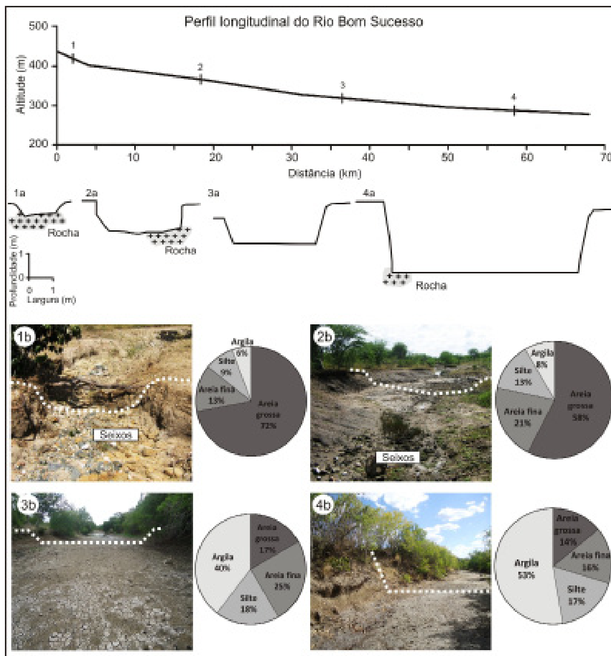
Figura 4 – Perfil longitudinal do Rio Bom Sucesso com sessões transversais e respectivos resultados da análise granulométrica. Fotografias realizadas em janeiro de 2011 e fevereiro de 2012.
