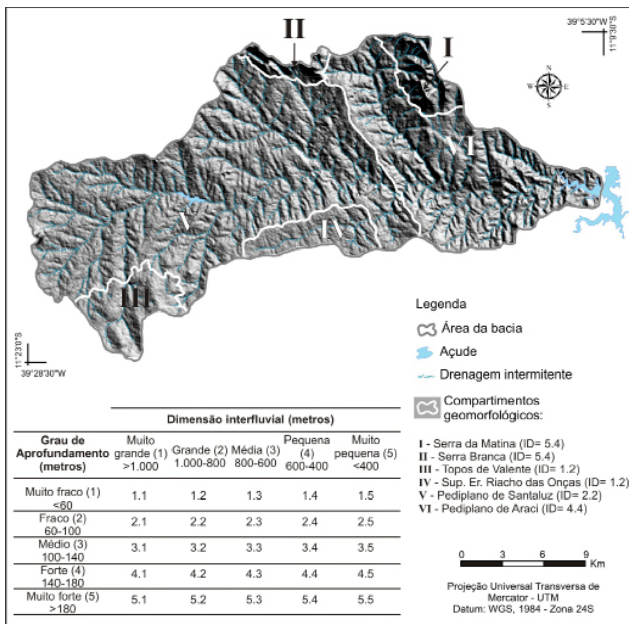
Figura 5 – Ordem de grandeza das formas de dissecação do relevo e respectivos valores dos índices de dissecação (ID) dos compartimentos geomorfológicos.
