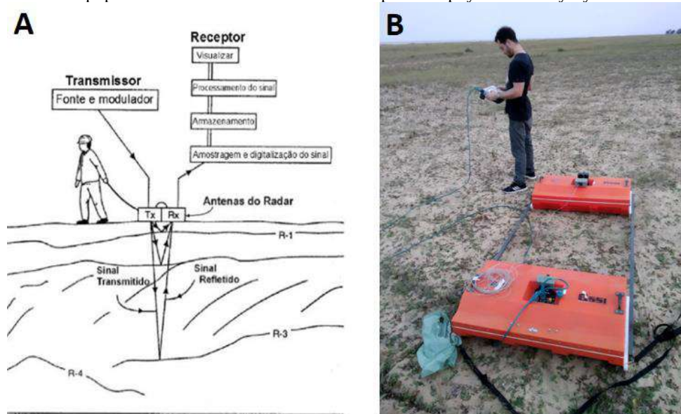
Figura 2 - A: Constituintes básicos de um sistema de GPR (REYNOLDS, 1997). B: exemplo de obtenção de dados com o equipamento modelo SIR3000 fabricado pela Geophysical Survey Systems Inc - GSSI.
