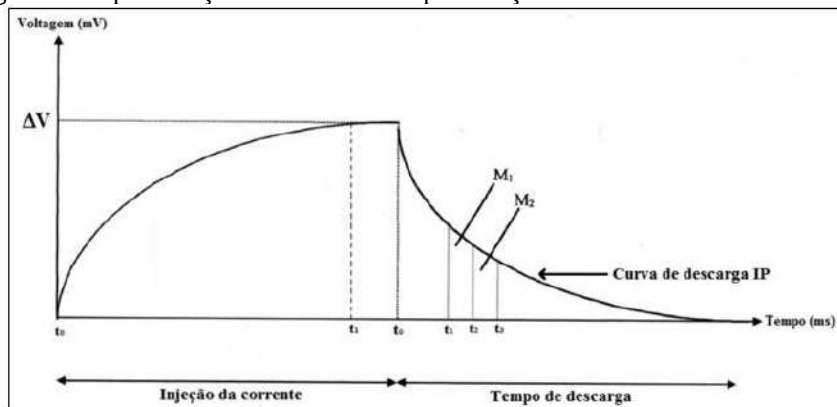
Figura 4 - Representação do fenômeno da polarização induzida no domínio do tempo.
