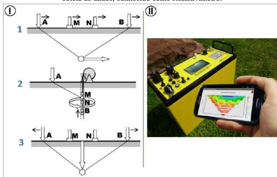
Figura 5 - I: Técnicas de campo mais utilizadas para ensaios geofísicos dos métodos geoeletricos. 1: Caminhamento elétrico; 2: Perfilagem elétrica; 3: Sondagem elétrica. II: Exemplo de equipamento utilizado para coleta de dados, conhecido como Resistivímetro.
