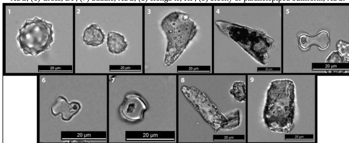
Figura 6 - Principais tipos de fitólitos observados em perfil na região costeira de Cabo Frio-RJ. 1) Globular echinate, XSC; (2) Globular granulate (DF); (3) Cuneiform bulliform, HF; (4) Acicular, XSC; (5) Bilobate, XSC; (6) Cross, DF; (7) Saddle, XSC; (8) elongate, HF; (9) blocky or parallelepiped bulliform, XSC.
