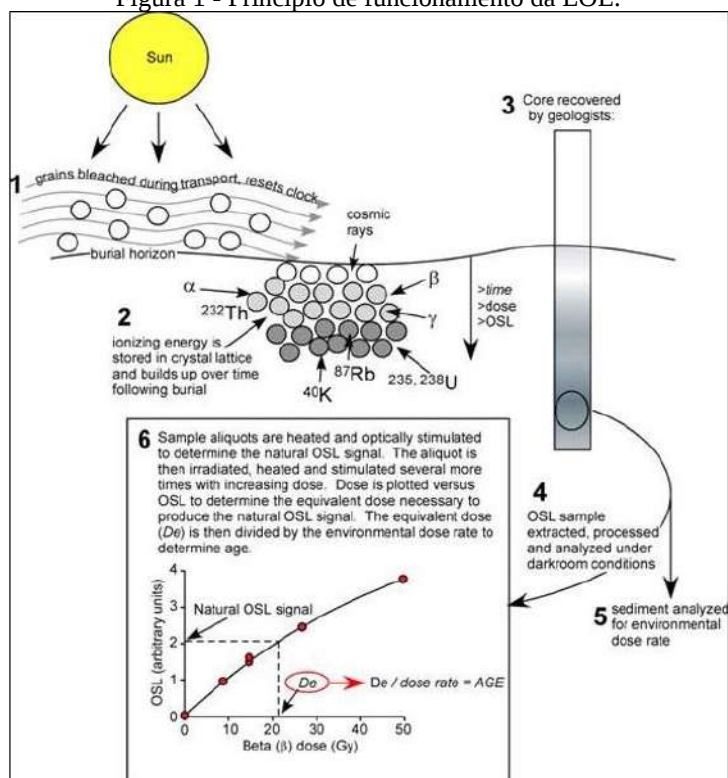
Figura 1 - Princípio de funcionamento da LOE.
