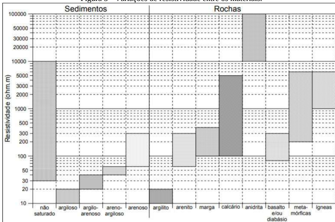
Figura 3 - Variações de resistividade entre os materiais.
