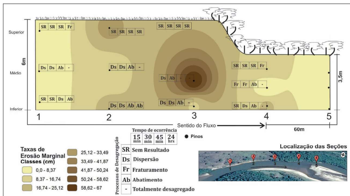
Figura 9 – Distribuição da erosão ao longo da margem da Curva 2 associada a desagregação de materiais segundo o tempo de ocorrência do processo, conforme Quadro 3
