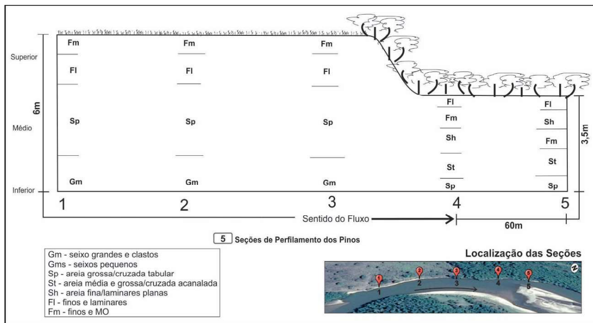
Figura 8 - Disposição faciográfica ao longo da margem da Curva 2, conforme Quadro 2
