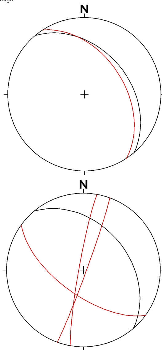
Figura 24. Presença de blocos instáveis na vertente devido a juntas de esfoliação (a), vertente estável e sem formação de cunhas devido à interações de falhas e fraturas (b)
