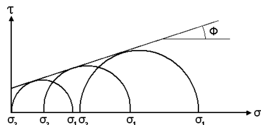
Figura 9. Critério de ruptura de Mohr-Coulomb
