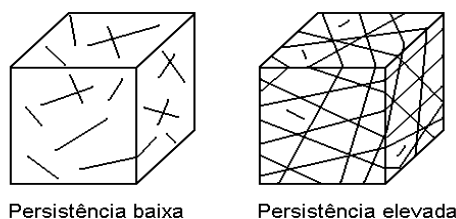
Figura 5. Aspectos da formação de blocos em função da persistência de juntas
