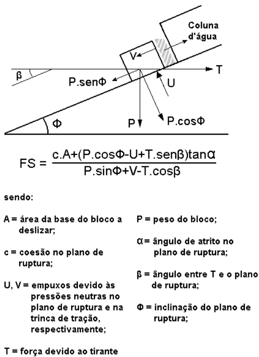
Figura 13. Exemplo de formulação do tipo equilíbrio-limite para o cálculo do FS em uma ruptura planar de um maciço rochoso (Modif. Augusto Fo. e Virgili 1981)
