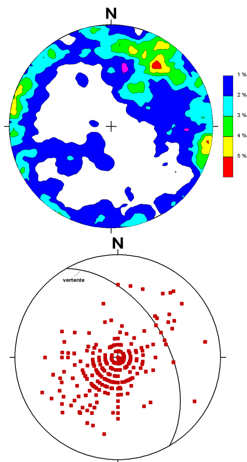
Figura 17. Diagramas de Schmidt das medidas estruturais de juntas em geral e falhas: (a) concentração de polos, (b) orientação da vertente e projeções polares das retas pendentes de mergulho de cada fratura
