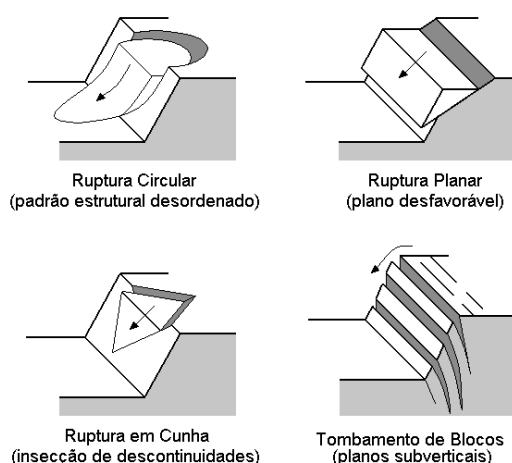
Figura 8. Tipos de ruptura decorrentes da distribuição espacial das discontinuidades em maciços rochosos (Modif. de Hoek e Londe 1974, Piteau e Martin 1981)
