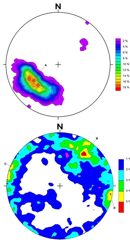
Figura 22. Tratamento estatístico realizado com Stereonet: (a) tratamento estatístico dos dados de juntas de esfoliação mostrando a atitude preferencial A: 57/47 , (b) tratamento estatístico dos dados de fraturas e falhas apresentando as atitudes preferenciais C: 110/87 e D: 289/85 (citadas por Santoro et. al. 1979) e o novo sistema preferencial B: 216/64
