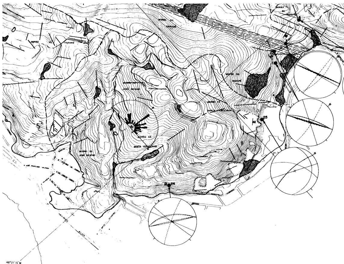
Figura 14. Mapa estrutural do Morro Santa Terezinha contendo os sistemas preferenciais persistentes de descontinuidades e a rosácea de fotlineamentos dessa unidade de análise (Santoro et. al. 1979)
