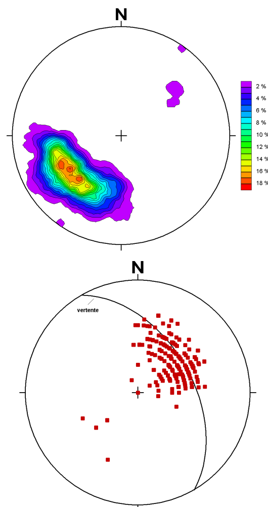
Figura 18. Diagramas de Schmidt das medidas estruturais de juntas de esfoliação: (a) concentração de polos, (b) vertente e projeções polares das retas pendentes de mergulho de cada junta de esfoliação
