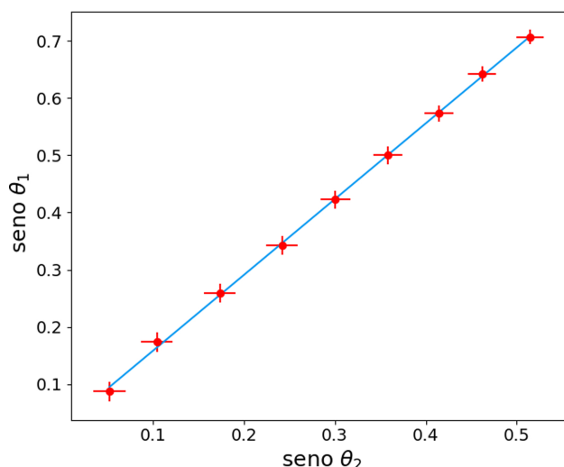
Figura 8: Gráfico das medidas realizadas para calcular o índice de refração da gelatina através do ajuste linear da reta.
