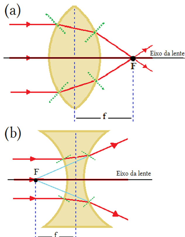
Figura 2: a) Lente biconvexa e b) Lente bicôncava. Em vermelho os raios incidentes e em verde as retas normais às respectivas interfaces. O ponto "F" é o foco da lente e "f" a distância focal para o caso particular de uma lente delgada. A linha preta marca o eixo óptico das lentes.
