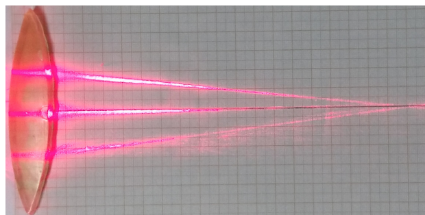
Figura 9: Experimento realizado com uma lente de gelatina biconvexa sobre um papel milimetrado. Com o auxílio de uma régua e um lápis é possível traçar o caminho do feixe de luz e então a partir do encontro das três retas medir a distância focal da lente.
