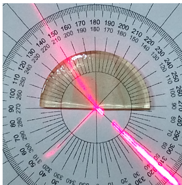
Figura 7: Experimento realizado para calcular o índice de refração da gelatina. Na imagem aparecem os feixes: incidente, refratado e refletido.
