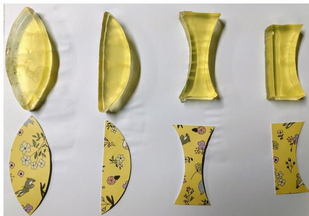
Figura 4: Algumas lentes cortadas seguindo os gabaritos feitos em folha de cartolina.
