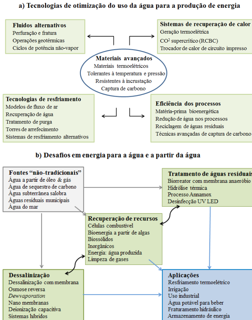
FIGURA 11 – Problemas e oportunidades tecnológicas para onexo água-energia.
