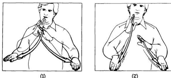
Figura 1 – O sinal (1) é QUIET e (2) é ACQUIESCE (BAKER-SHENK; COKELY, 1982, p. 41)
