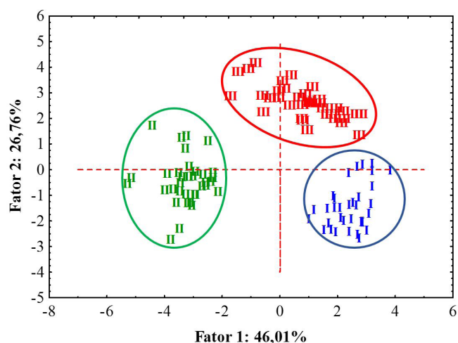
Figura 2. Análise de componentes principais dos atributos físicos nos diferentes sistemas de usos. I = pastagem; II = milho; III = floresta.
