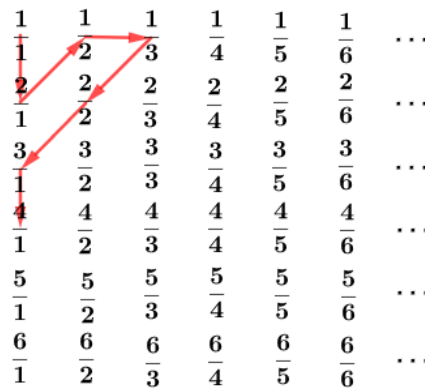
Figura 10: Observando f(7) a fim de conjecturar uma fórmula para o caso em que \alpha é ímpar e r \neq 0 .
