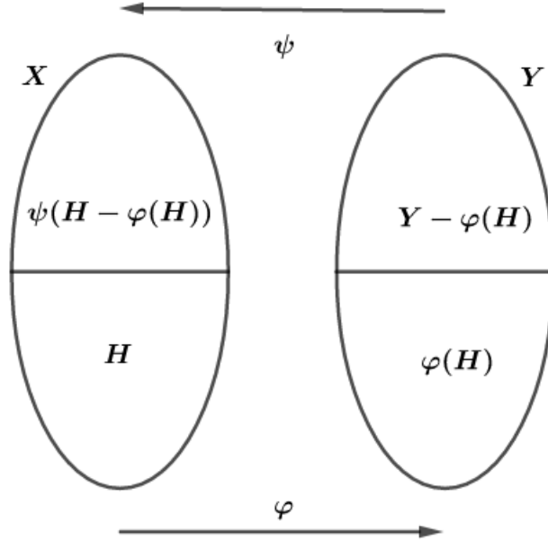
Figura 15: Visualização gráfica da demonstração do Teorema 35 - (ii) .
