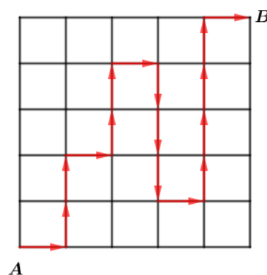
Figura 4: Um caminho diferente.
