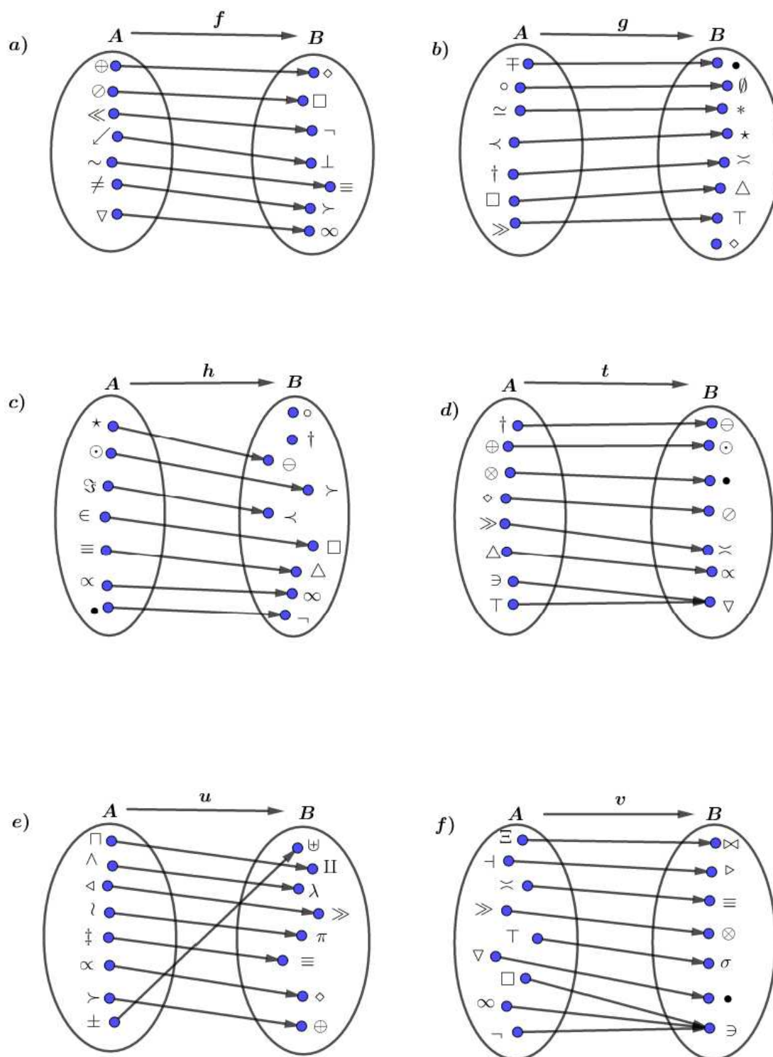
Figura 16: Conjuntos e funções do Exercício 1.
