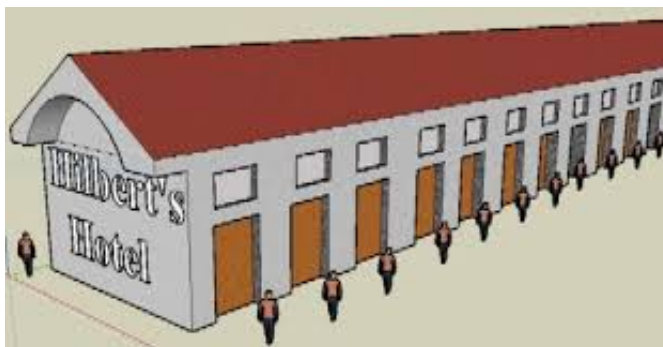
Figura 17: Uma ilustração para o Hotel de Hilbert.
