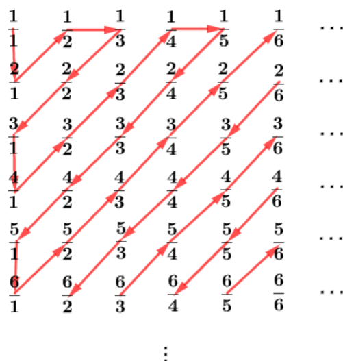
Figura 20: Uma possível solução para o item a) do Exercício 3.
