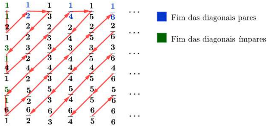
Figura 9: Fim das diagonais pares e ímpares pelo caminho.
