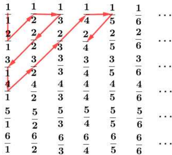
Figura 8: Exemplificando o caso particular da décima-segunda fração.
