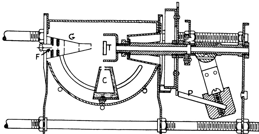
Fig. 5.2 – Corte transversal da aparelhagem experimental de Davisson e Germer. As letras representam: G – disparador de elétrons; T – alvo; C – dupla caixa coletora de Faraday, P – dois pratos que teriam a função de auxiliar na concentração da emissão do filamento
