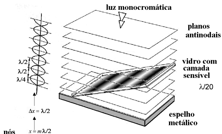
Fig. 3.2 – Esquema explicativo do experimento de Wiener (1890). Um feixe de luz monocromática incide perpendicularmente a um espelho metálico. Formam-se ondas estacionárias, sendo o plano do espelho uma região nodal. Os planos nodais e anti-nodais são paralelos ao espelho. Um vidro com uma camada fotossensível é colocado em uma posição inclinada, próximo ao espelho (o ângulo está muito exagerado, na figura). A intersecção entre a camada fotossensível e a figura de interferência da luz produz uma série de regiões claras e escuras, paralelas, na película, após a revelação.
