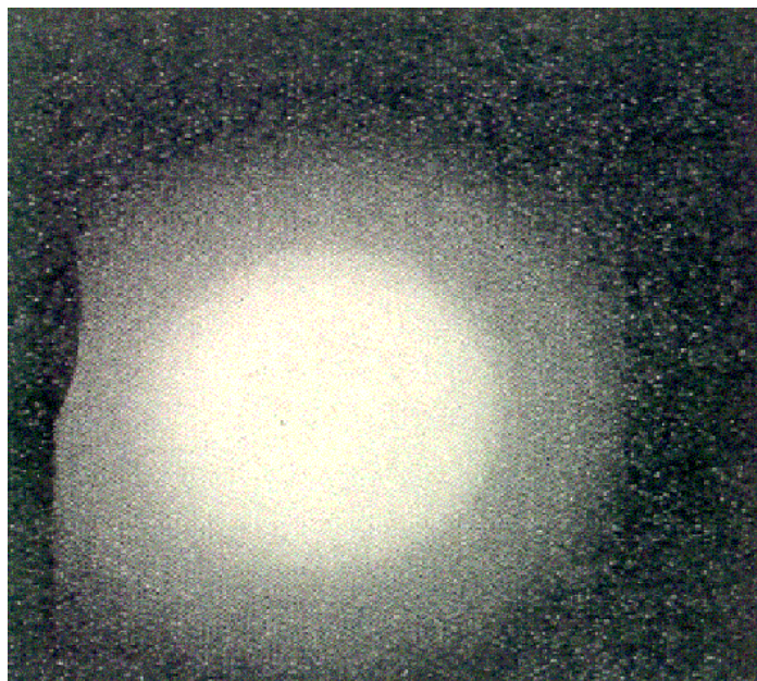
Fig. 5.1 – Fotografia de difração de elétrons obtida por Thomson e Reid
