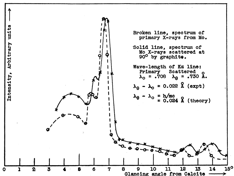
Fig. 2.2 – Gráfico obtido por Compton em 1923. A curva tracejada representa o espectro de raio X primário do Mo; a linha sólida corresponde ao espectro de raio X do Mo espalhado num ângulo de 90° pela grafite. O comprimento de onda da linha K \alpha calculado por Compton corresponde a: comprimento de onda primário ( \lambda_0 = 0.708 \text{ \AA} ); espalhado ( 0.730 \text{ \AA} ).
