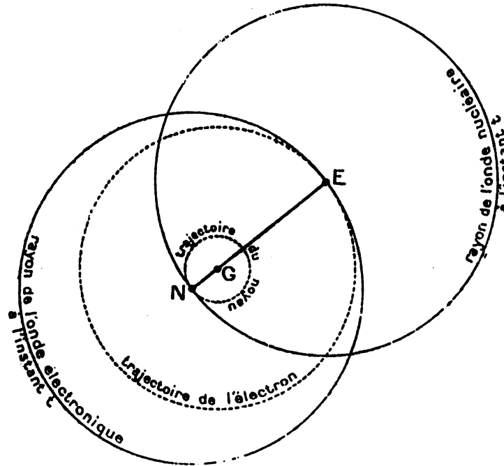
Fig. 4.2 – Figura esquemática de De Broglie, mostrando o movimento do elétron e do núcleo atômico em torno do centro de massa (DE BROGLIE, 1925a, p. 75).
