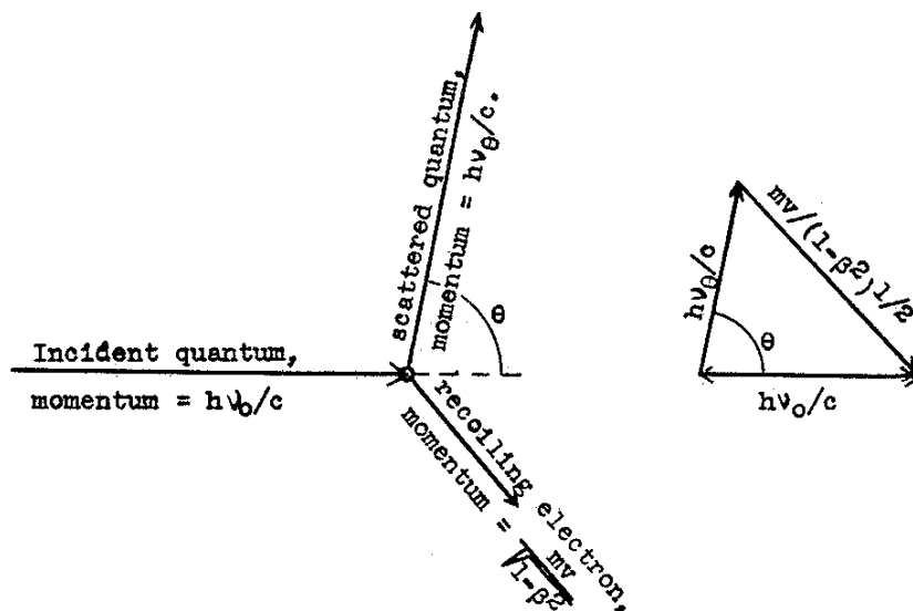
Fig. 2.1 – Desenho esquemático de Compton
