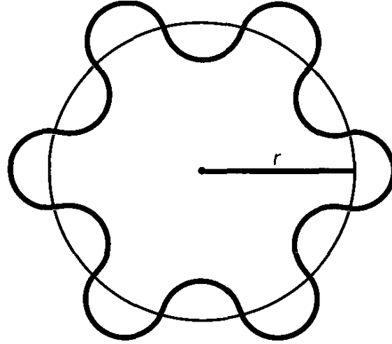
Fig. 4.1 – Ilustração didática da condição de quantização de De Broglie.
