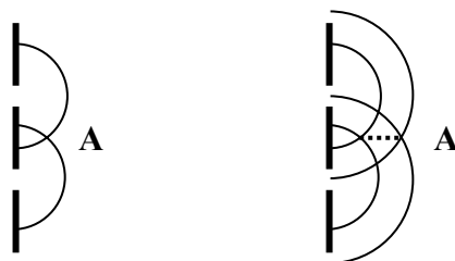
Fig. 4.3 – A velocidade do ponto de interseção das ondas que passam por duas fendas pode ser maior do que a velocidade de cada uma dessas ondas.
