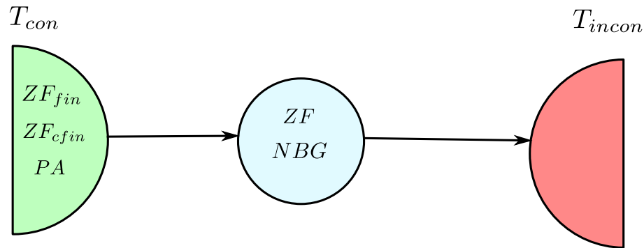
Figura 5 – Universo com PA2(mod).
