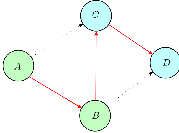
Figura 4 – Uso simultâneo de duas metodologias
