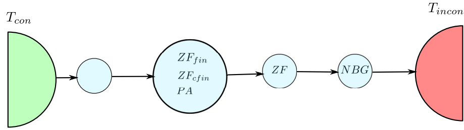
Figura 6 – Universo com PA(int).
