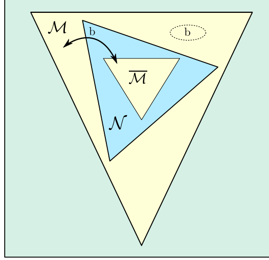
Figura 2 – Relação entre modelos semi-bi-interpretáveis.
