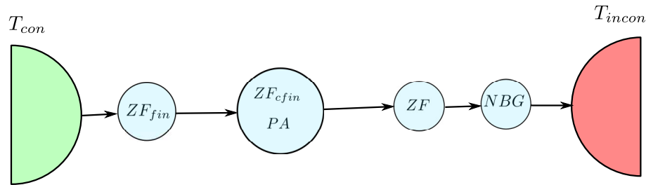
Figura 8 – Universo com toda a hierarquia
