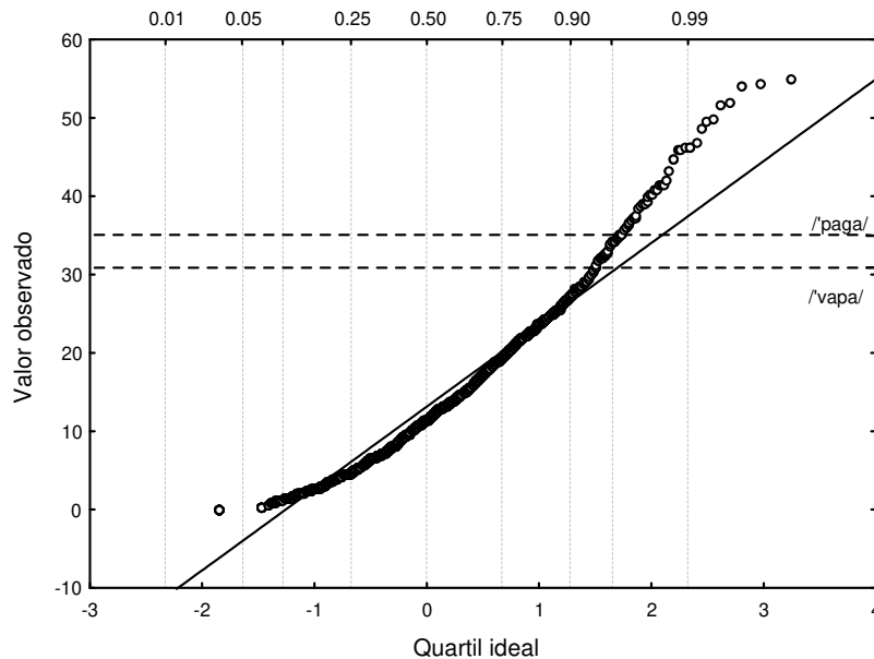
Figura 4.1: Distribuição de ['pa\eta] e ['va\eta] na distribuição normal teórica de SFV para quatro segmentos.
