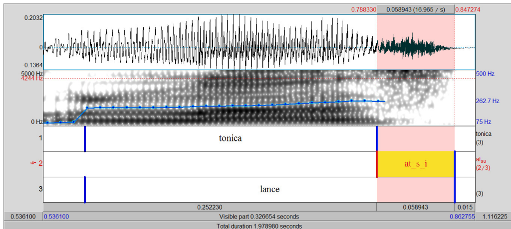
Figura 7: Exemplo de /i/ vozeado em (a) e /i/ desvozeado em (b) para a palavra “lance” /laNsi/. As porções destacadas indicam em (a) periodicidade da vogal vozeada e em (b) a extensão do desvozeamento total.
