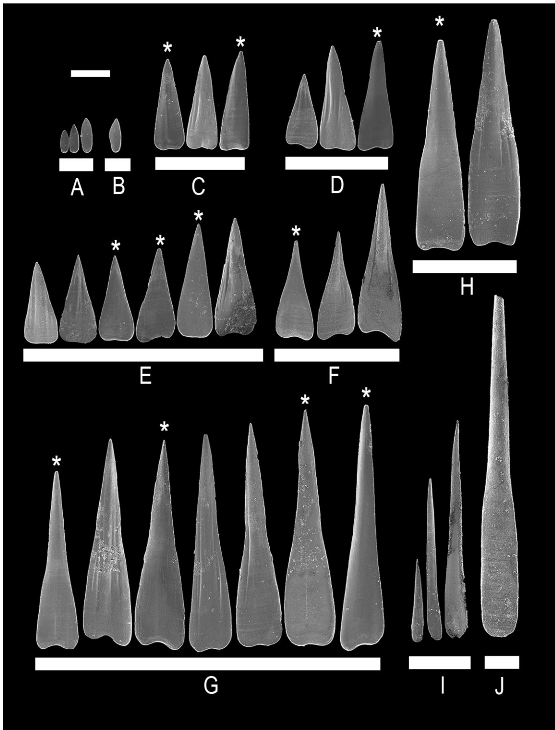
Figura 6: Falcidens n. sp. Micrografia eletrônica de varredura das escleritos isoladas das diferentes partes do corpo: (A-B) no Anterium; (C-D) no Pescoço; (E-G) no Tronco; (H-J) no Posterium. Os asteriscos mostram a face voltada para o corpo. Escala = 60 \mu m.
