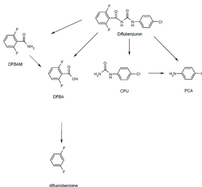
Fig. 1. Diflubenzuron (DFB) e produtos da sua degradação em água e solo. DFBA= ácido 2,6-difluorobenzóico, DFBAM= 2,6-difluorobenzamida, CPU= p-clorofeniluréia, PCA= p-cloroanilina (Nimmo et al., 1984).
