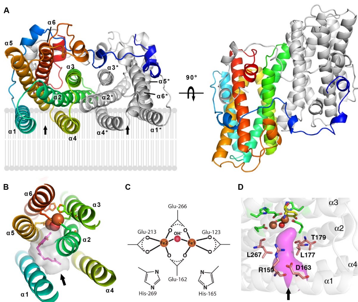
Figura 6. Estrutura da AOX. (A) Representação em cartoon da estrutura cristalográfica da AOX de T. brucei (TAO; PDB ID 3w54) e modelagem da interação com a membrana fosfolipídica. Um dos monômeros está colorido da porção N-terminal (azul) para a C-terminal (vermelho), e o outro monômero está em cinza. Setas indicam a entrada do sítio catalítico voltada para a membrana fosfolipídica. (B) e (C) Destaque dos íons de ferro e resíduos de aminoácido envolvidos em sua coordenação, bem como o inibidor coetochlorina B ( stick magenta) dentro do sítio de interação com o substrato (sombreamento cinza). (D) Modelo estrutural da AOX de Sauromatum guttatum , exibindo o sítio de ligação ao substrato (superfície magenta), os resíduos de coordenação com o ferro ( stick verde), os resíduos que orientam o substrato para a conformação favorável à reação enzimática ( stick magenta) e a tirosina envolvida na catálise ( stick amarelo). Adaptado de [28–30].
