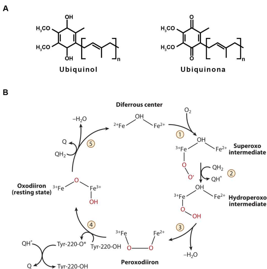
Figura 7. Mecanismo catalítico da AOX. (A) Estrutura do ubiquinol e da ubiquinona. Na mitocôndria, as formas mais comuns são com 9 e 10 unidades isoprênicas (Q 9 e Q 10 ). (B) Mecanismo catalítico parcialmente proposto. Retirado de [29].
