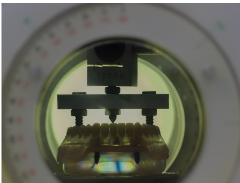
Figura 12. Célula de aplicação de carga, simulando uma oclusão balanceada bilateralmente.
