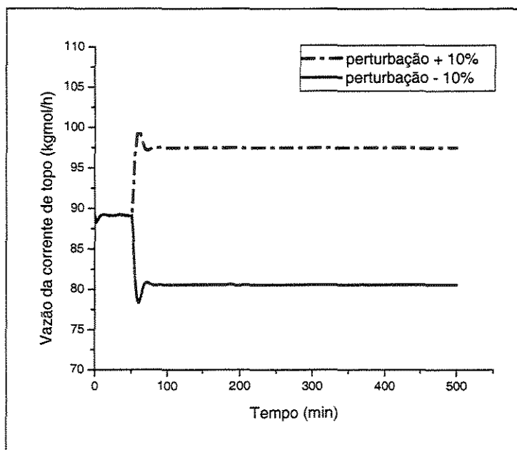
Figura 6.19: Vazão da corrente de topo
