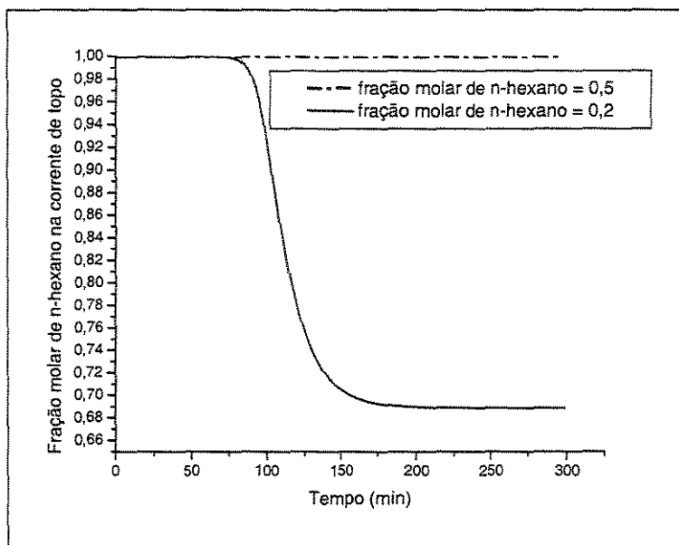
Figura 5.18: Fração molar de n-hexano na corrente de topo
