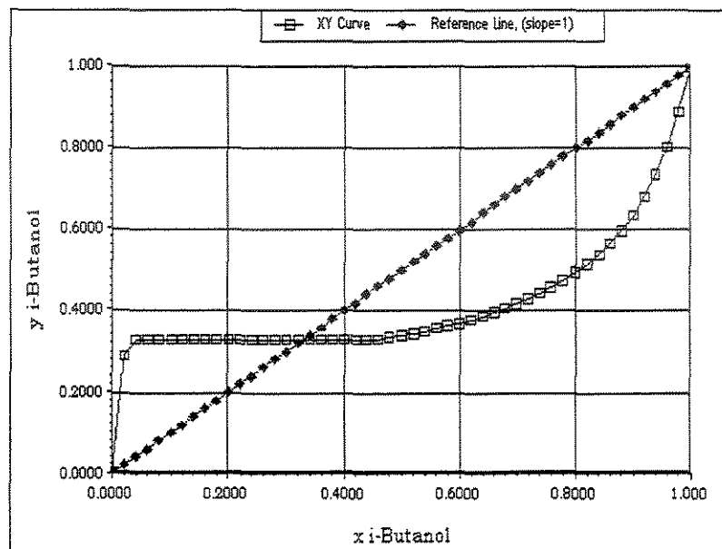
Figura 2.5: Diagrama de equilíbrio líquido-vapor (xy) para a mistura isobutanol (1)/água (2) a 1 atm.
