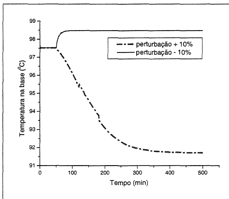
Figura 5.4: Temperatura na base da coluna
