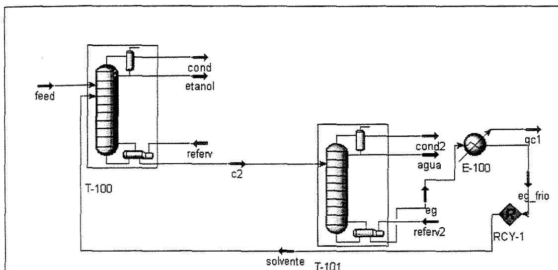
Figura 4.1: Fluxograma para o processo de destilação extrativa
