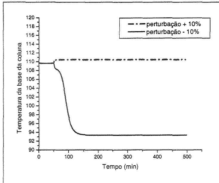
Figura 6.31: Temperatura na base da coluna
