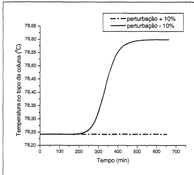
Figura 6.3: Temperatura no topo da coluna
