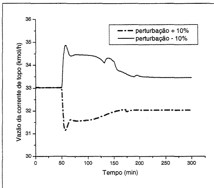
Figura 5.13: Vazão da corrente de topo
