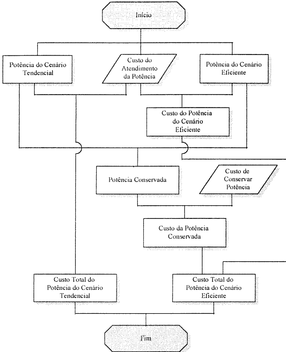
Figura 2. 8: Fluxograma dos Custos da Potência Instalada
