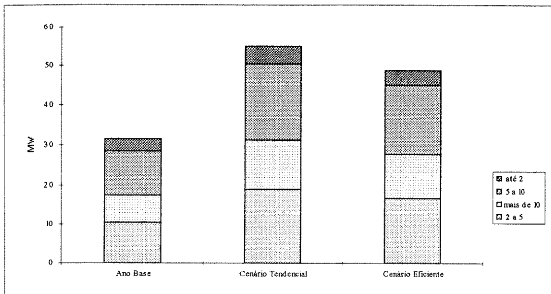
Gráfico 5. 6: Potência Instalada por Faixa de Renda no Setor Residencial da RAC (área rural)
