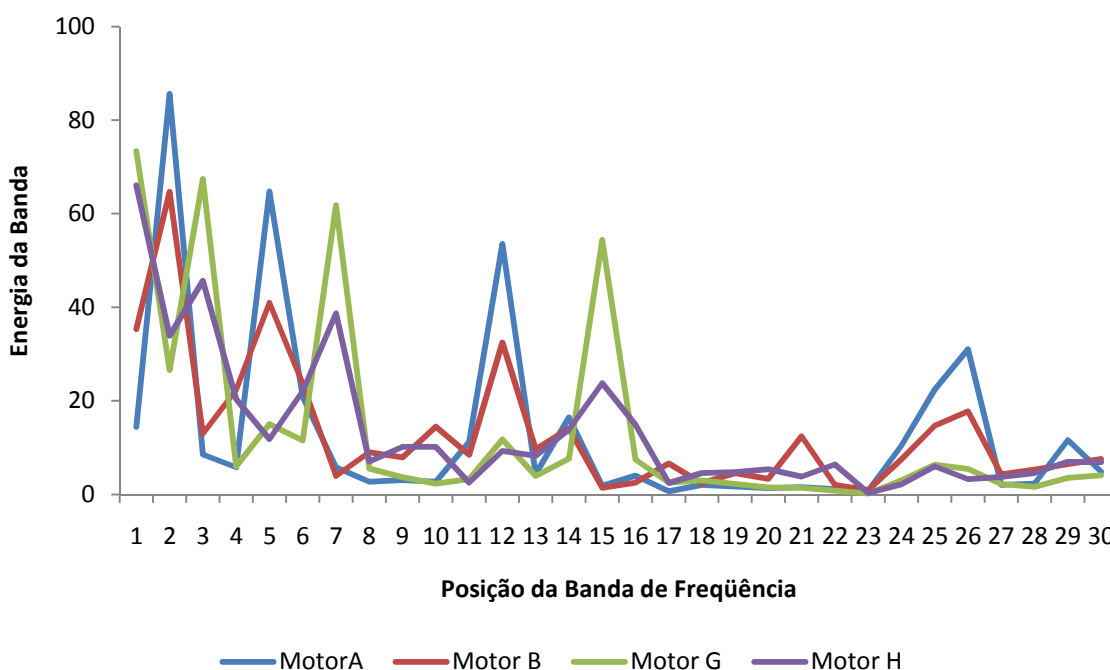
Figura 4.17 - Níveis de energia para a condição de 4000 rpm, em máximo torque.
