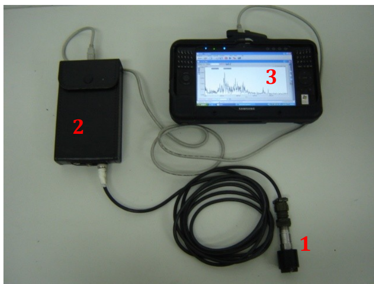
Figura 4.4 – Sistema de análise de vibrações composto por: 1. Acelerômetro piezoeletrico; 2. Conversor analógico/digital; 3. Computador portátil com software de processamento de sinais.
