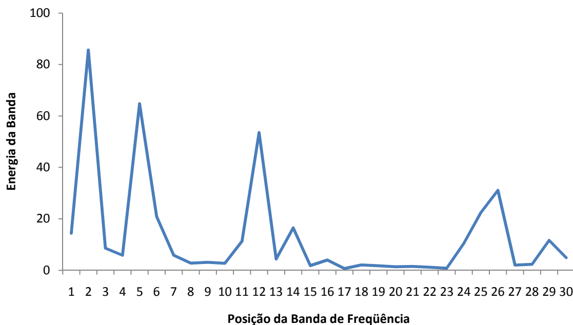
Figura 4.12 – Níveis de energia em cada banda da WTP, a 4000 rpm, com limite de medição a 2 kHz.
