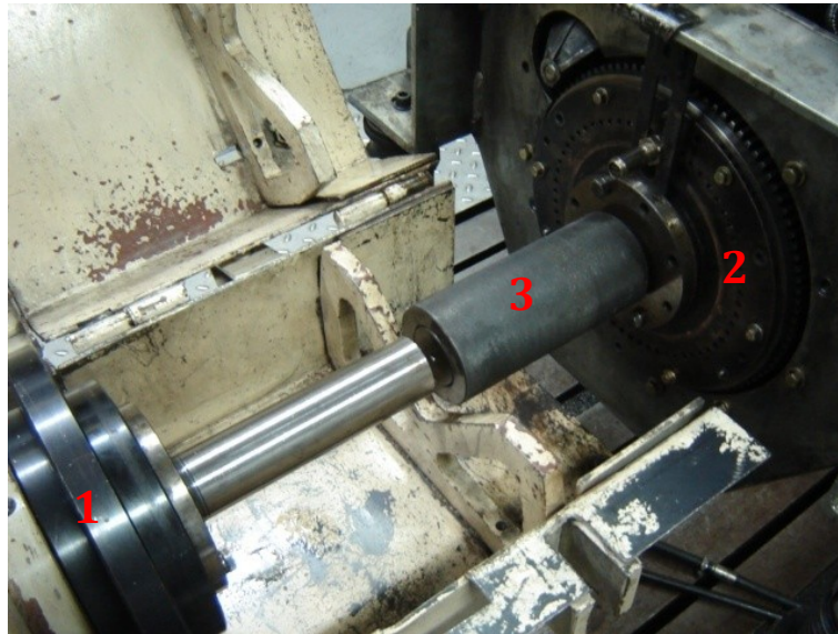
Figura 4.2 – Processo de alinhamento do motor ao dinamômetro: 1. Flange do dinamômetro com eixo de alinhamento montado. 2. Volante do motor com o eixo de alinhamento montado. 3. Buscha deslizante (passa não passa) para verificação do alinhamento entre os dois eixos.
