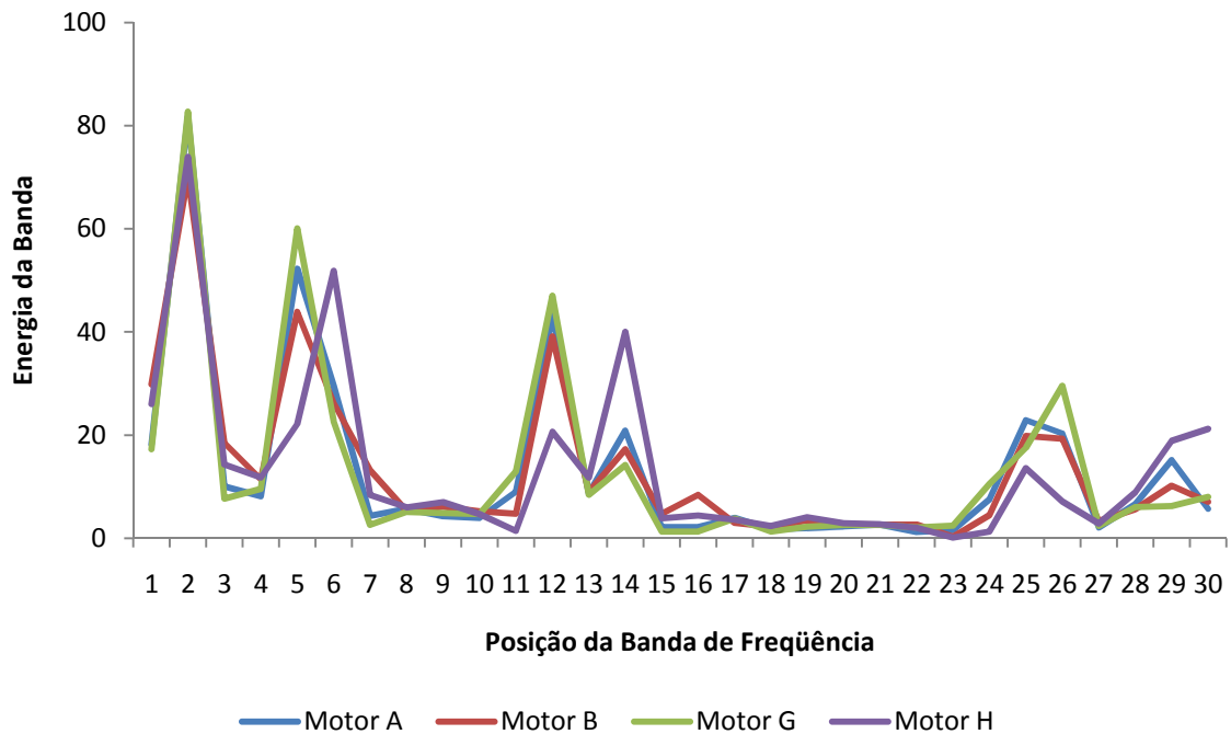
Figura 4.23 - Níveis de energia para a condição de 1600 rpm, em máximo torque.
