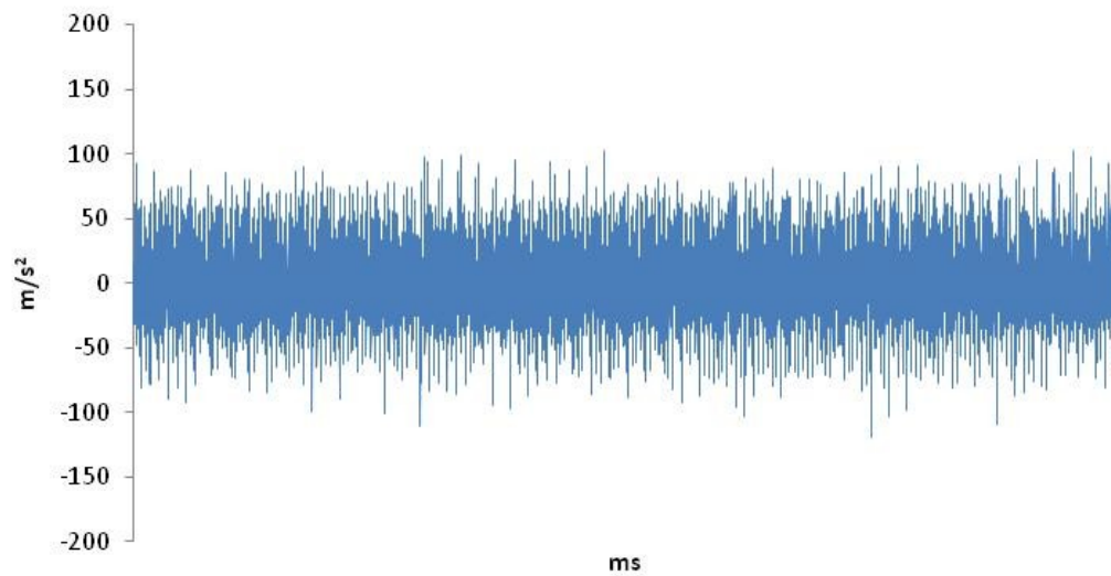
Figura 4.6 – Sinal da amplitude da aceleração em função do tempo, sem nenhum tipo de tratamento matemático, de um motor NGD funcionando a 4000 rpm na condição de mínimo torque.
