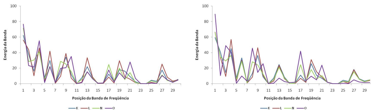
Figura 4.27 – Níveis de energia em cada um dos nós da WTP para (a) 1400 rpm (b) 1200 rpm.
