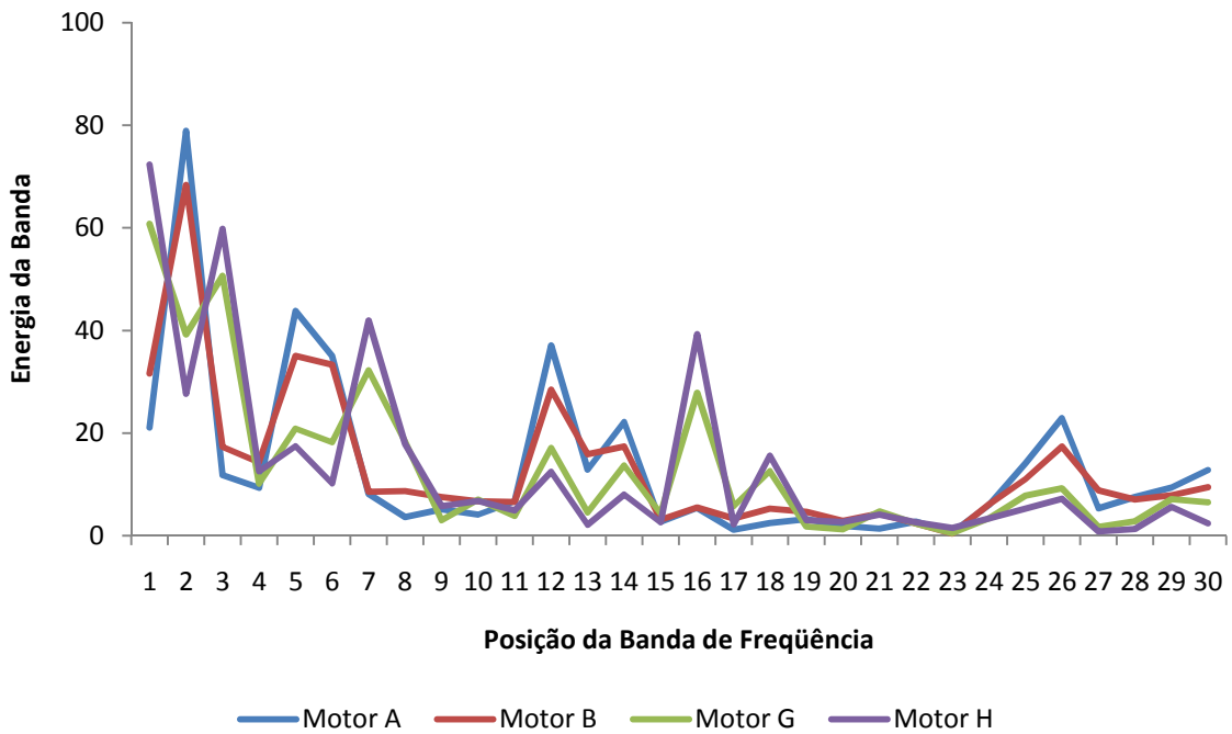
Figura 4.19 - Níveis de energia para a condição de 3200 rpm, em máximo torque.
