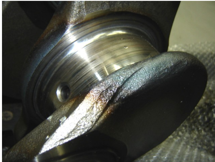
Figura 4.14 – Virabrequim do motor com sinais de agarramento, junto à posição de montagem da bronzina.
