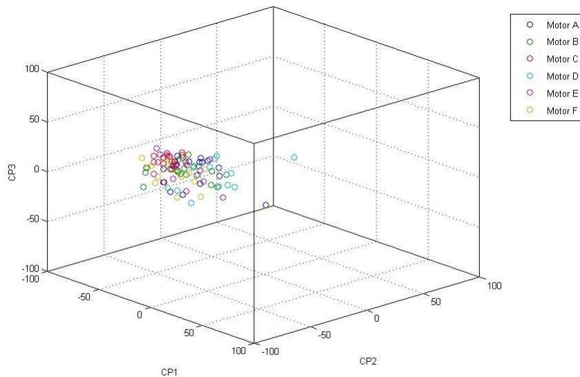
Figura 4.29 – Validação do polinômio de resposta. Motores A, B, C, D, E foram utilizados na elaboração do polinômio. Os vetores CP1 \times CP2 \times CP3 para o motor F foram obtidos a partir do polinômio já elaborado, no plano ( CP1; CP2; CP3 ).
