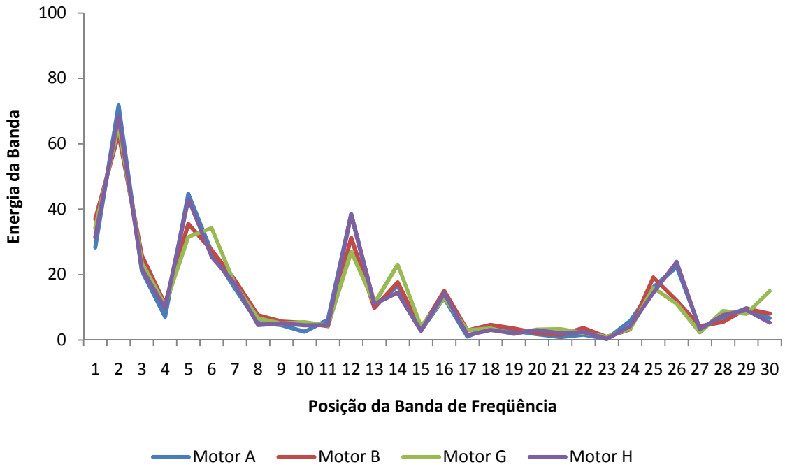
Figura 4.18 - Níveis de energia para a condição de 3600 rpm, em máximo torque.
