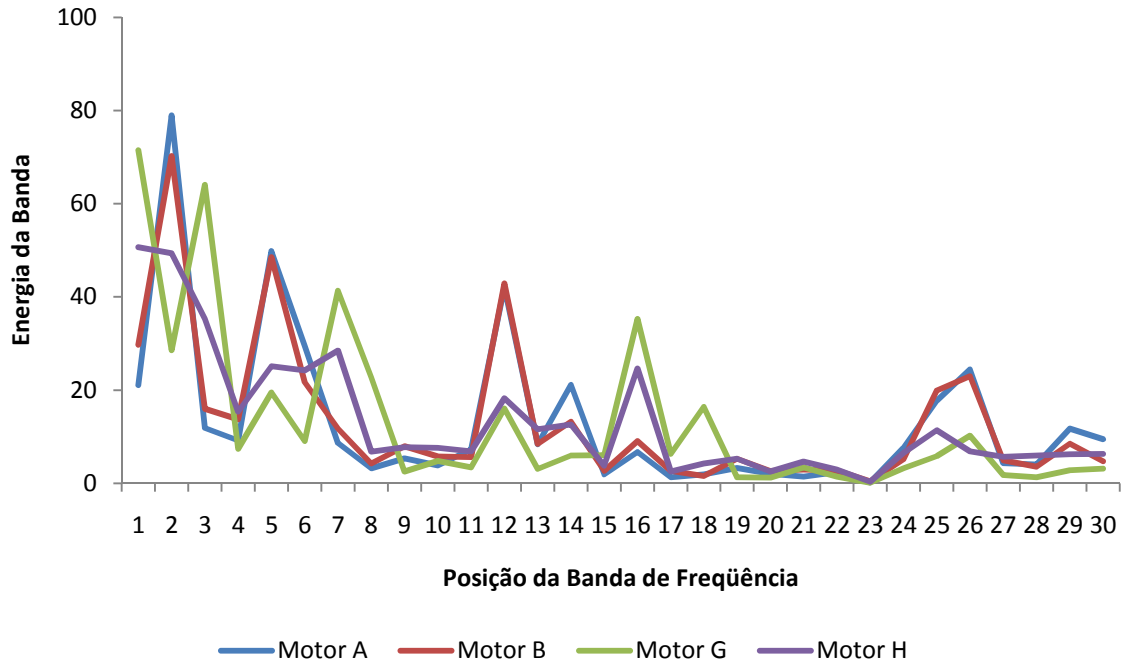
Figura 4.20 - Níveis de energia para a condição de 2800 rpm, em maximo torque.
