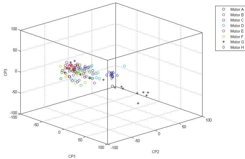
Figura 4.30 – Polinômio validado com motores defeituosos - Motores A, B, C, D, E, F são motores em condições normais de funcionamento. Os motores G, H são motores que apresentam agarramento de bronzina de biela, no plano ( CP1; CP2; CP3 ).
