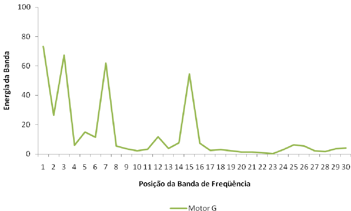
Figura 4.15 – Níveis de energia de aceleração para o motor (com início de agarramento) funcionando a 4000 rpm em máximo torque, obtido com base na WTP.
