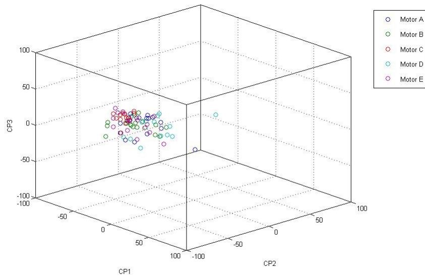
Figura 4.28 - Resultados obtidos a partir da Análise de Componentes Principais para 5 motores (grupo 1) em condições normais de funcionamento, no plano ( CP1 ; CP2 ; CP3 ).
