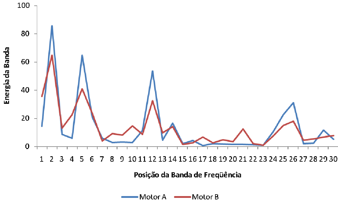
Figura 4.13 - Semelhança entre os níveis de energia de motores 2 motores , rodando a 4000 rpm em condições normais de funcionamento.
