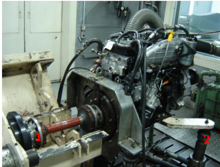
Figura 4.3 – Instalação do motor junto ao dinamômetro concluída. 1. Eixo cardan instalado, interligando motor ao dinamômetro 2. Coxins de borracha utilizados para isolar as vibrações motor e ambiente.
