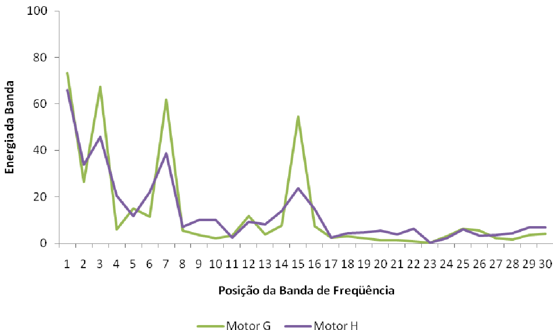
Figura 4.16 - Níveis de Energia para a condição de 4000 rpm, em máximo torque, de motores defeituosos.
