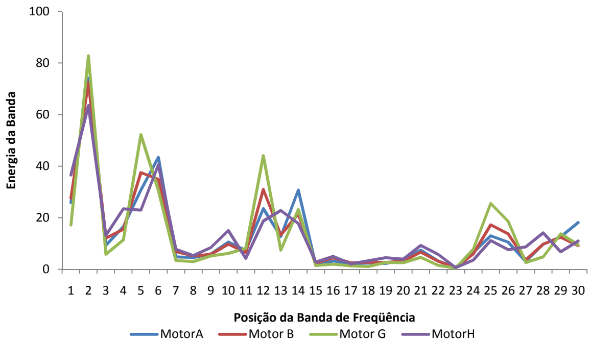
Figura 4.22 - Níveis de energia para a condição de 2000 rpm, em máximo torque
