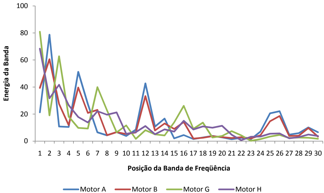
Figura 4.21 - Níveis de energia para a condição de 2400 rpm, em máximo torque.
