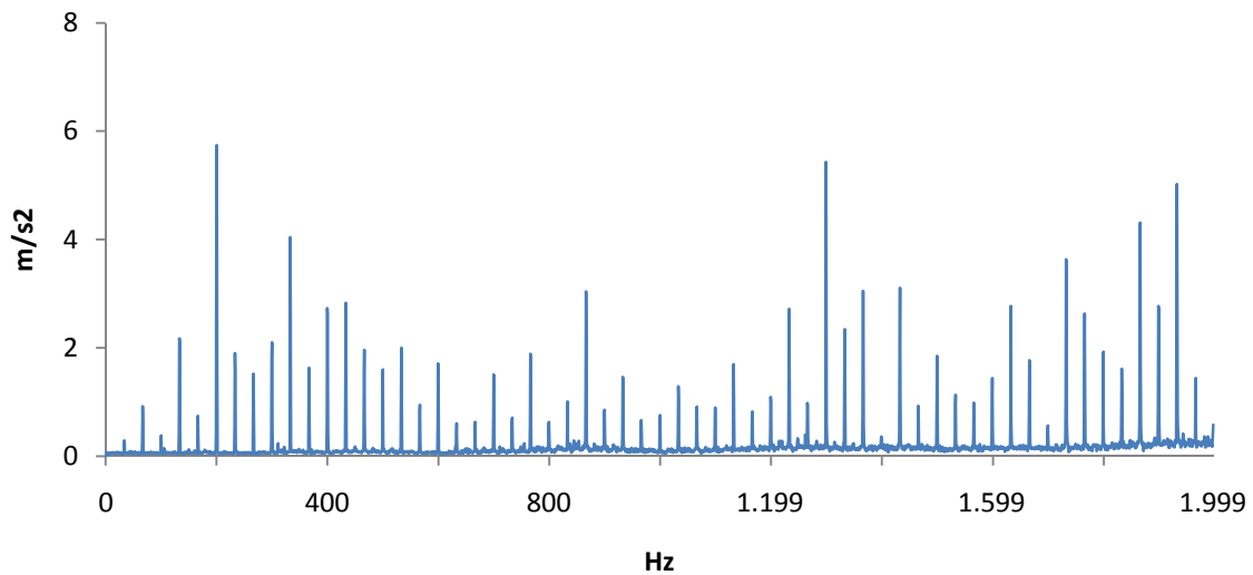
Figura 4.11 – Espectro de aceleração a 4000 rpm, com limite de medição a 2 kHz.
