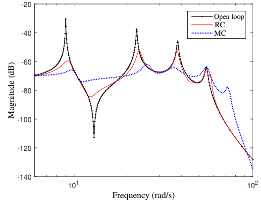
(b) T_{z_2 w} .
