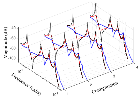
(b) T_{z_2 w} .
