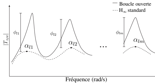
Figure B.4 - Atténuation de T_{z,w} et les amplitudes de crête respectives.
