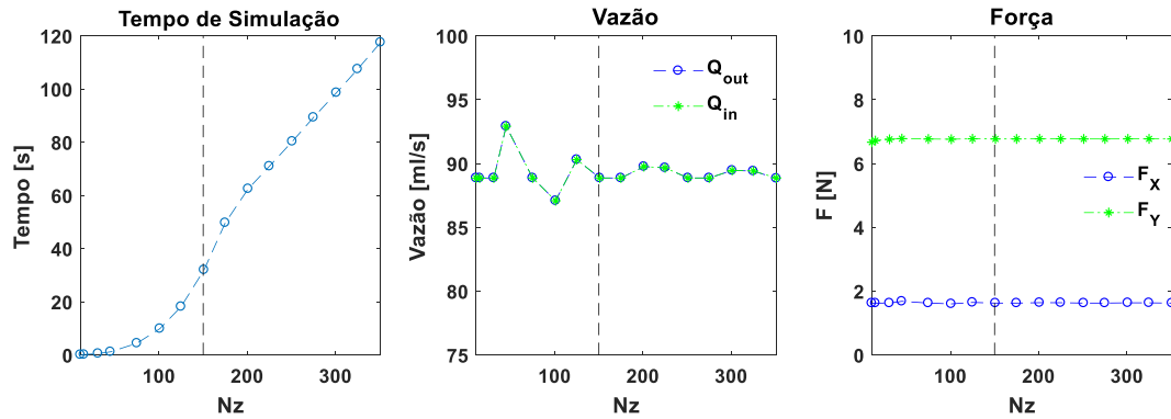
Figura 26: Teste de seleção de malha na direção z.
