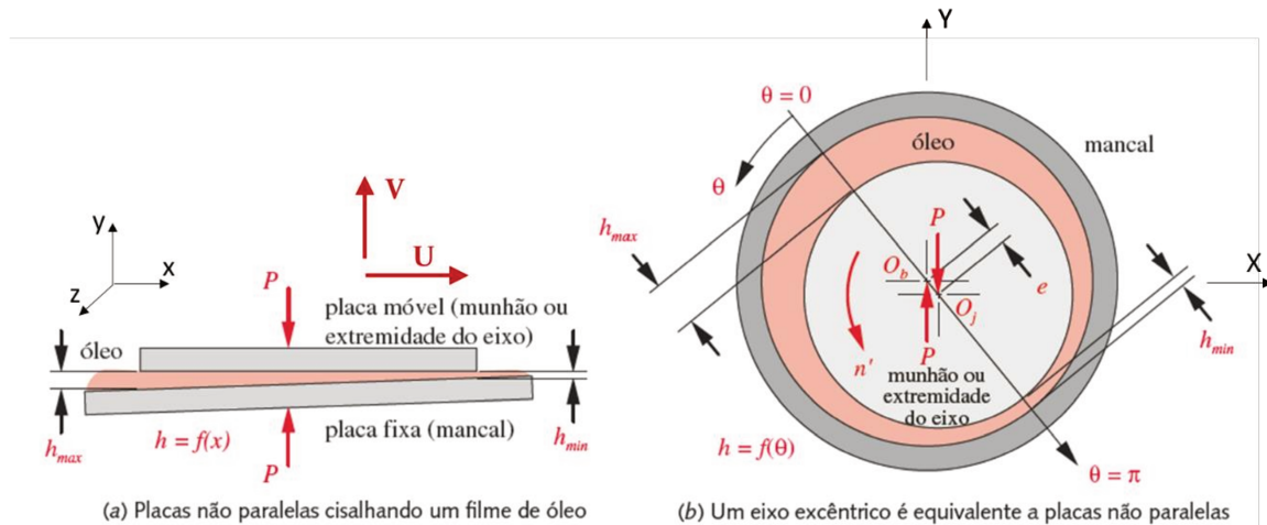
Figura 5: Representação de um mancal hidrodinâmico, mostrando uma hipótese em detalhe (a) e uma visão geral (b). Adaptado de Norton (2013).
