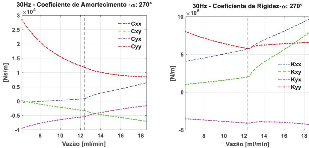
Figura 47: Influência da vazão nos coeficientes equivalentes para o groove em 270°. Valor da vazão de referência em destaque.
