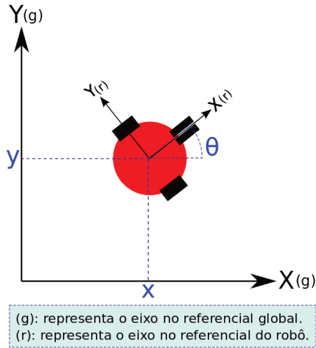
Fig. 1.1: Sistemas de coordenadas e postura do robô
