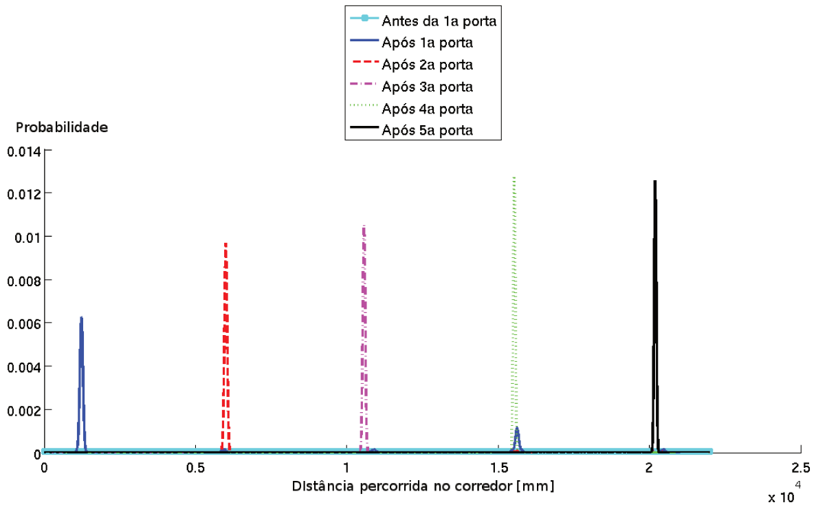
Fig. 4.4: Evolução da crença em ambiente real
