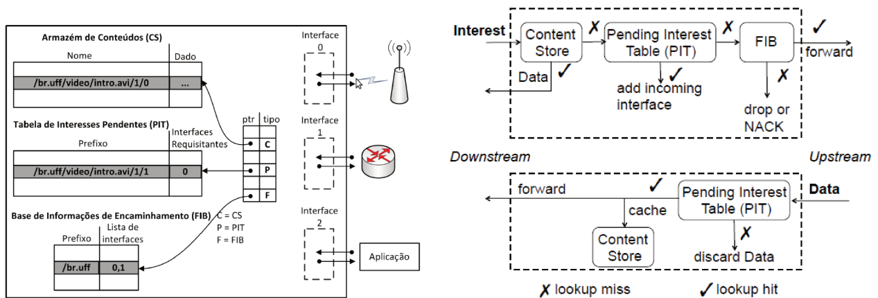
(a) Estruturas de um nó CCN (reproduzido de (de Brito et al. 2012)) (b) Dinâmica do encaminhamento CCN (reproduzido de (Yi et al. 2012))
