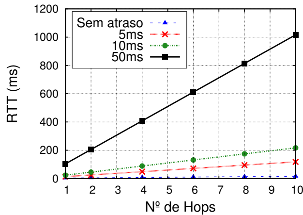
Figura 4.1: RTT vs nº de hops para diferentes valores de atraso de link
