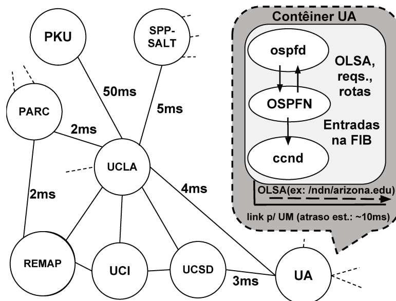
Figura 3.9: Parte do testbed NDN com destaque para o roteamento OSPFN
