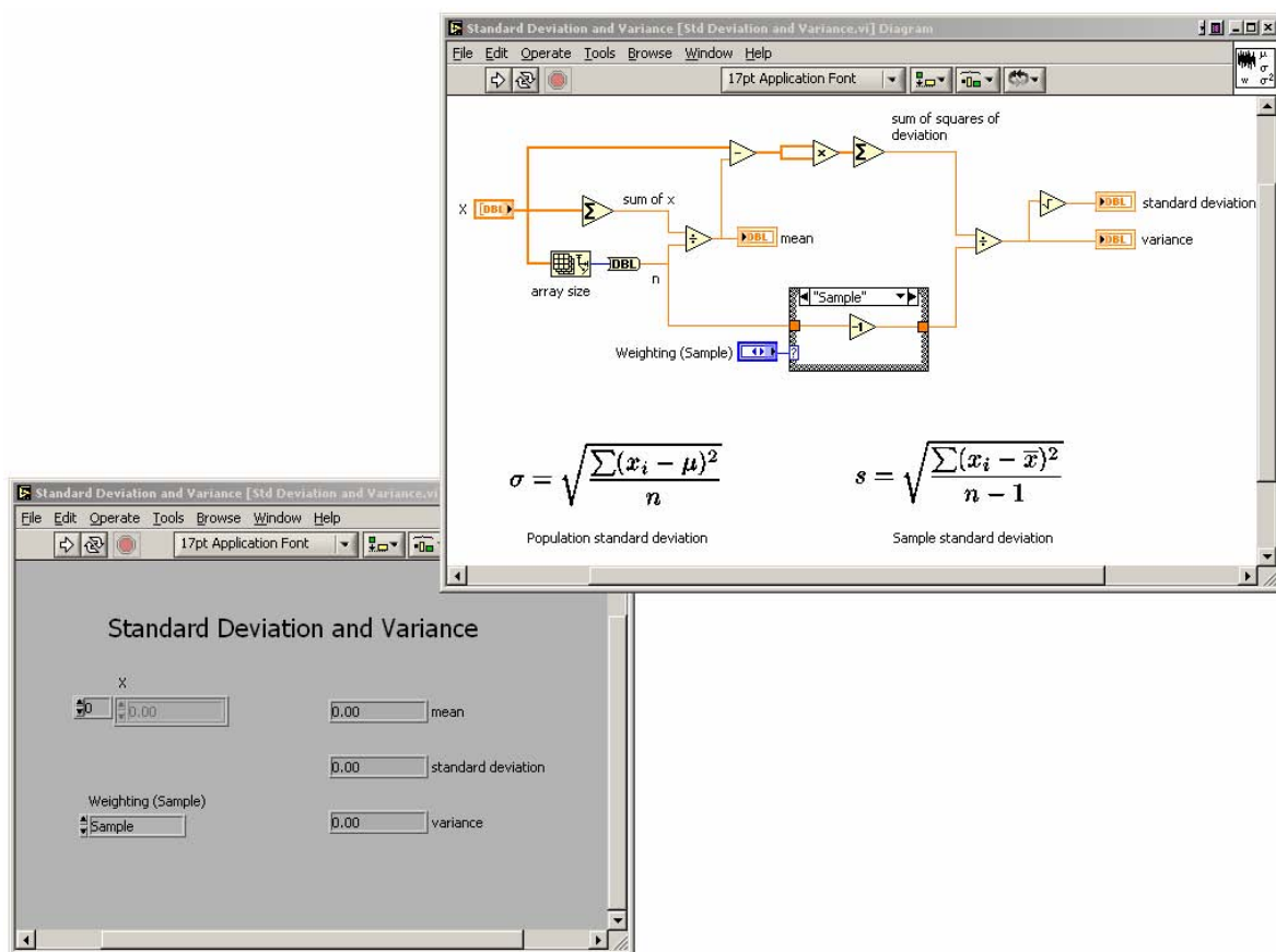
Figura A.5: Tela de um programa simples em LabVIEW que calcula a media e o desvio padrão de um vetor de entrada, mostrando o painel frontal e o diagrama de blocos.
