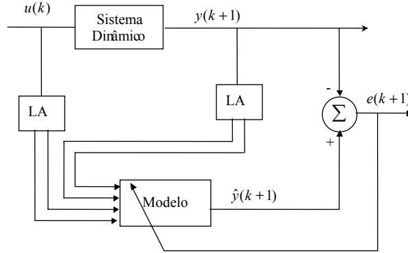
Figura 6.16 – Arquitetura de identificação de sistema não-linear (LA – linhas de atraso)
