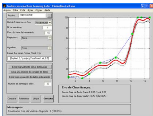
Figura 4.29 – Regressão com kernel do tipo B-spline infinito.
