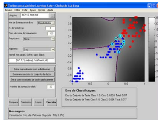
Figura 4.18 – Separação das amostras da espécie Iris virginica das amostras das outras duas espécies, usando SVM com funções de base radial ( \sigma=1,0 ).
