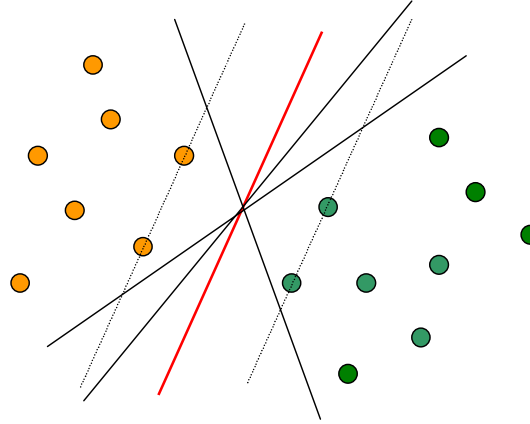
Figura 4.3 – Hiperplano de separação ótimo (em vermelho), com os seus hiperplanos-suporte (tracejados).
