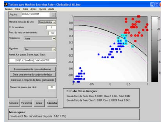
Figura 4.19 – Separação das amostras da espécie Iris virginica das amostras das outras duas espécies, usando SVM com kernel polinomial (grau 2, C = 10 ).
