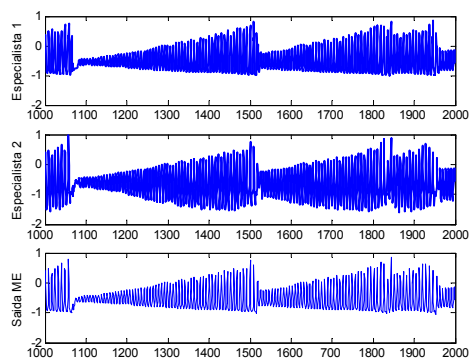
Figura 6.13 – Saída dos especialistas sobre parte do conjunto de teste e saída da mistura.
