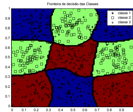
Figura 6.41 – Fronteira de decisão para o conjunto de treinamento
