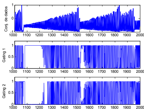
Figura 6.12 – Saída da gating sobre parte do conjunto de teste.
