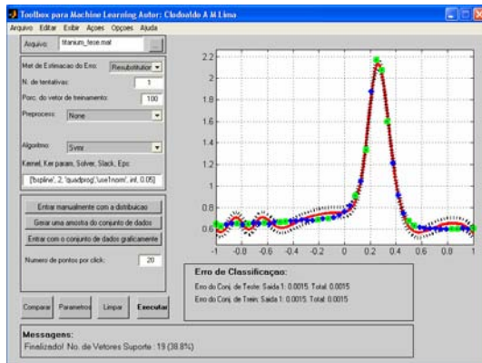
Figura 4.32 – Regressão usando B-spline para Titanium ( \varepsilon = 0,05 , C \rightarrow \infty ).
