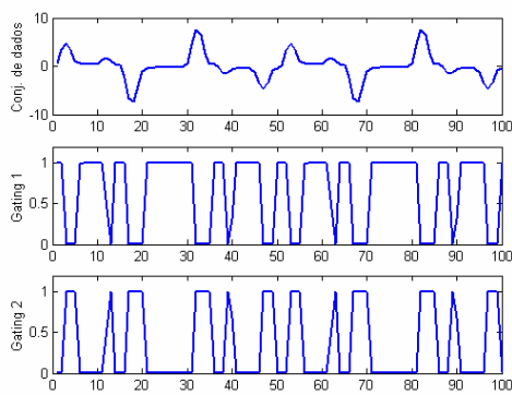
Figura 6.21 – Saída da rede gating de uma ME[SVM].
