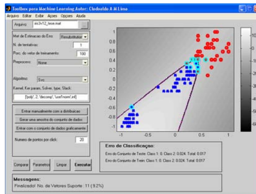
Figura 4.16 – Separação das amostras da espécie Iris virginica das amostras das outras duas espécies, usando SVM com kernel polinomial (grau 2).
