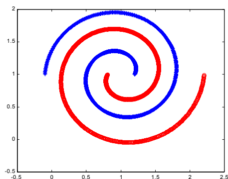
Figura 5.8 – O problema de classificação das duas espirais.
