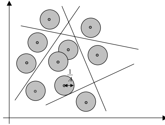
Figura 4.4 – Os candidatos a hiperplano canônico devem manter uma distância mínima de 1/A das amostras.
