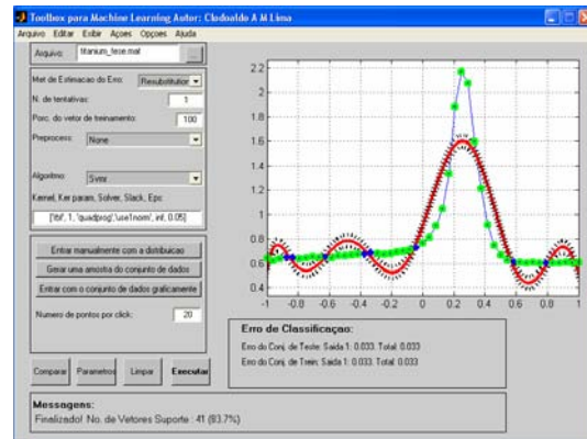
Figura 4.33 – Regressão usando RBF gaussiano para Titanium ( \varepsilon=0,05 , \sigma=1,0 , C \rightarrow \infty ).
