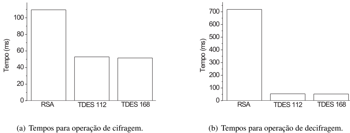
Fig. 4.3: Tempos para cifragem e decifragem empregando RSA e TDES.
