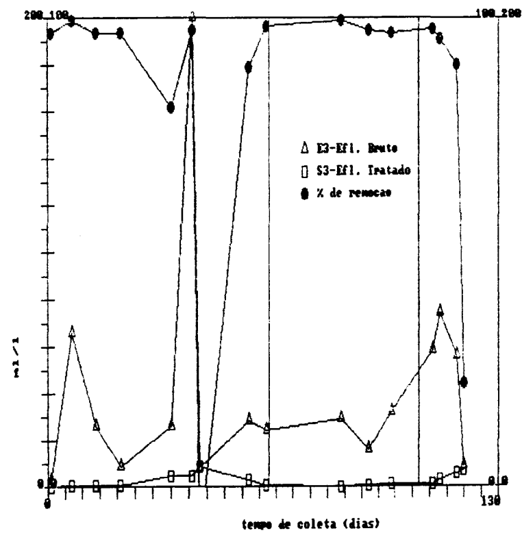
FIGURA 60. Sól. Sedimentáveis: Rampa nº 3 - FASES 2, 3 e 4
