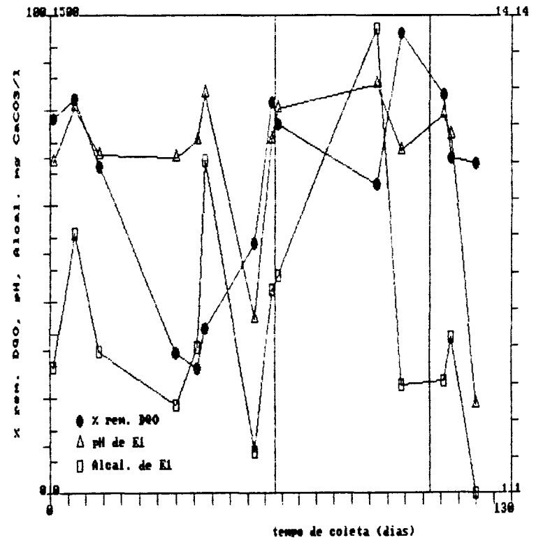
FIGURA 107. Influência dos valores de pH e alcalinidade na Z Rem. de DQO ao longo do tempo na rampa nº 1 nas FASES 2, 3 e 4
