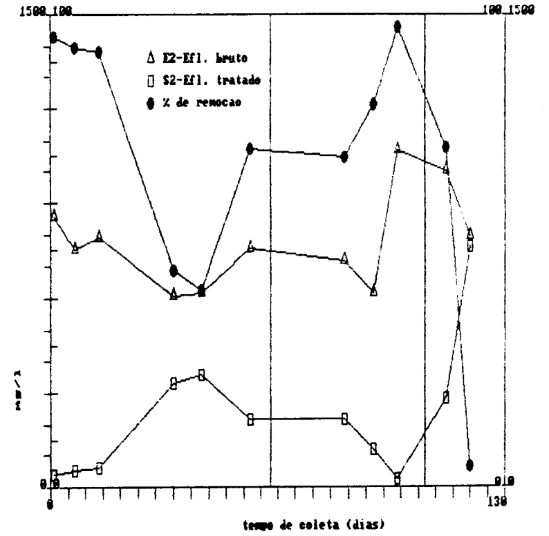
FIGURA 82. Sól. Susp. Totais: Rampa nº 2 - FASES 2, 3 e 4
