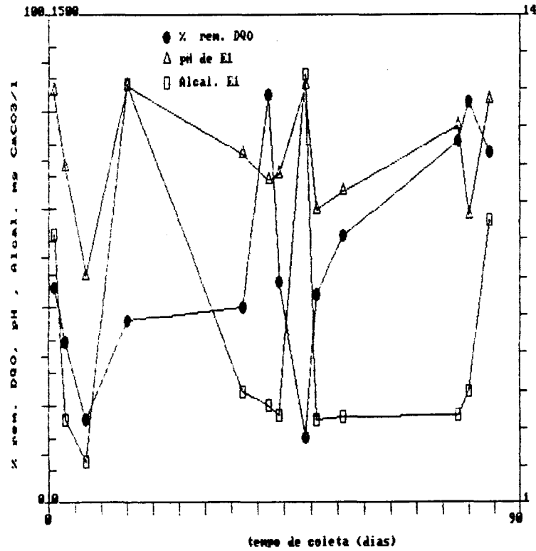
FIGURA 106. Influência dos valores de pH e alcalinidade na Z Rem. de DQO ao longo do tempo na rampa nº 1 na FASE 1
