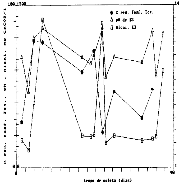
FIGURA 116. Influência dos valores de pH e alcalinidade na % Rem. de Fósforo Total ao longo do tempo na rampa nº 3 na FASE 1
