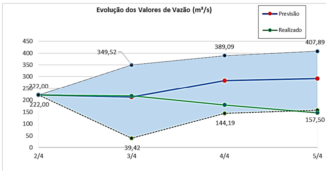
Figura 30 – Gráfico de Envoltórias para Análise do Ponto 2
