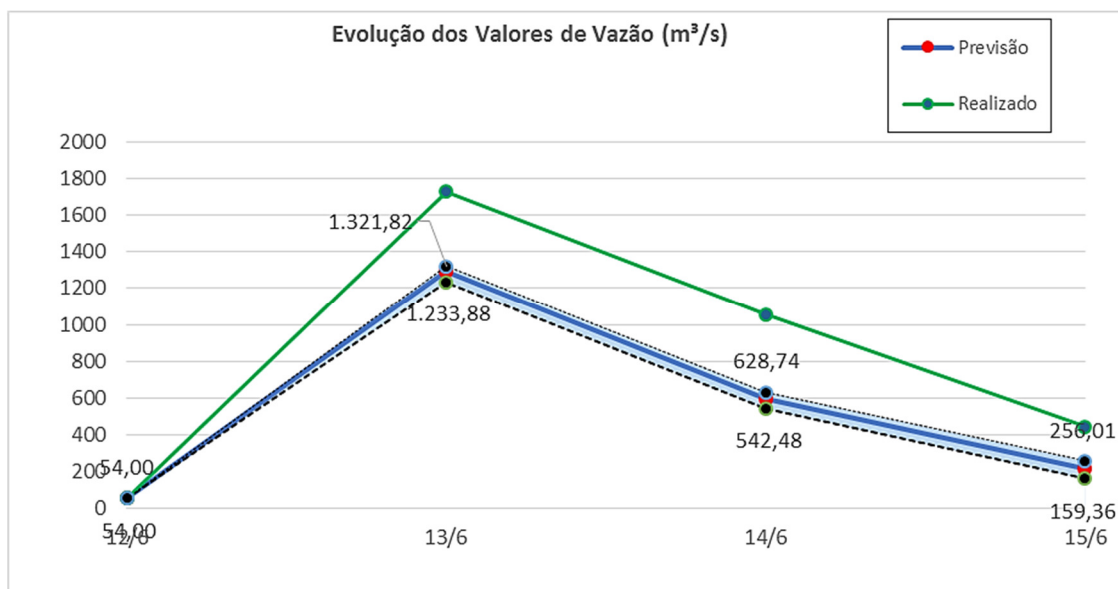
Figura 34 – Gráfico de Envoltórias para Análise do Ponto 6
