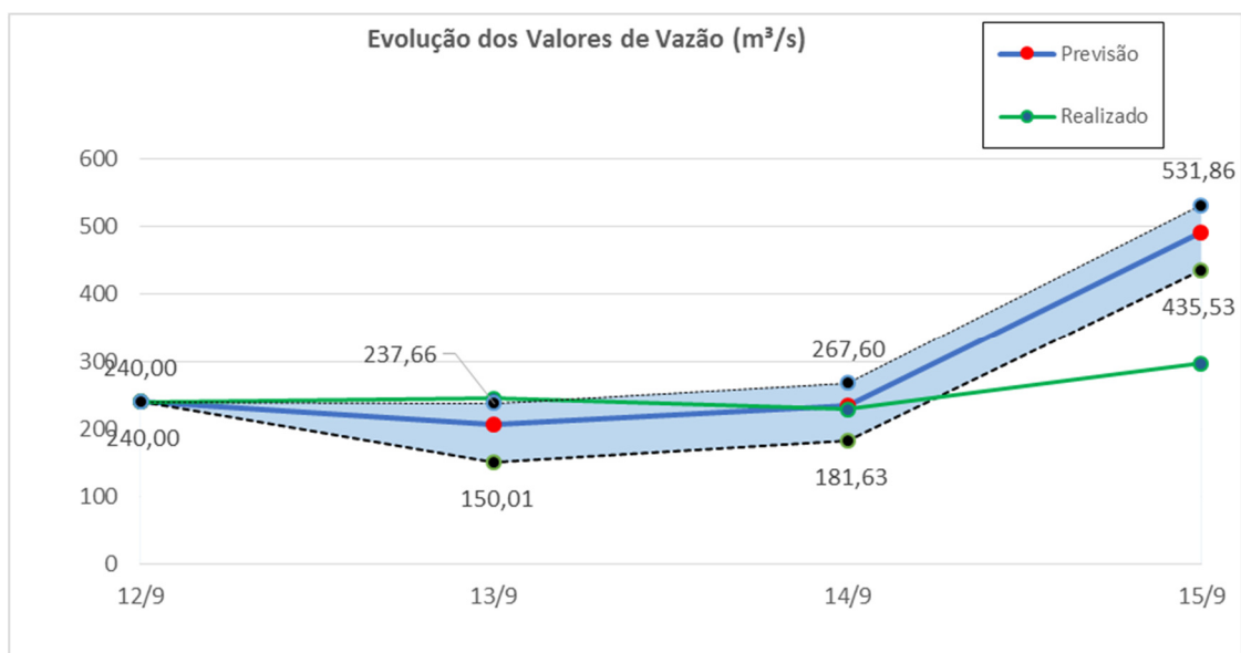
Figura 32 – Gráfico de Envoltórias para Análise do Ponto 4
