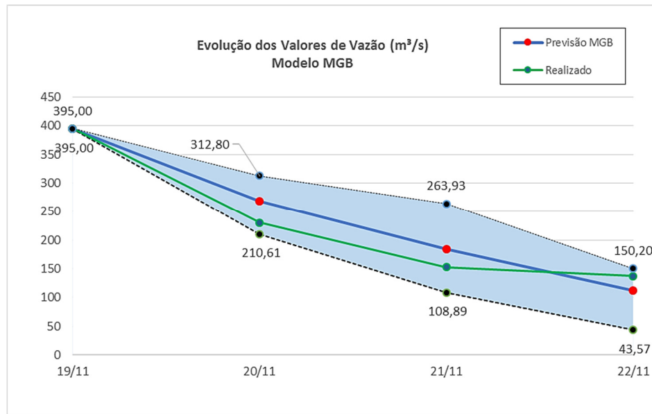
Figura 41 – Gráfico de Envoltórias Modelo MGB para Análise do Ponto 11
