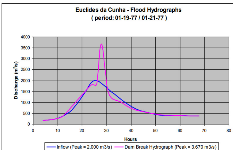
Figura 4 - Hidrograma da ruptura da UHE Euclides da Cunha
