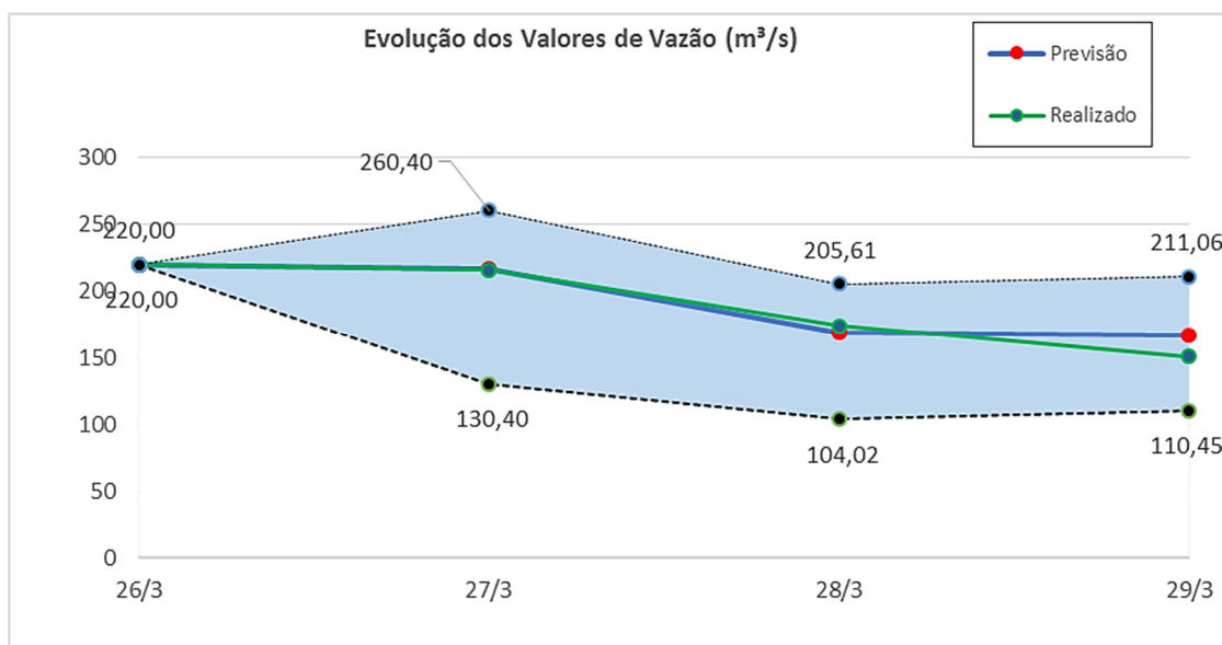
Figura 33 – Gráfico de Envoltórias para Análise do Ponto 5
