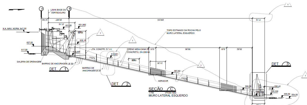
Figura 9 - Seção típica do vertedouro da UHE Barra Grande
