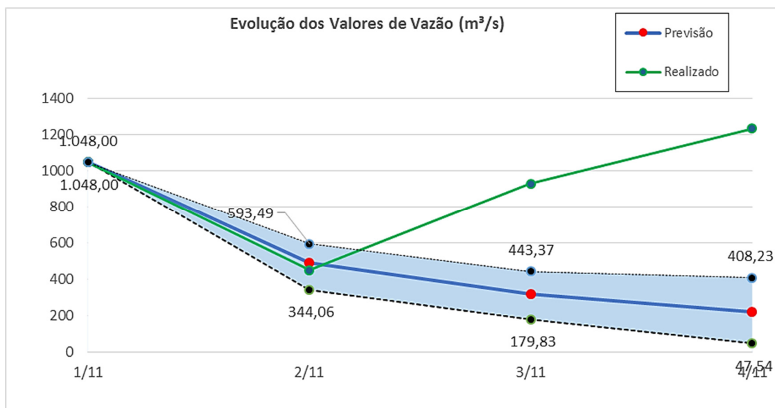
Figura 36 – Gráfico de Envoltórias para Análise do Ponto 8
