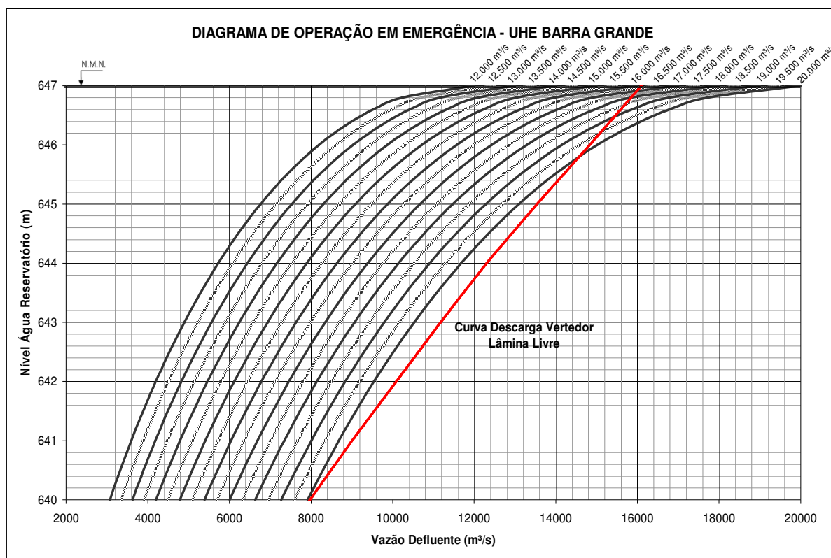
Figura 2 - Diagrama de operação do Vertedouro em Emergência - Exemplo da Usina de Barra Grande, rio Pelotas-RS
