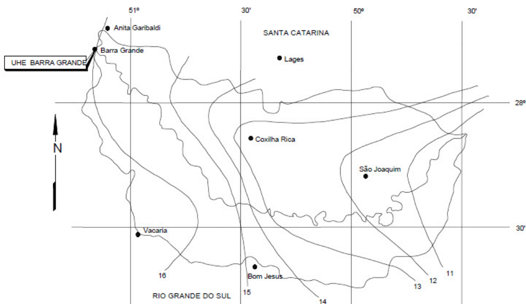
Figura 18 – Isotermas Anuais Médias na Bacia do Rio Pelotas a Montante da UHE Barra Grande
