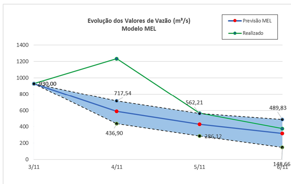
Figura 38 - Gráfico de Envoltórias Modelo MEL para Análise do Ponto 9
