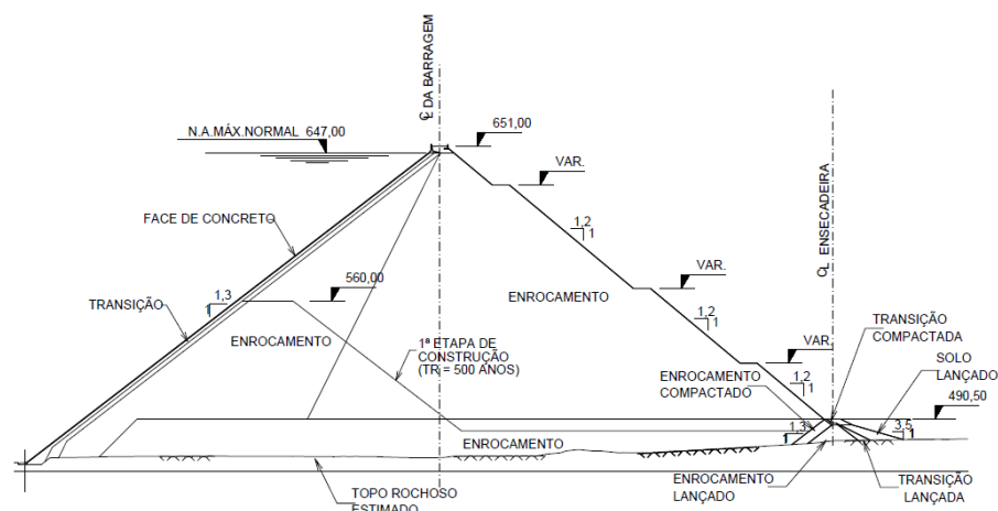
Figura 15 – Seção Transversal da Barragem
