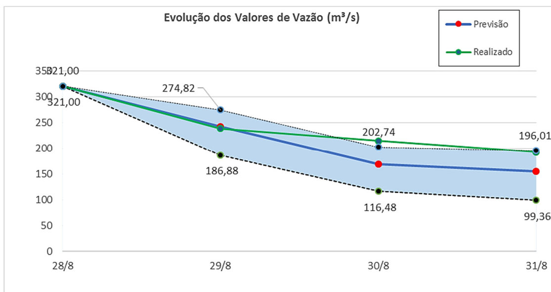
Figura 31 – Gráfico de Envoltórias para Análise do Ponto 3
