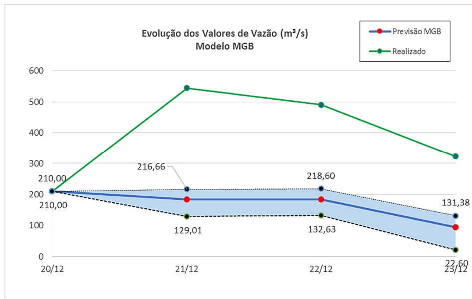
Figura 43 – Gráfico de Envoltórias Modelo MGB para Análise do Ponto 12
