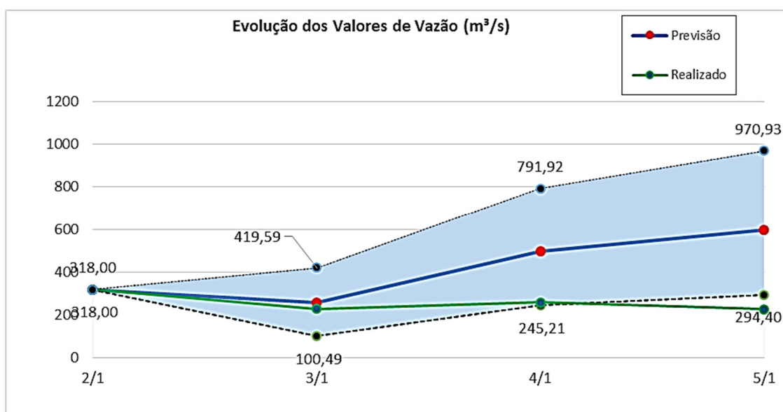
Figura 29 – Gráfico de Envoltórias para Análise do Ponto 1
