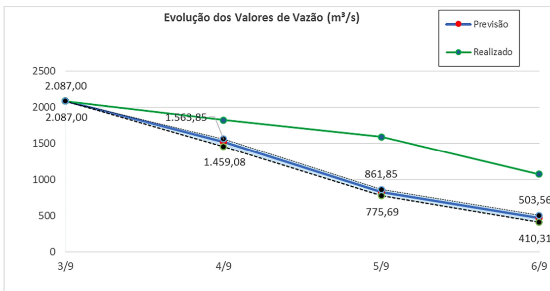
Figura 35 – Gráfico de Envoltórias para Análise do Ponto 7
