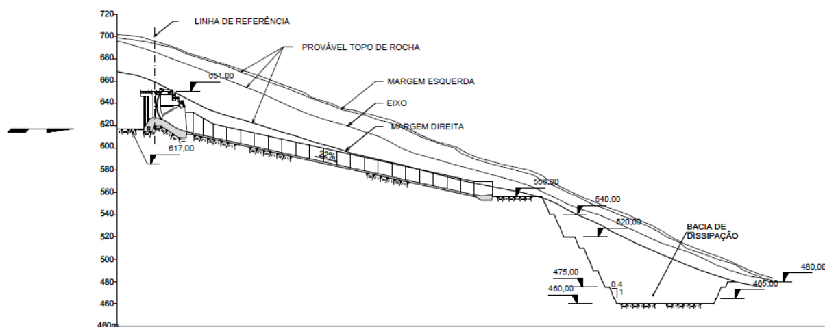
Figura 17 – Seção Transversal do Vertedouro
