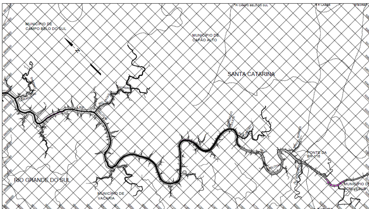
Figura 13 – Planta do Reservatório (2/2)
