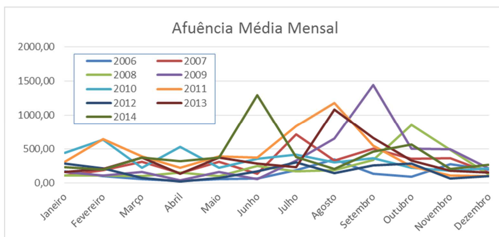
Figura 20 - Afluência Média Mensal da Região da usina de Barra Grande
