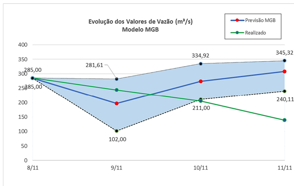
Figura 39 – Gráfico de Envoltórias Modelo MGB para Análise do Ponto 10
