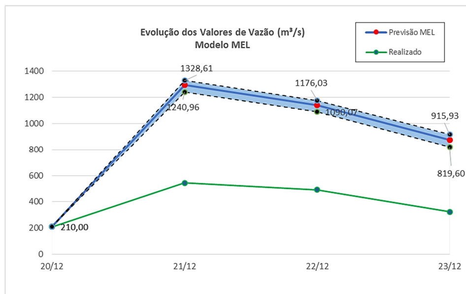
Figura 44 - Gráfico de Envoltórias Modelo MEL para Análise do Ponto 12
