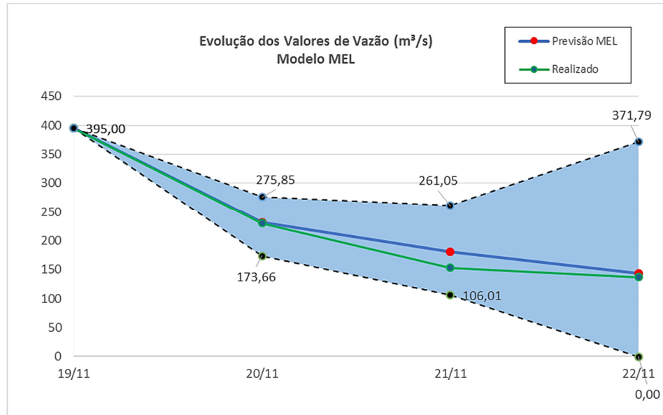
Figura 42 - Gráfico de Envoltórias Modelo MEL para Análise do Ponto 11
