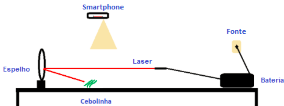
Figura 1. Configuração experimental para avaliação através do Biospeckle.
