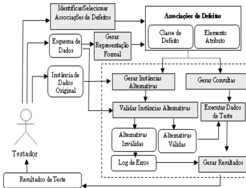
Figura 6.1: Ilustração das funcionalidades da XTool
