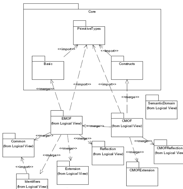
Figura 2.7: Pacotes de MOF 2.0
