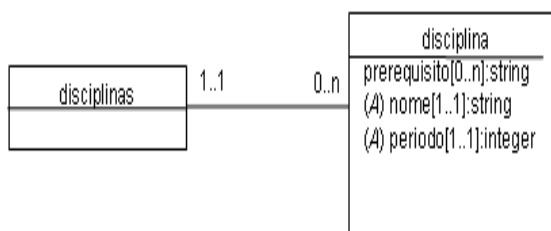
Figura 5.2: Modelo de dados do XML Schema “disciplinas.xsd”
