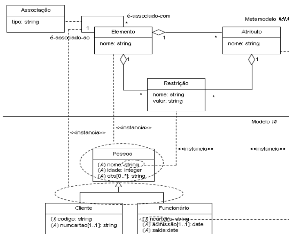
Figura 4.4: Modelo de dados M descrito pelo Metamodelo MM
