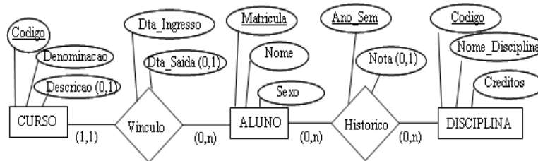
Figura 5.3: Diagrama Entidade-Relacionamento
