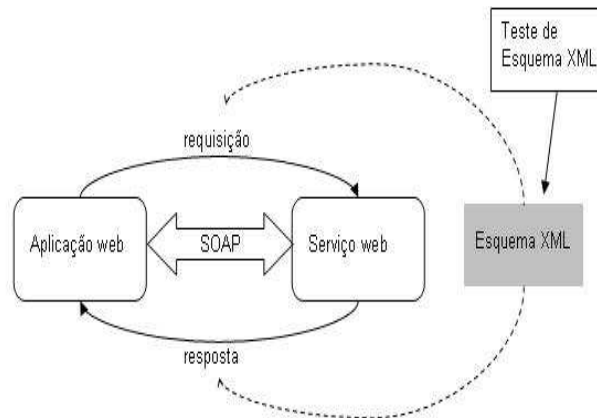
Figura 5.1: Contexto de teste de esquema XML no teste de serviços Web
