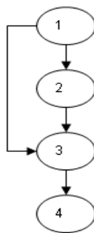
Figura 2.8: Exemplo de grafo de fluxo de controle de um programa P
