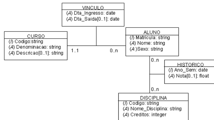
Figura 5.4: Modelo de dados para o esquema representado pelo DER da Figura 5.3
