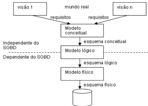
Figura 2.1: Níveis da abordagem top-down no projeto de uma base de dados
