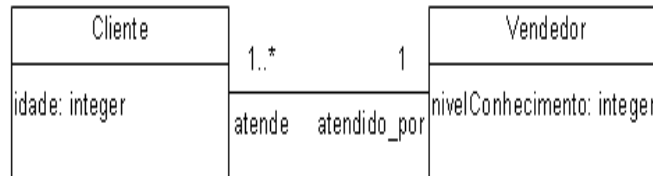
Figura A.1: Diagrama de classes usado para exemplificar invariantes
