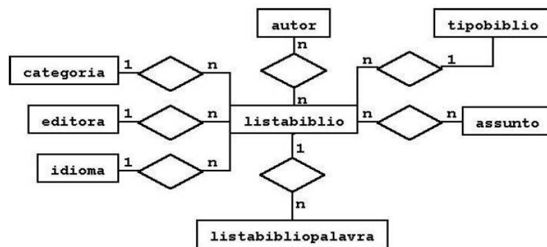
Figura E.2: Diagrama de Entidade-Relacionamento da biblioteca - Estudo de Caso IV
