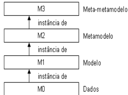
Figura 2.4: Arquitetura de Metamodelagem
