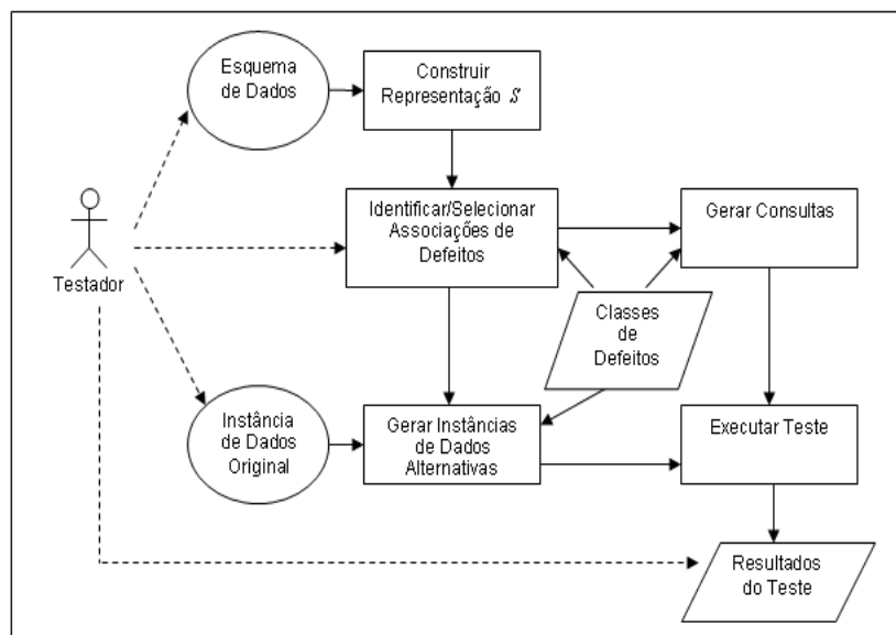
Figura 4.1: Processo de teste definido na AIDA
