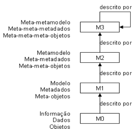
Figura 2.5: Arquitetura de MOF
