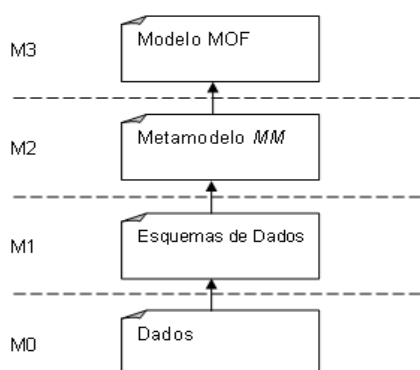
Figura 4.2: Metamodelo MM no modelo MOF
