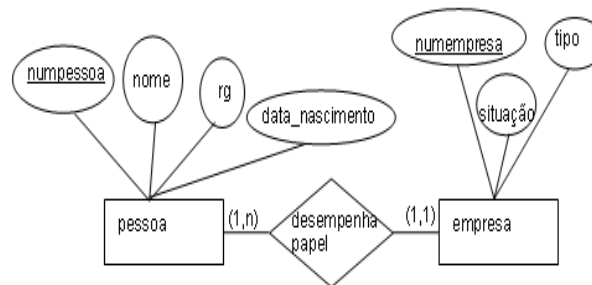
Figura 2.2: Exemplo de DER
