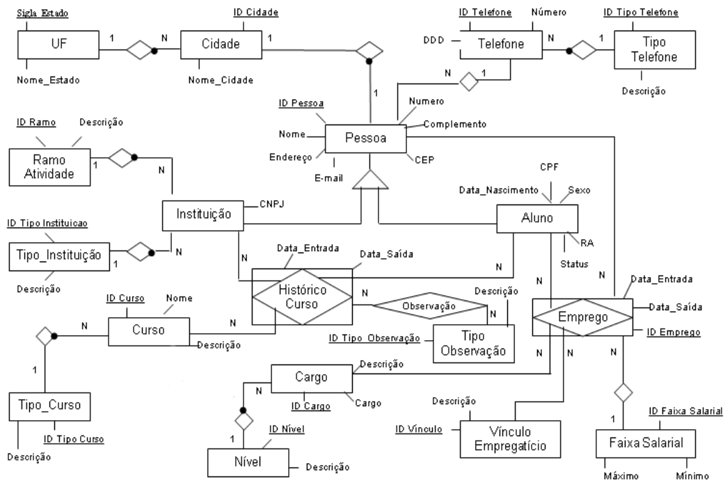
Figura D.1: Diagrama de Entidade-Relacionamento da base de dados relacional - Estudo de Caso III
