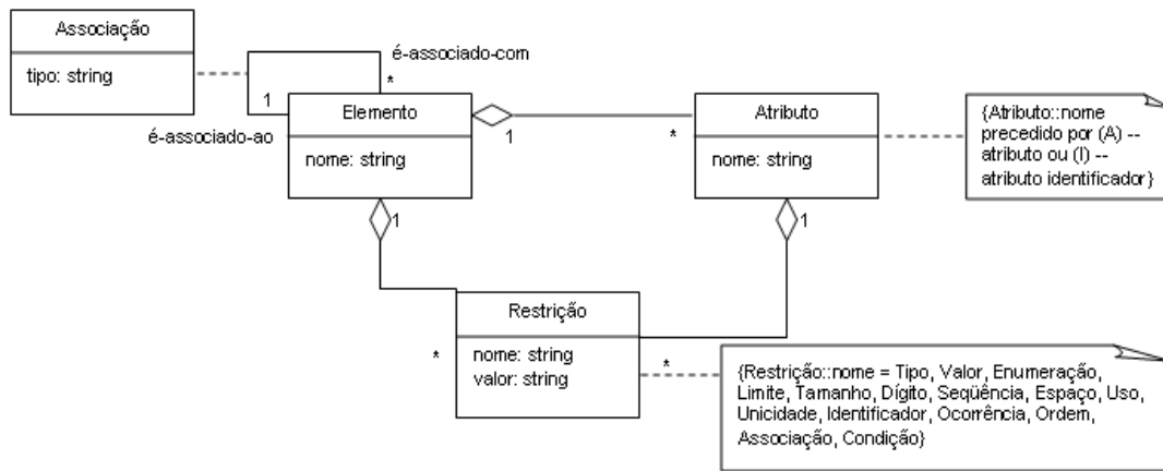
Figura 4.3: Metamodelo MM
