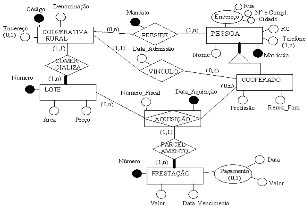
Figura E.1: Diagrama de Entidade-Relacionamento da cooperativa rural - Estudo de Caso IV
