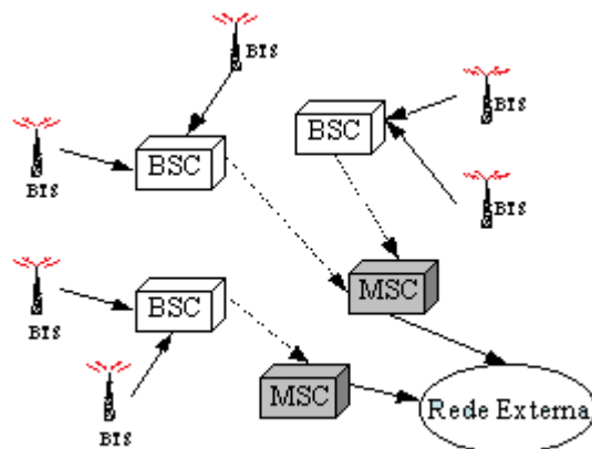
FIGURA 2.4: EXEMPLO DE UMA REDE TELEFONIA MÓVEL CELULAR (GSM).
