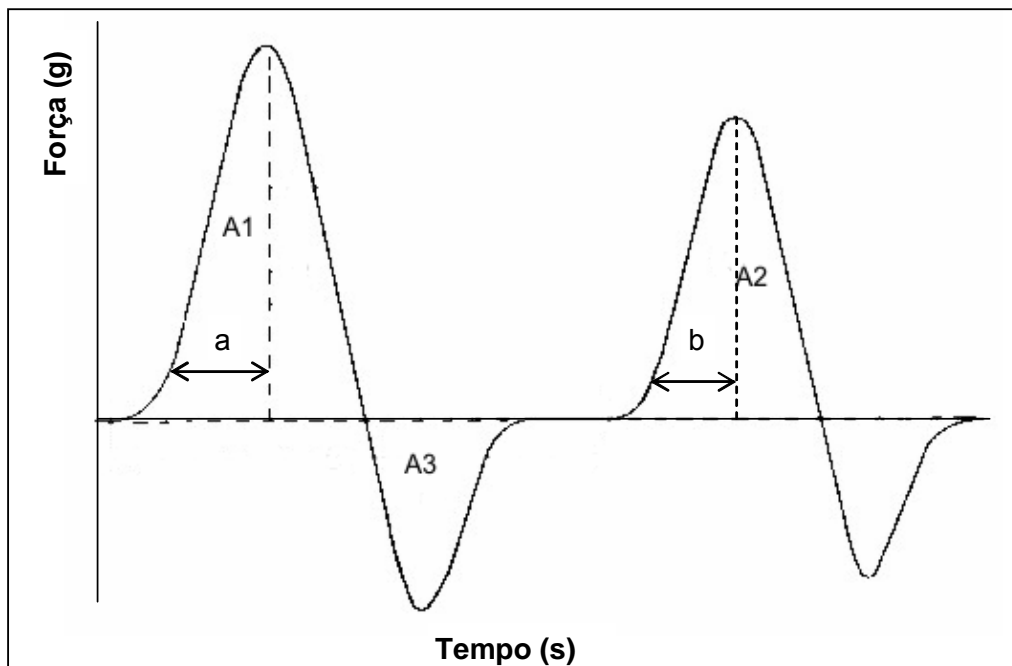
Figura 6. Curva típica de um perfil de textura instrumental.
