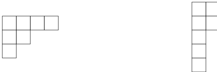
Figura 1 – Diagramas de Young de [\lambda] , a esquerda, e [\mu] , a direita.
