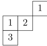
Figura 16 – T_{(3^2,2,1) \setminus (3,2)} .
