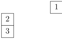
Figura 19 – T_{(5,1^2) \setminus (4)}
