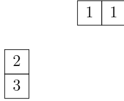
Figura 10 – T_{(5,2,1^2) \setminus (3,2)} .
