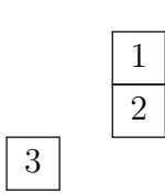
Figura 21 – T_{(3^2,1) \setminus (2^2)}
