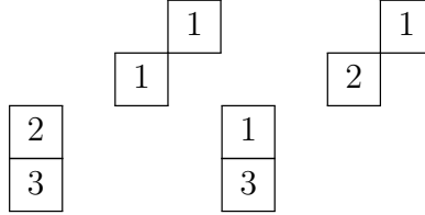
Figura 13 – T_{(4,3,1^2) \setminus (3,2)} .
