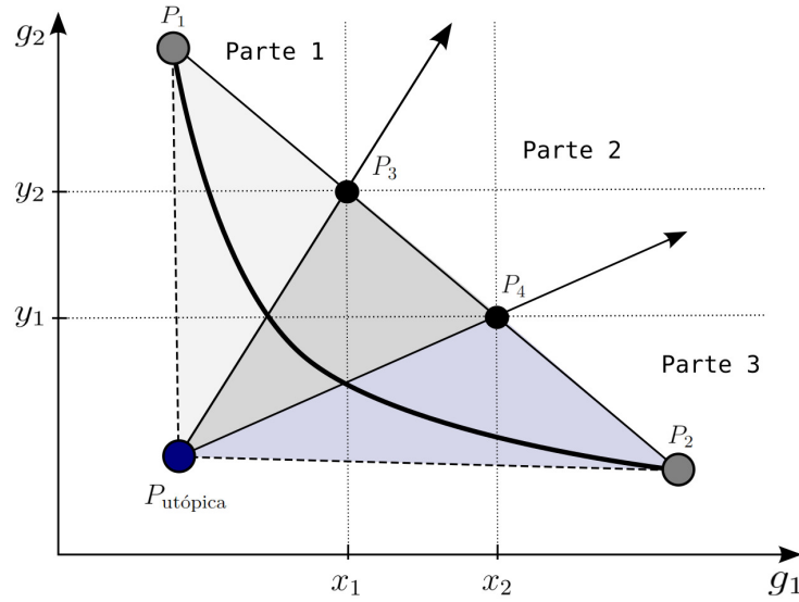
Figura 26 – Divisão da fronteira não-dominada em três partes. As soluções em cinza representam os extremos da fronteira, P_1 = (\min(g_1), \max(g_2)) e P_2 = (\max(g_1), \min(g_2)) . A solução em azul representa a solução utópica, P_{\text{utópica}} = (\min(g_1), \min(g_2)) .
