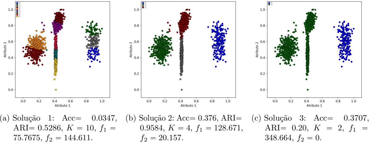
Figura 33 – Indivíduos não dominados de f_1 = \text{Compactação} e f_2 = \text{Conectividade} do conjunto 2d-4c-no6.
