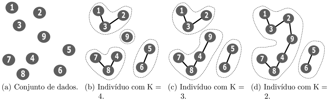
Figura 23 – Exemplo de inicialização de indivíduos pelo Algoritmo de Kruskal , com [K_{min}, K_{max}] = [2, 4] .
