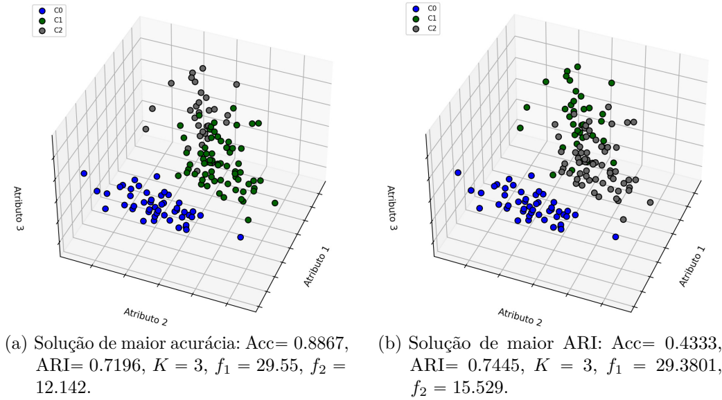
Figura 36 – Soluções de maior acurácia e ARI de f_1 = \text{Compactação} e f_2 = \text{Conectividade} .
