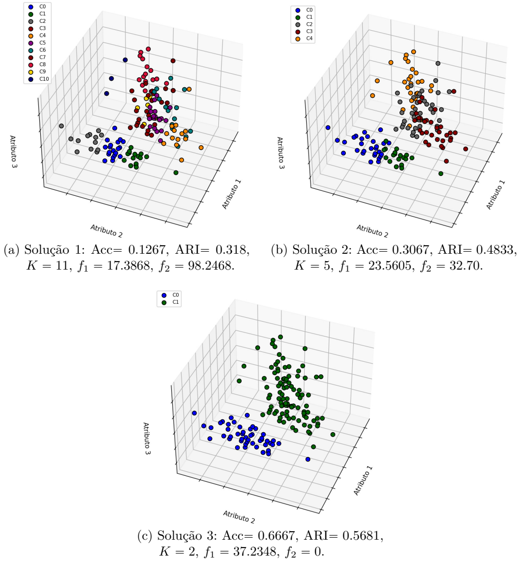
Figura 35 – Indivíduos não dominados de f_1 = \text{Compactação} e f_2 = \text{Conectividade} do conjunto Iris .
