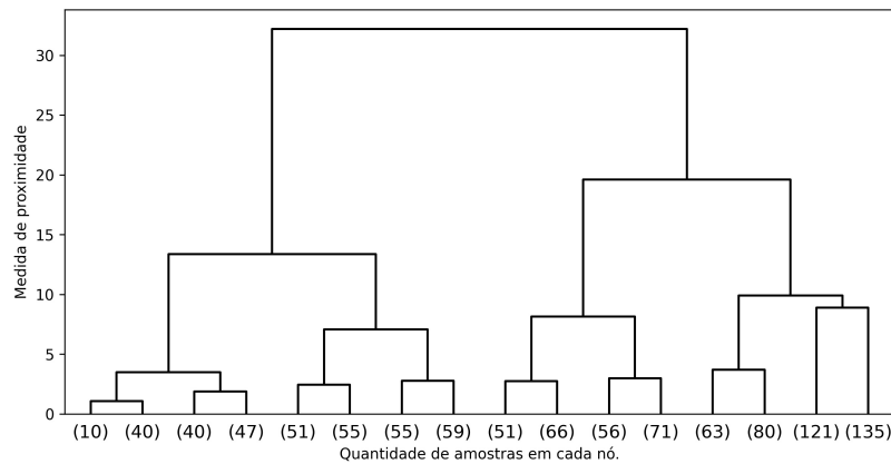
Figura 6 – Dendrograma do conjunto de dados Moons , gerado a partir da biblioteca Scipy e Scikit-learn .
