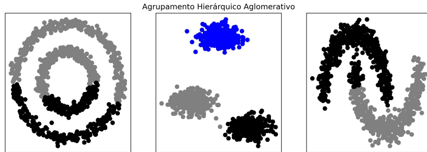
Figura 5 – Resultado do algoritmo de agrupamento hierárquico aglomerativo com ligação Average-link gerado respectivamente para as bases Circles , Blobs e Moons .
