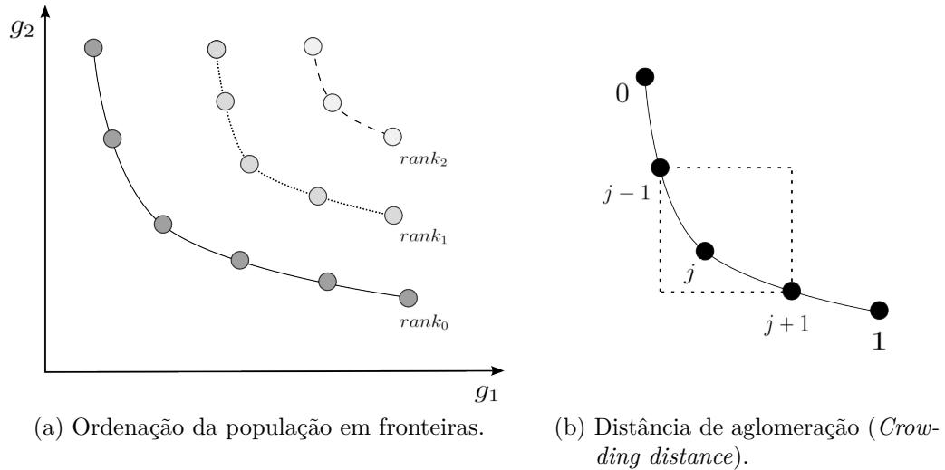
Figura 13 – Classificação não-dominada e distância de aglomeração utilizada no NSGA-II.
