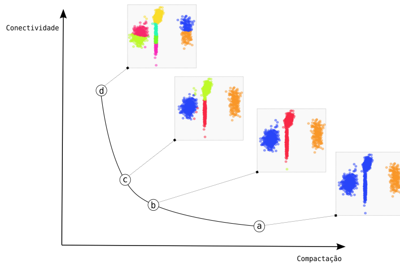
Figura 22 – Representação da fronteira com as soluções não-dominadas, destacando diferentes formas de agrupar os dados. Solução a ( K=2 ), b ( K=4 ), c ( K=4 ) e d ( K=8 ).
