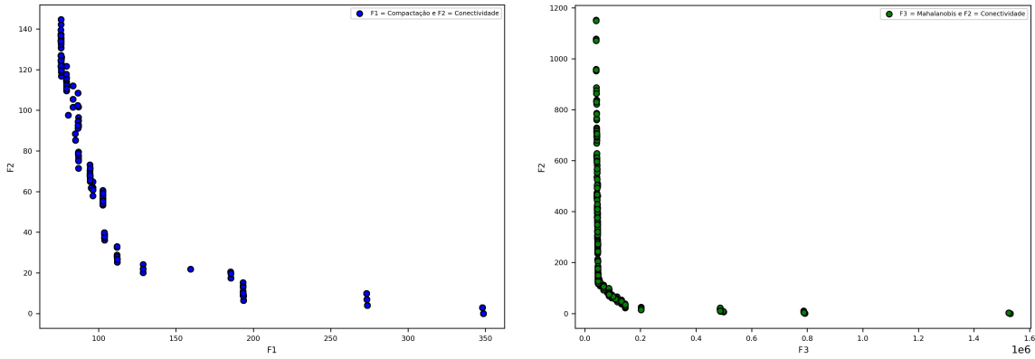
(a) f_1 = Compactação e f_2 = Conectividade.
