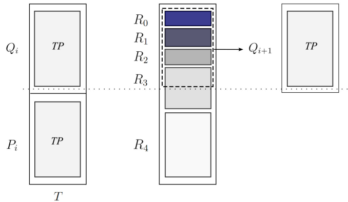
Figura 14 – Processo de seleção da próxima geração no NSGA-II.
