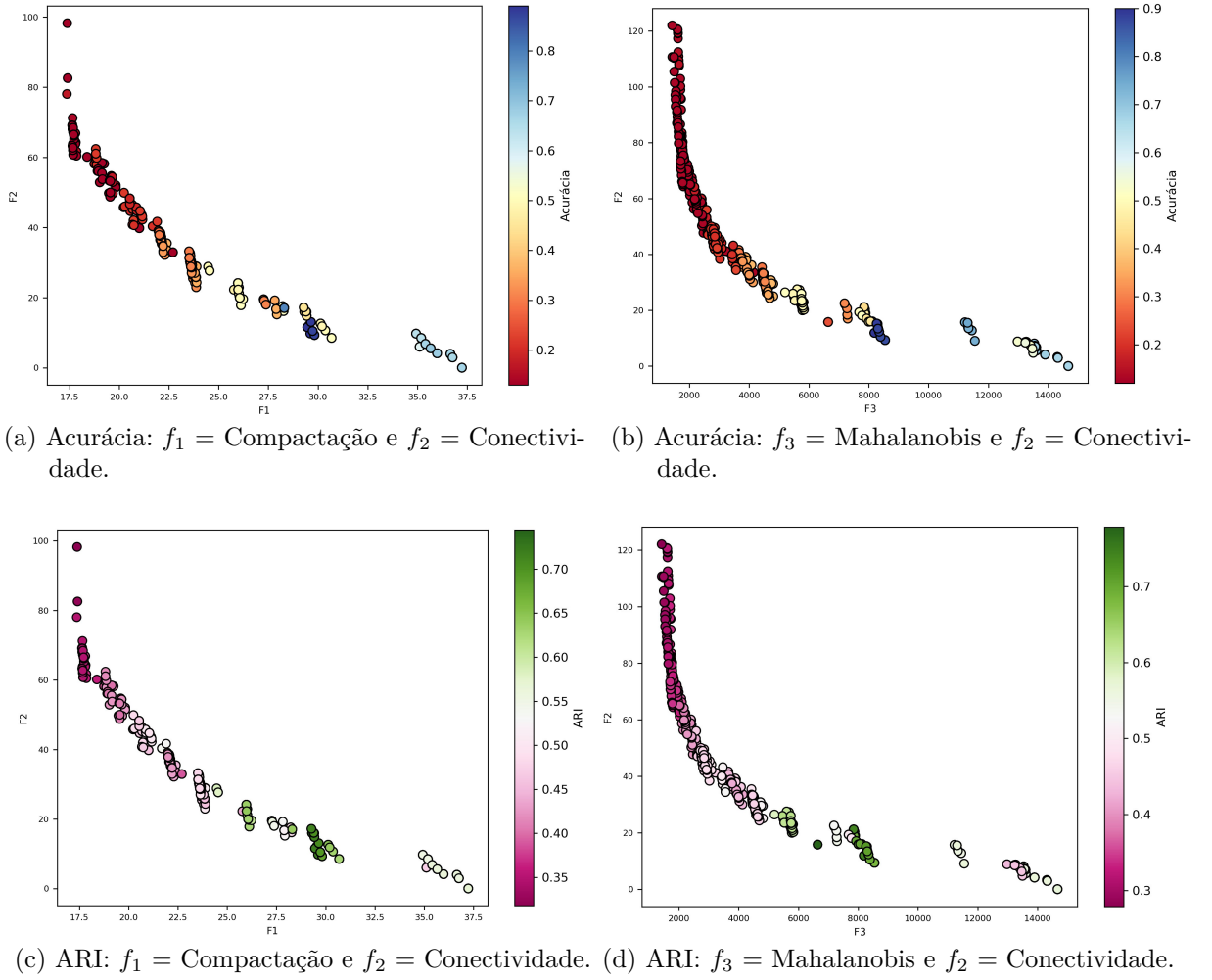
Figura 32 – Acurácia e ARI das soluções não-dominadas de 5 rodadas do conjunto Iris .
