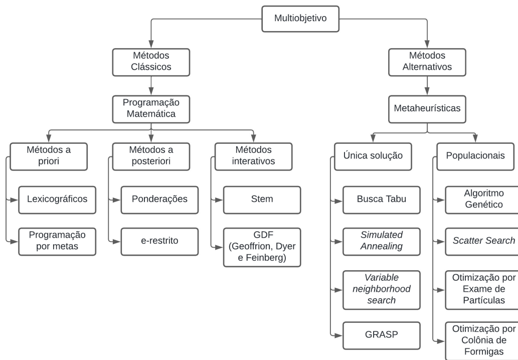
Figura 12 – Categorização dos métodos de resolução para multiobjetivo.
