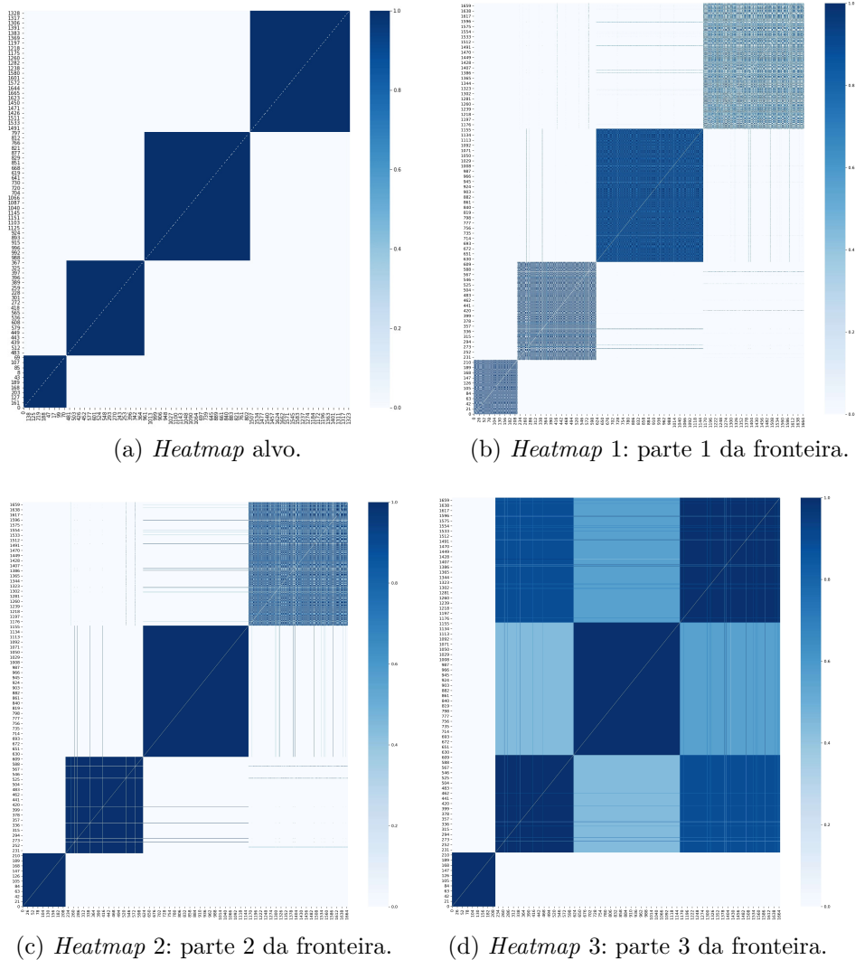
Figura 37 – Heatmaps 2d-4c-no6.
