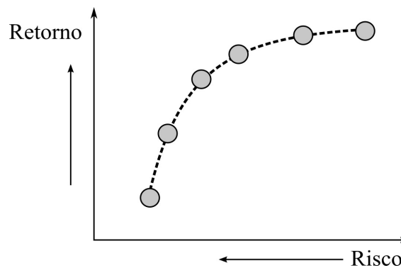
Figura 8 – Exemplo de um problema de seleção de portfólios.
