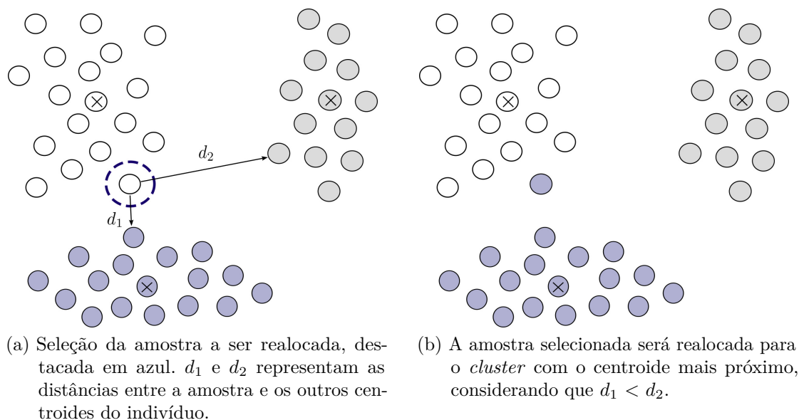
Figura 24 – Exemplo de mutação centroide.
