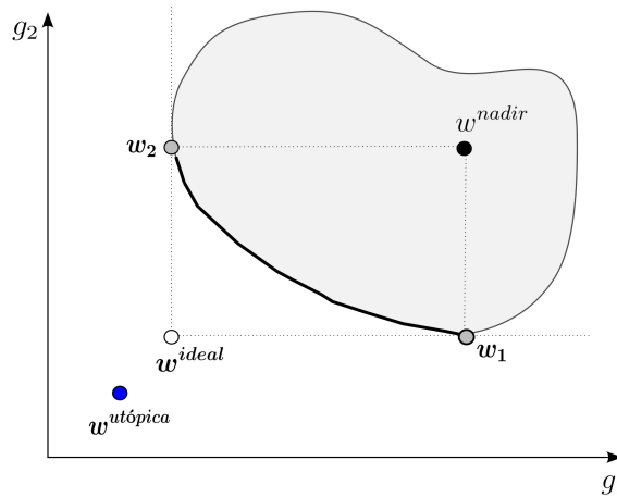
Figura 11 – Soluções especiais de um problema multiobjetivo.
