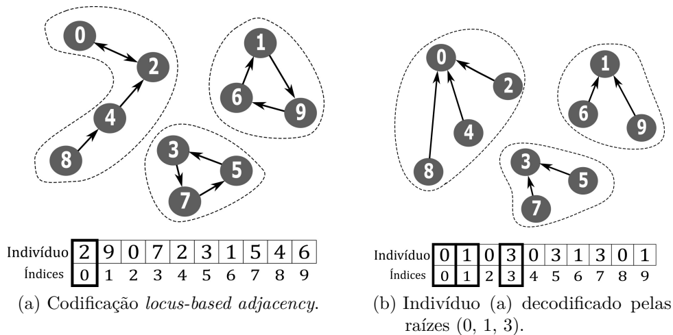
Figura 21 – Exemplo da codificação e decodificação utilizada no algoritmo.
