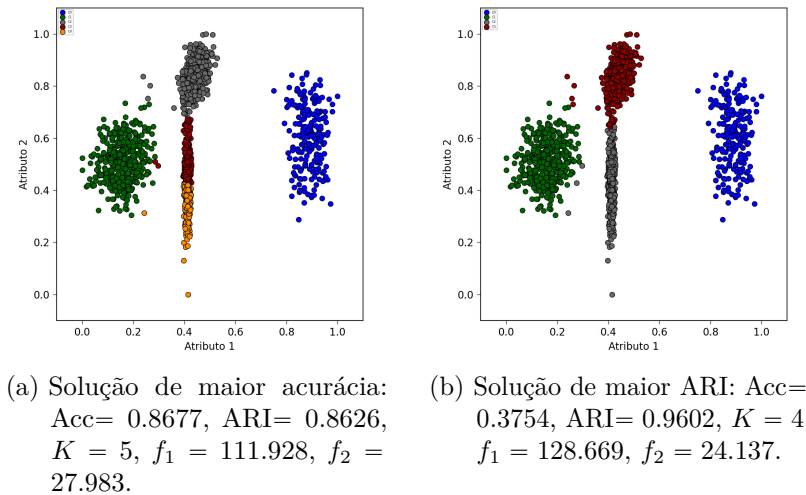
Figura 34 – Soluções de maior acurácia e ARI de f_1 = \text{Compactação} e f_2 = \text{Conectividade} .
