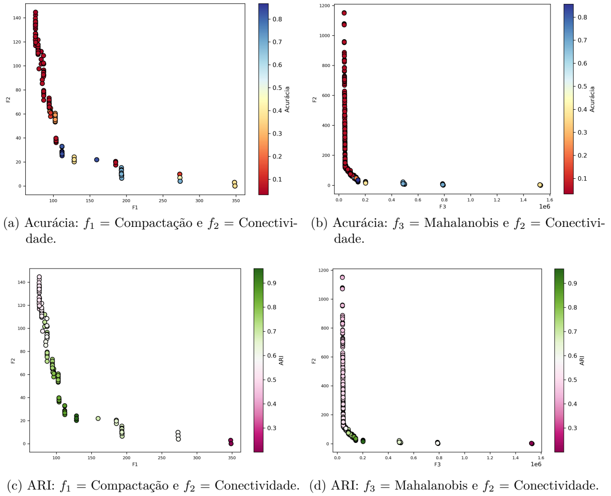
Figura 31 – Acurácia e ARI das soluções não-dominadas de 5 rodadas do conjunto 2d-4c-no6.
