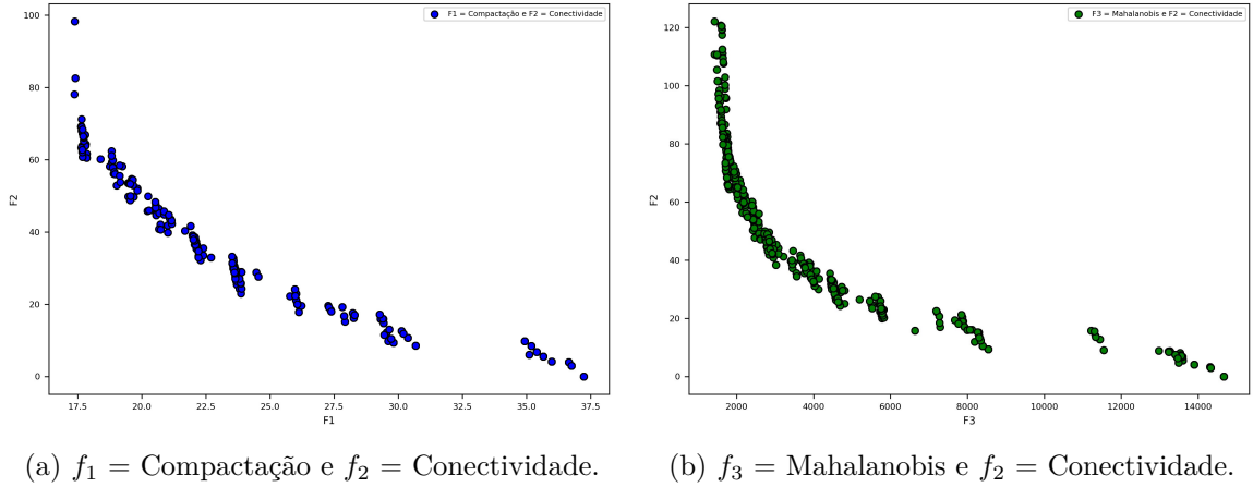
Figura 30 – Variações das funções-objetivo conjunto Iris .
