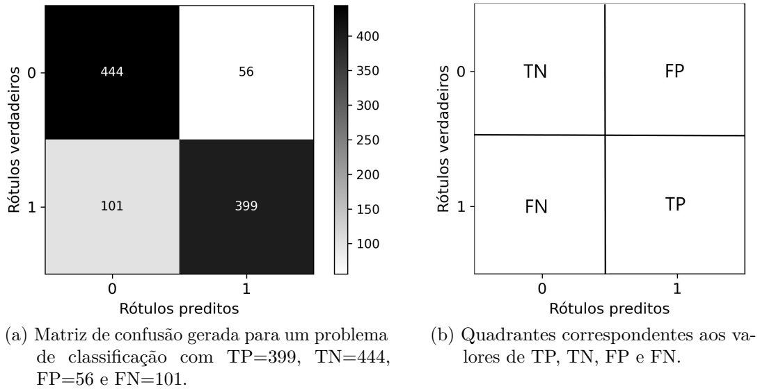
Figura 7 – Matriz de confusão.
