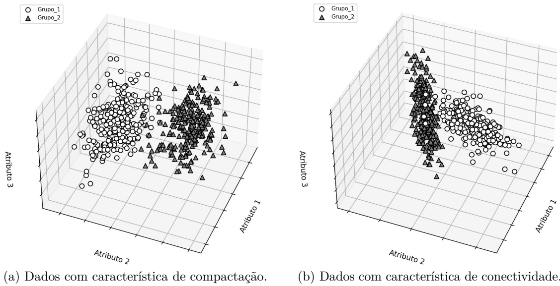
Figura 18 – Diferentes distribuições de dados.
