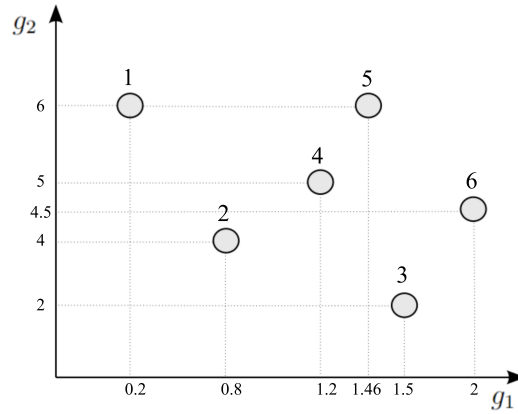
Figura 10 – Conceito de dominância em um problema multiobjetivo.
