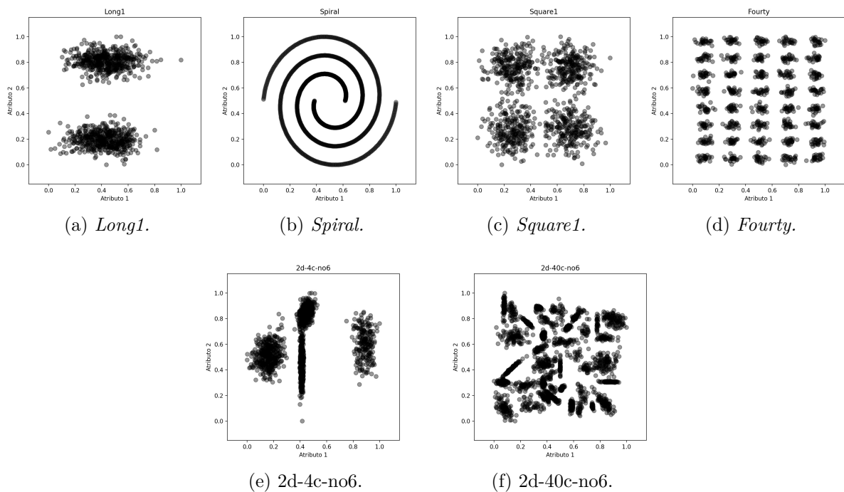
Figura 28 – Conjuntos de dados sintéticos.
