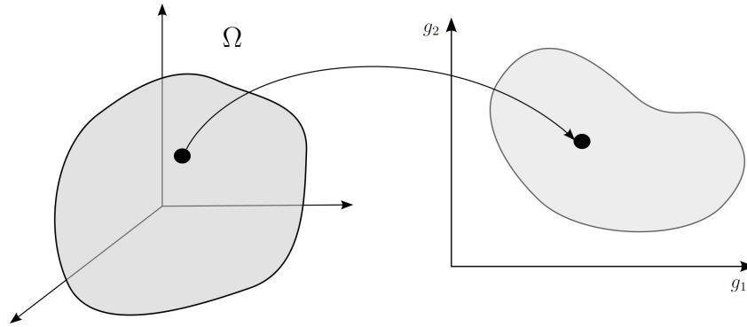
Figura 9 – Espaço das variáveis de decisão e espaço dos objetivos.
