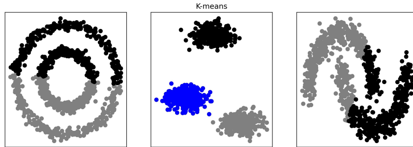
Figura 4 – Resultado do algoritmo K-means gerado respectivamente para as bases Circles , Blobs e Moons .
